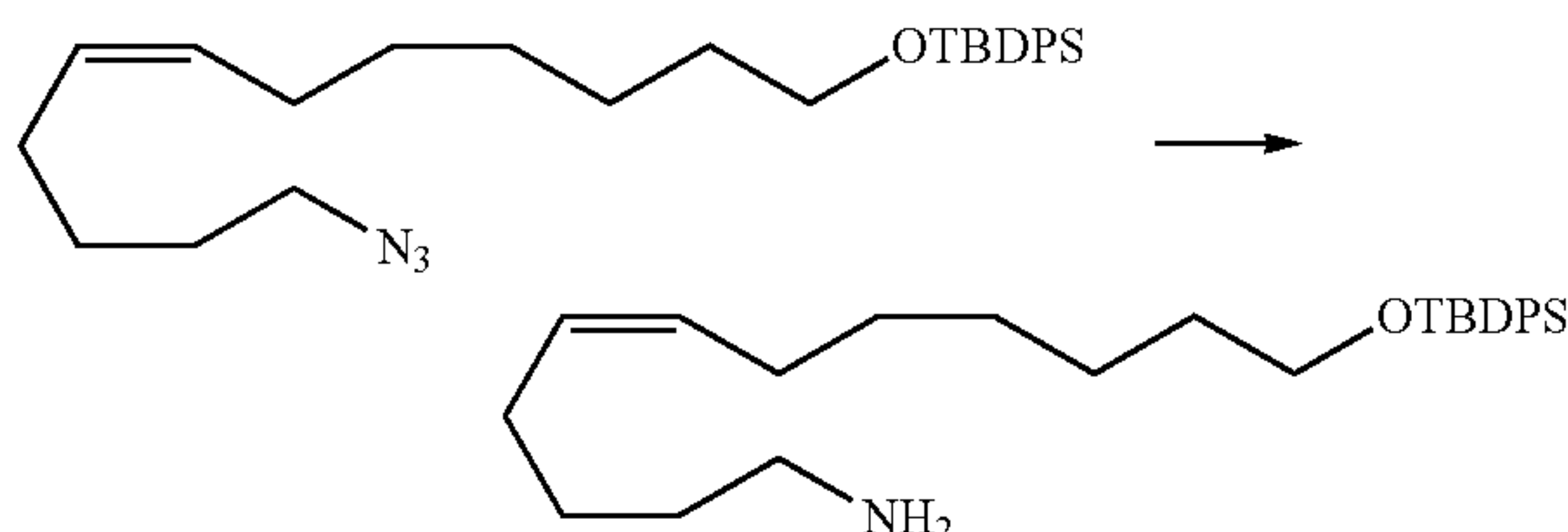
1-tert-Butyldiphenylsilyloxy-12-aminododec-7(Z)-ene
