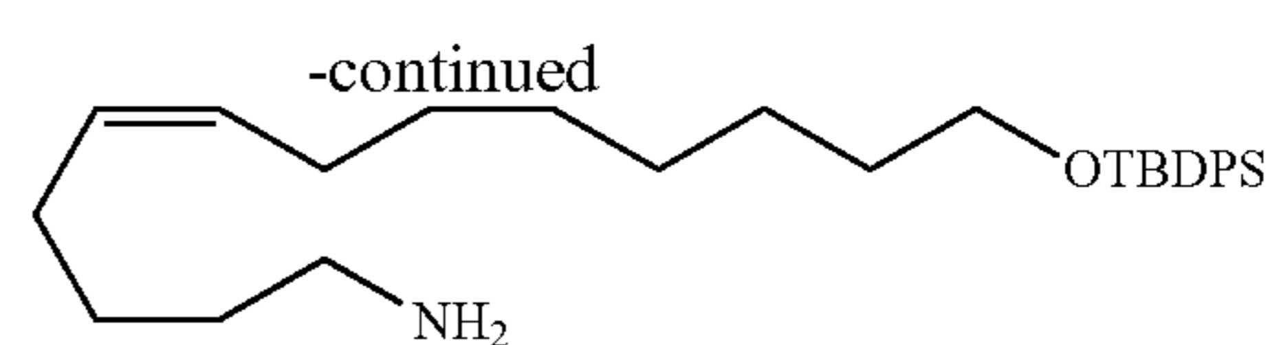
1-tert-Butyldiphenylsilyloxy-13-aminotridec-8(Z)-ene
