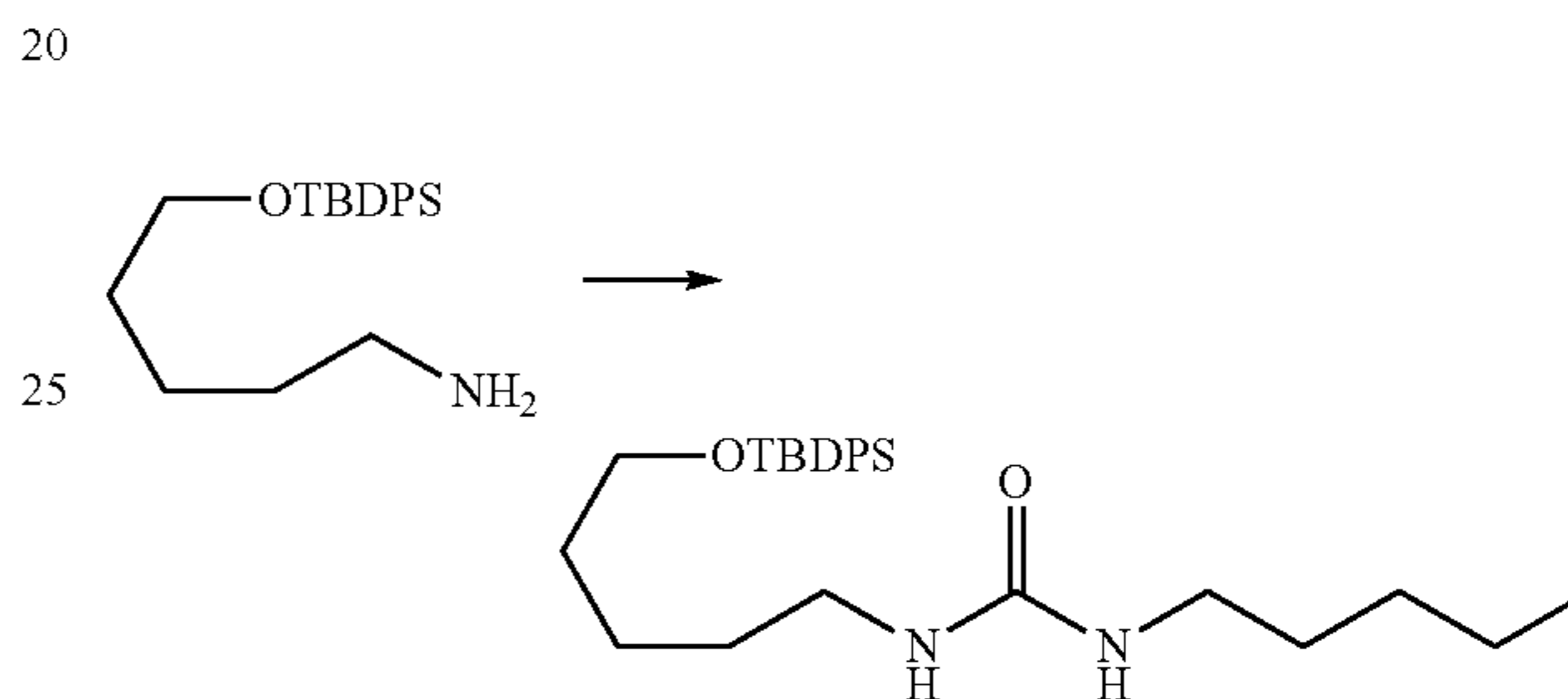
1-(5-(tert-Butyldiphenylsilyloxy)pentyl)-3-n-pentylurea
