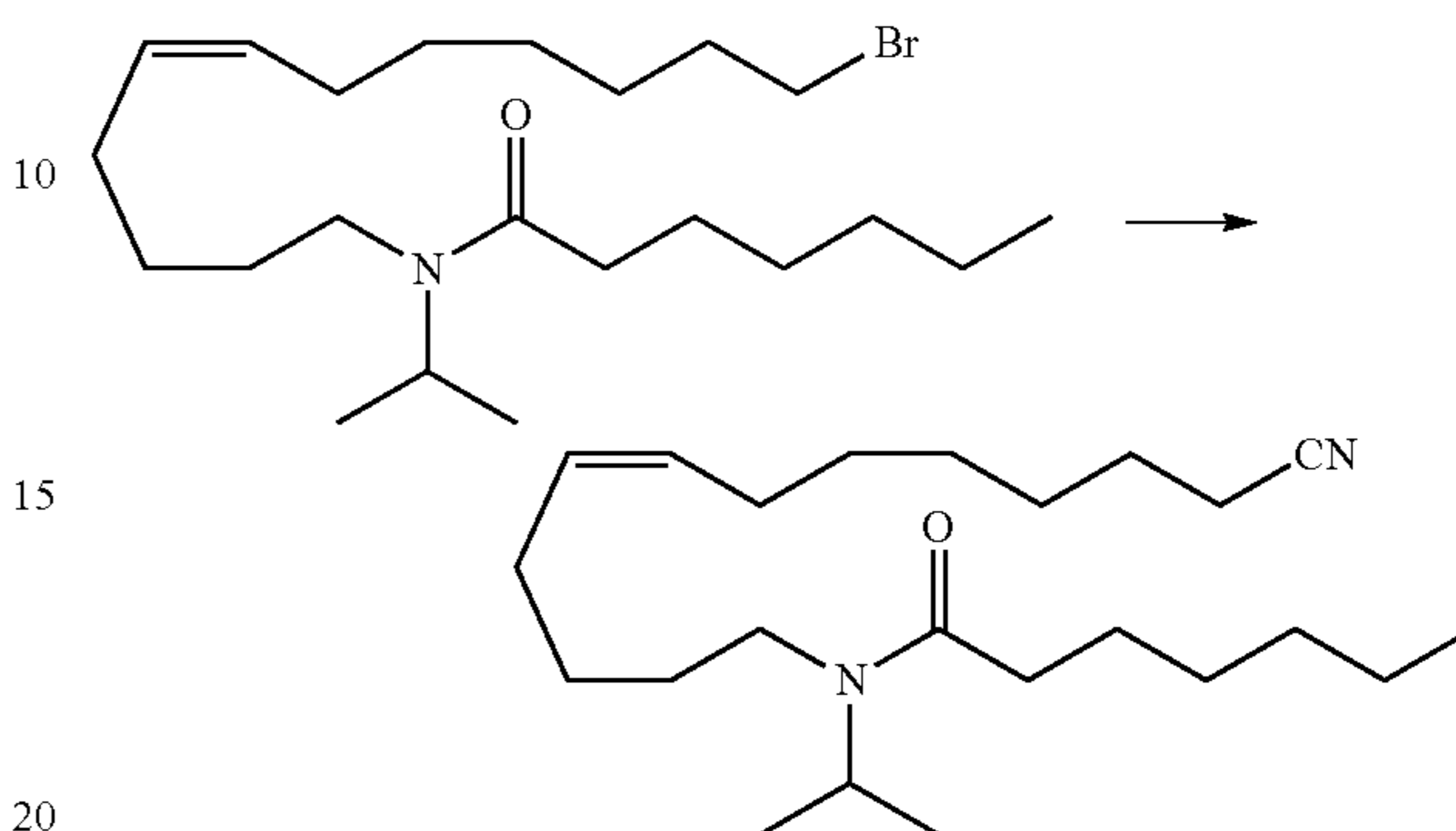
N-(12-Cyanododec-5(Z)-enyl)-N-isopropyl-n-hexanamide
