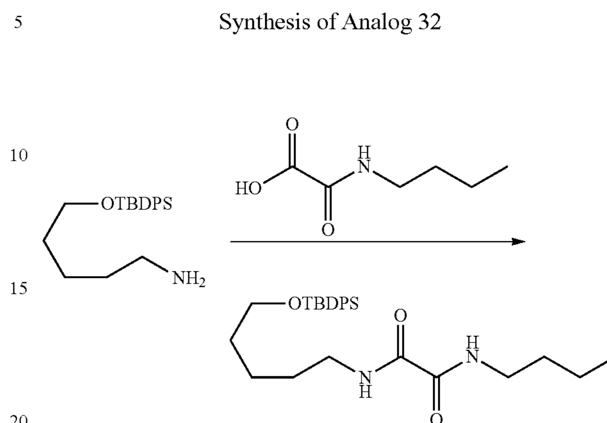
N 1 -n-Butyl-N 2 -(5-(tert-butyl-diphenylsilyloxy)pentyl)oxalamide
