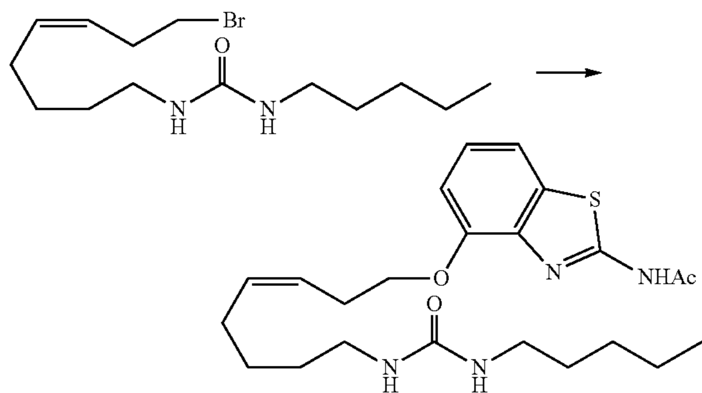
N-(4-(8-(3-n-Pentylureido)oct-3(Z)-enyloxy)benzo[d]thiazol-2-yl)acetamide (33)
