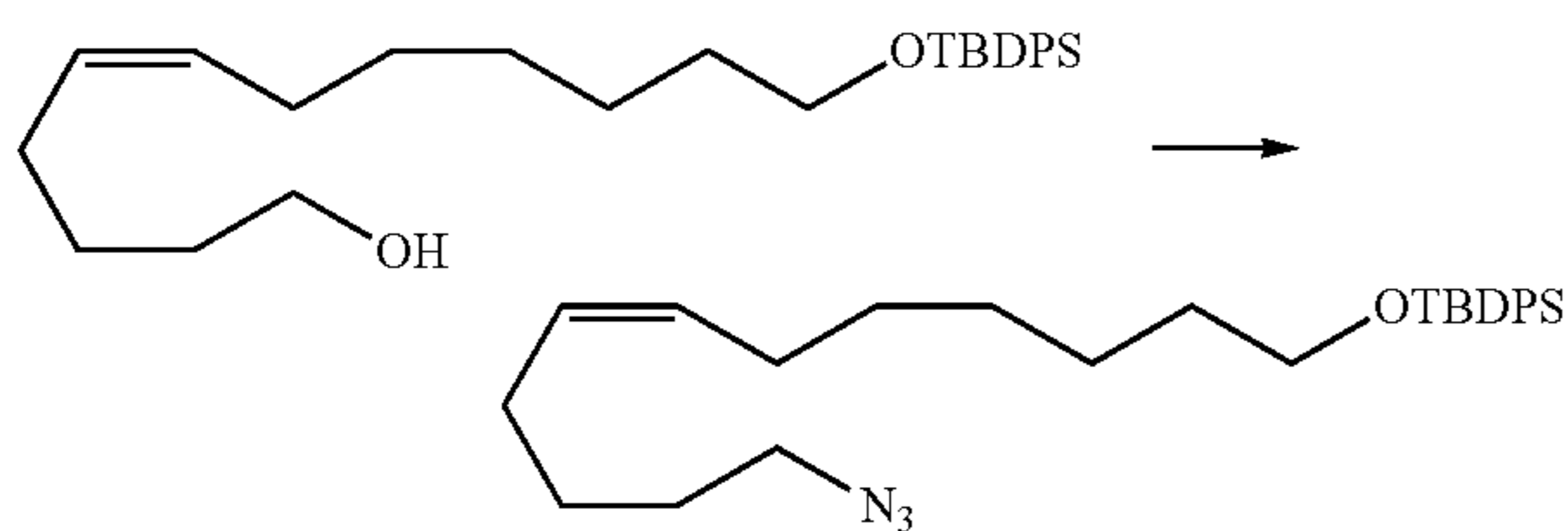
1-tert-Butyldiphenylsilyloxy-12-azidododec-7(Z)-ene
