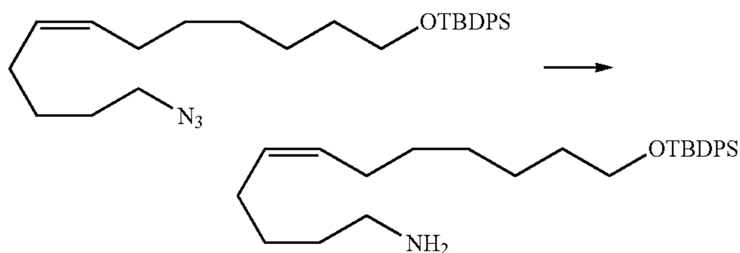
1-tert-Butyldiphenylsilyloxy-12-aminododec-7(Z)-ene
