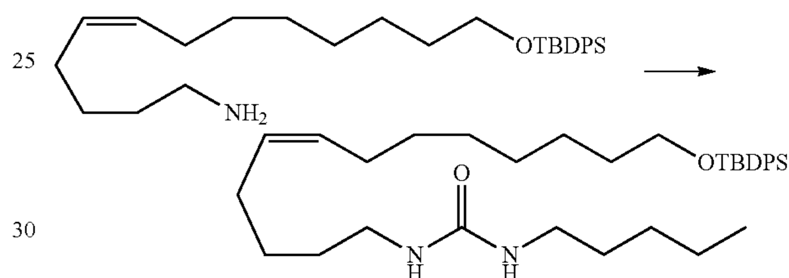
1-(13-(tert-Butyldiphenylsilyloxy)tridec-5(Z)-enyl)-3-n-pentylurea
