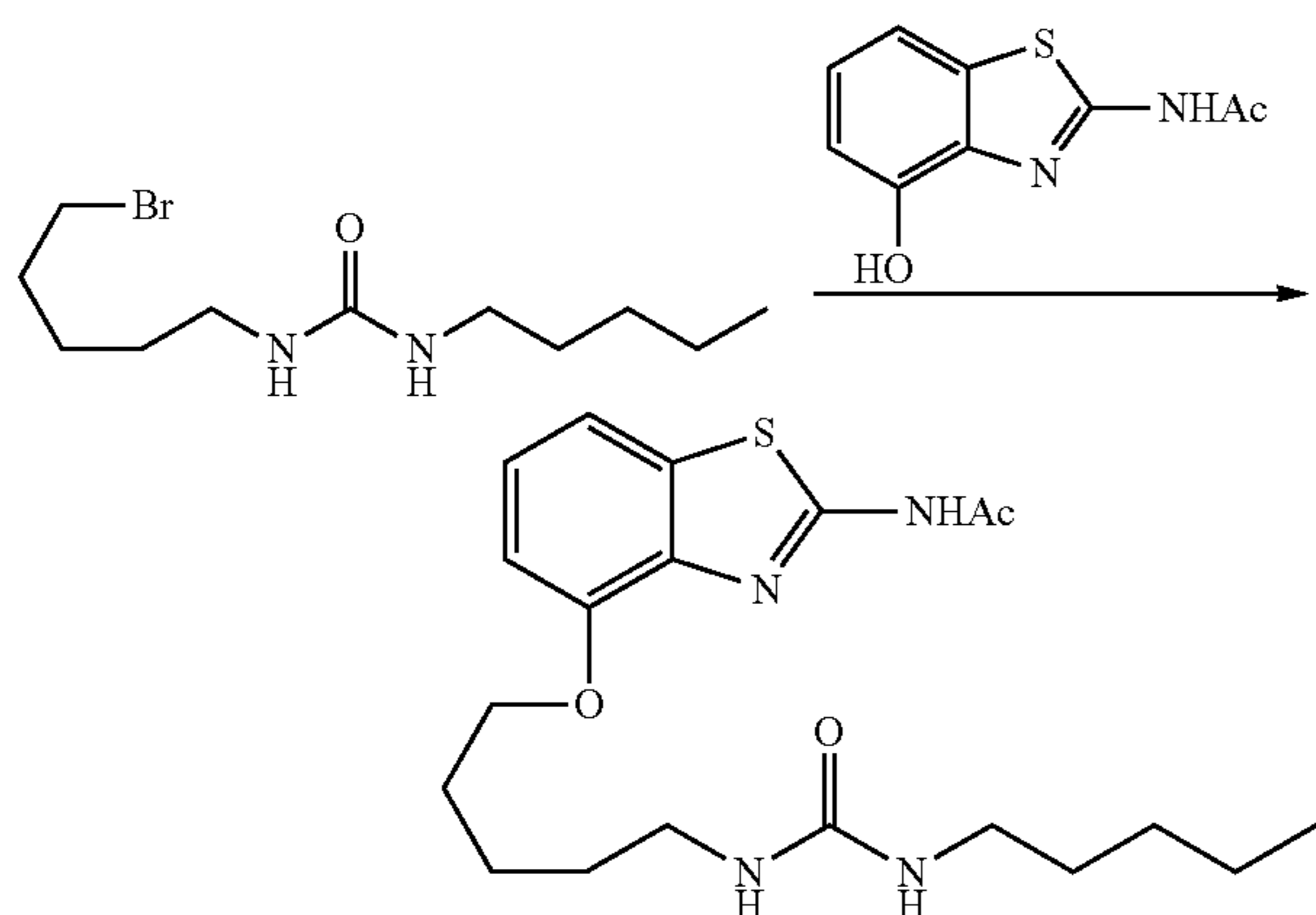
N-(4-(5-(3-n-Pentylureido)pentyl)oxy)benzo[d]thiazol-2-yl)acetamide (31)
