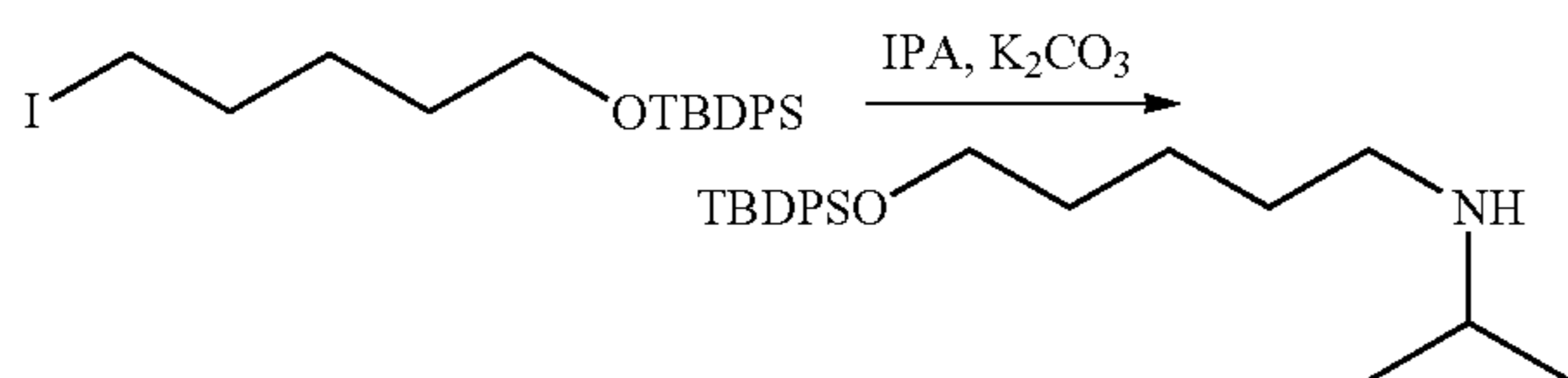
5-(tert-Butyldiphenylsilyloxy)-N-isopropylpentan-1-amine (4)
