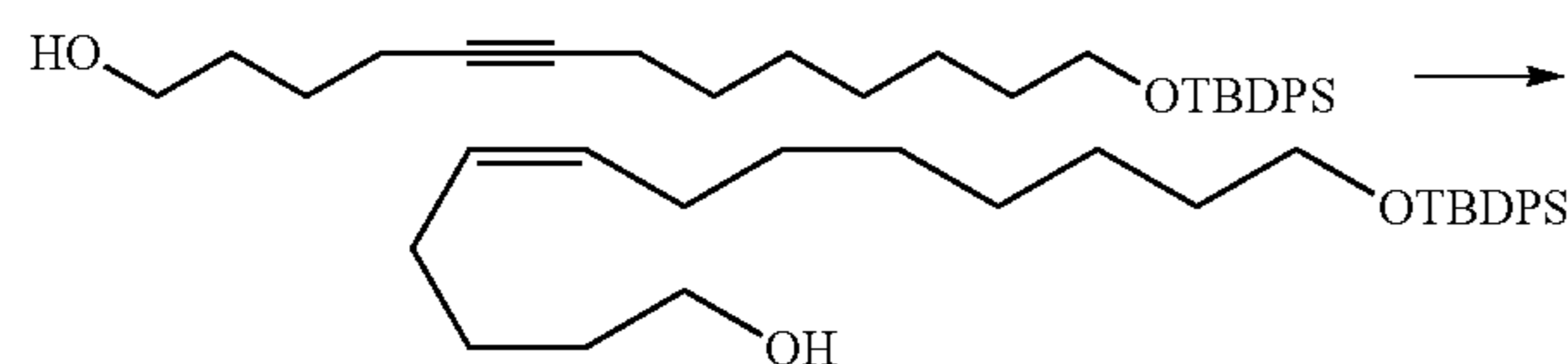
(Z)-13-(tert-Butyldiphenylsilyloxy)tridec-5-en-1-ol
