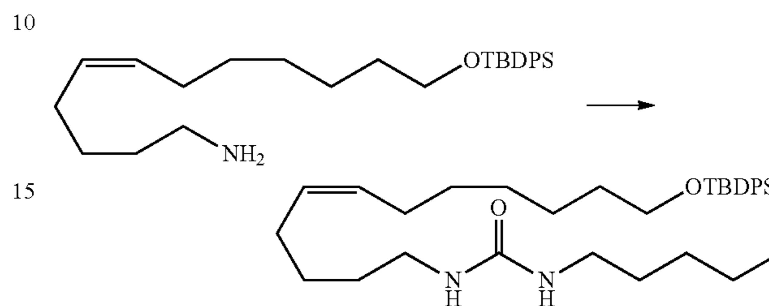
1-(12-(tert-Butyldiphenylsilyloxy)dodec-5(Z)-enyl)-3-n-pentylurea
