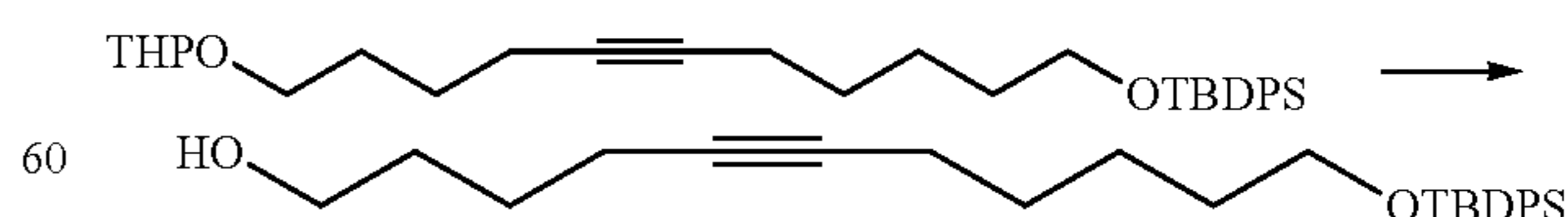
1-(tert-Butyldiphenylsilyloxy)undec-5-yn-1-ol
