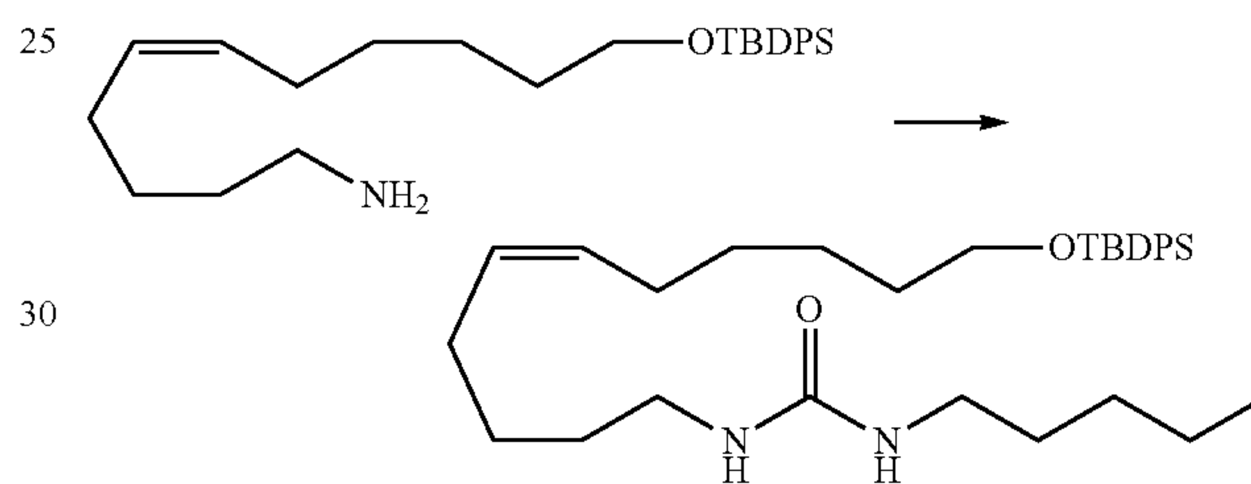
1-(11-(tert-Butyldiphenylsilyloxy)undec-5(Z)-enyl)-3-n-pentylurea
