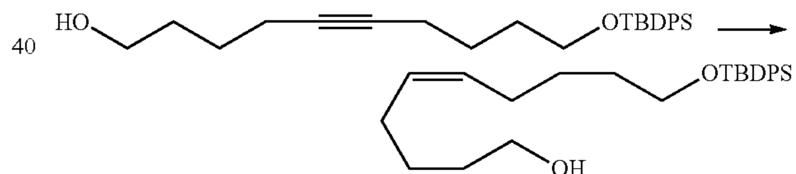
10-(tert-Butyldiphenylsilyloxy)dec-5(Z)-en-1-ol
