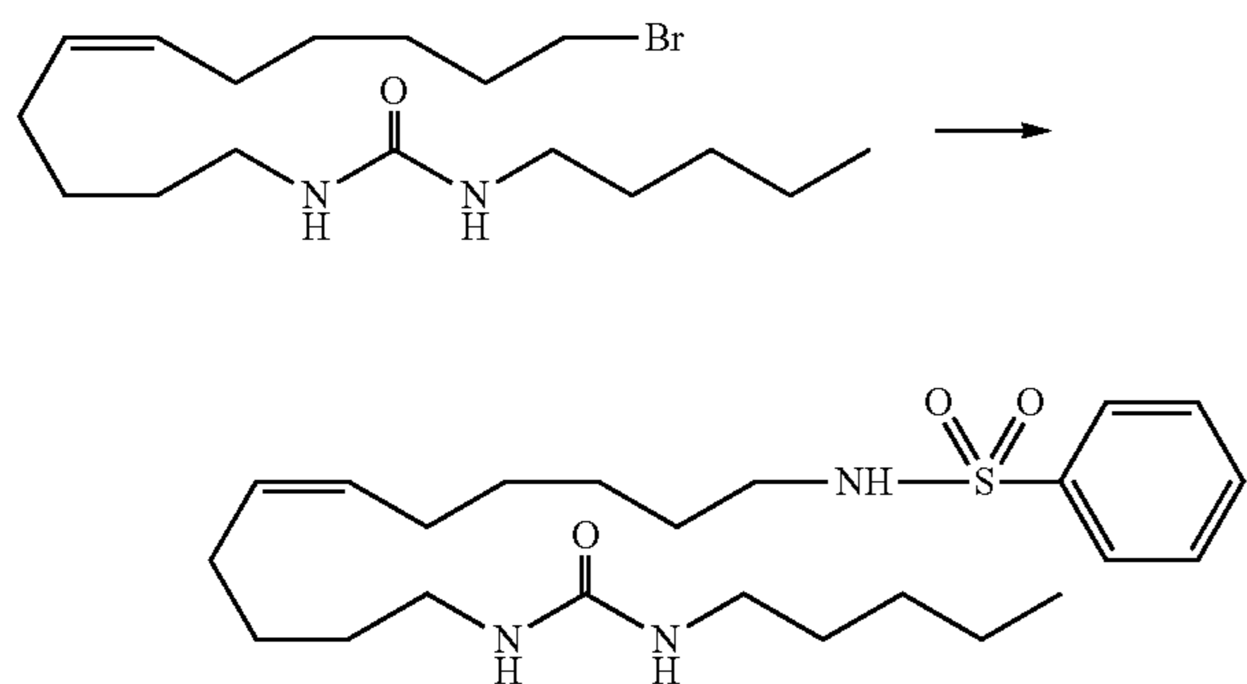
N-(11-(3-n-Pentylureido)undec-6(Z)-enyl)benzenesulfonamide (12)
