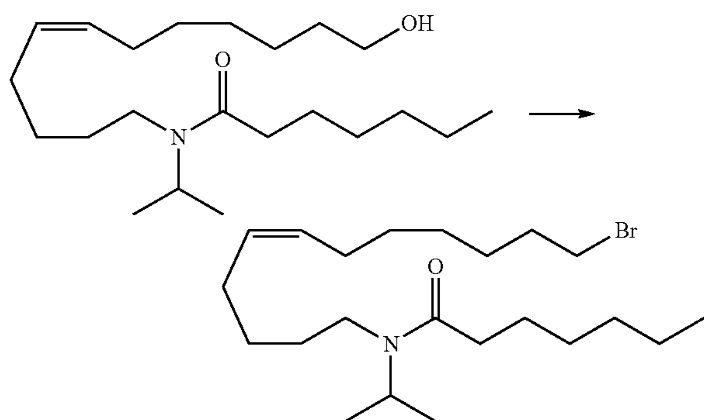
N-(12-Bromododec-5(Z)-enyl)-N-isopropyl-n-hexanamide
