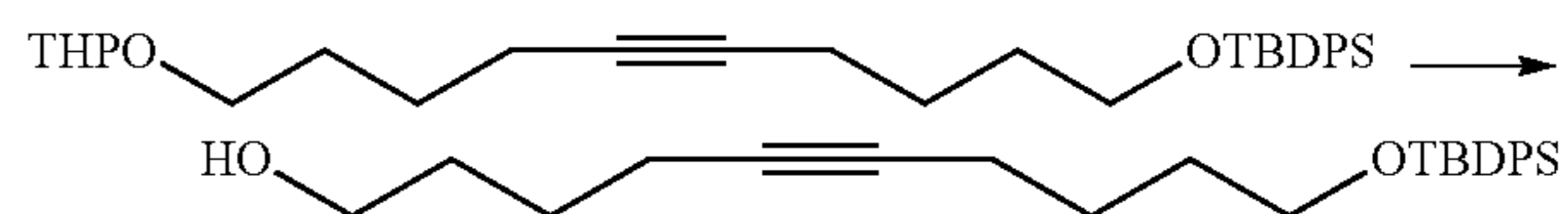
10-(tert-Butyldiphenylsilyloxy)dec-5-yn-1-ol
