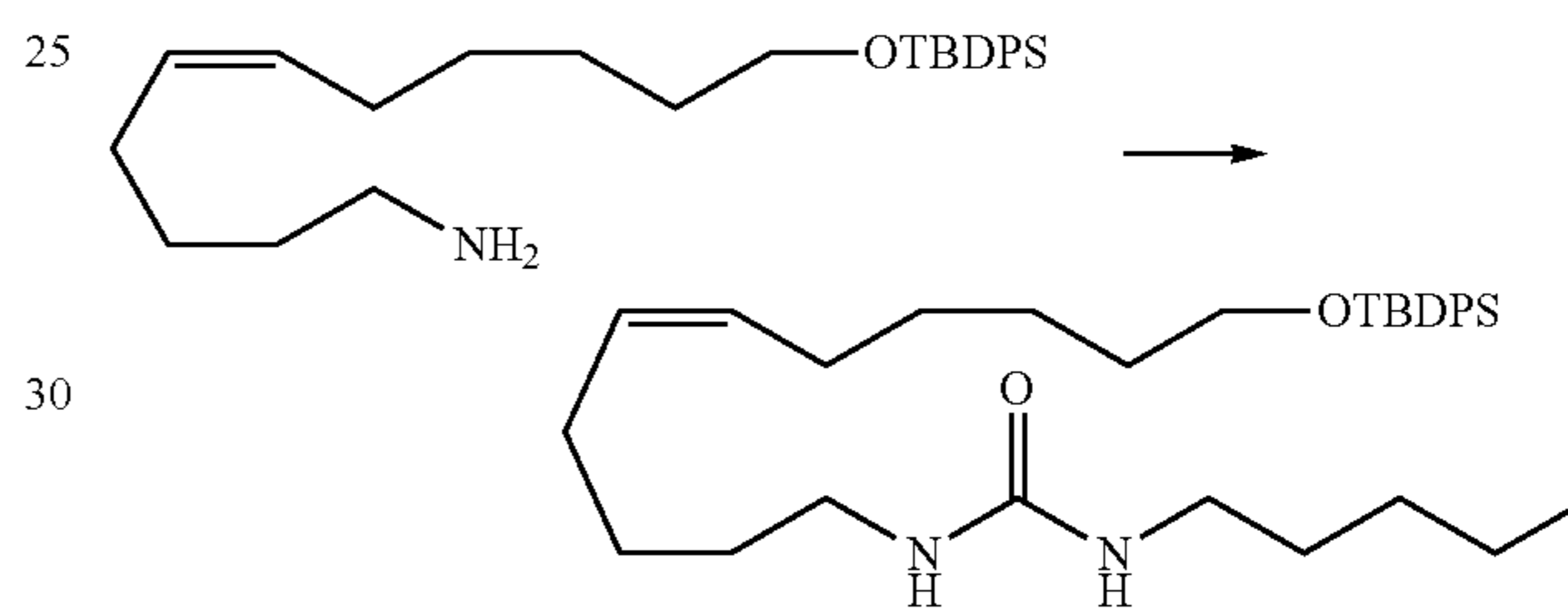
1-(11-(tert-Butyldiphenylsilyloxy)undec-5(Z)-enyl)-3-n-pentylurea
