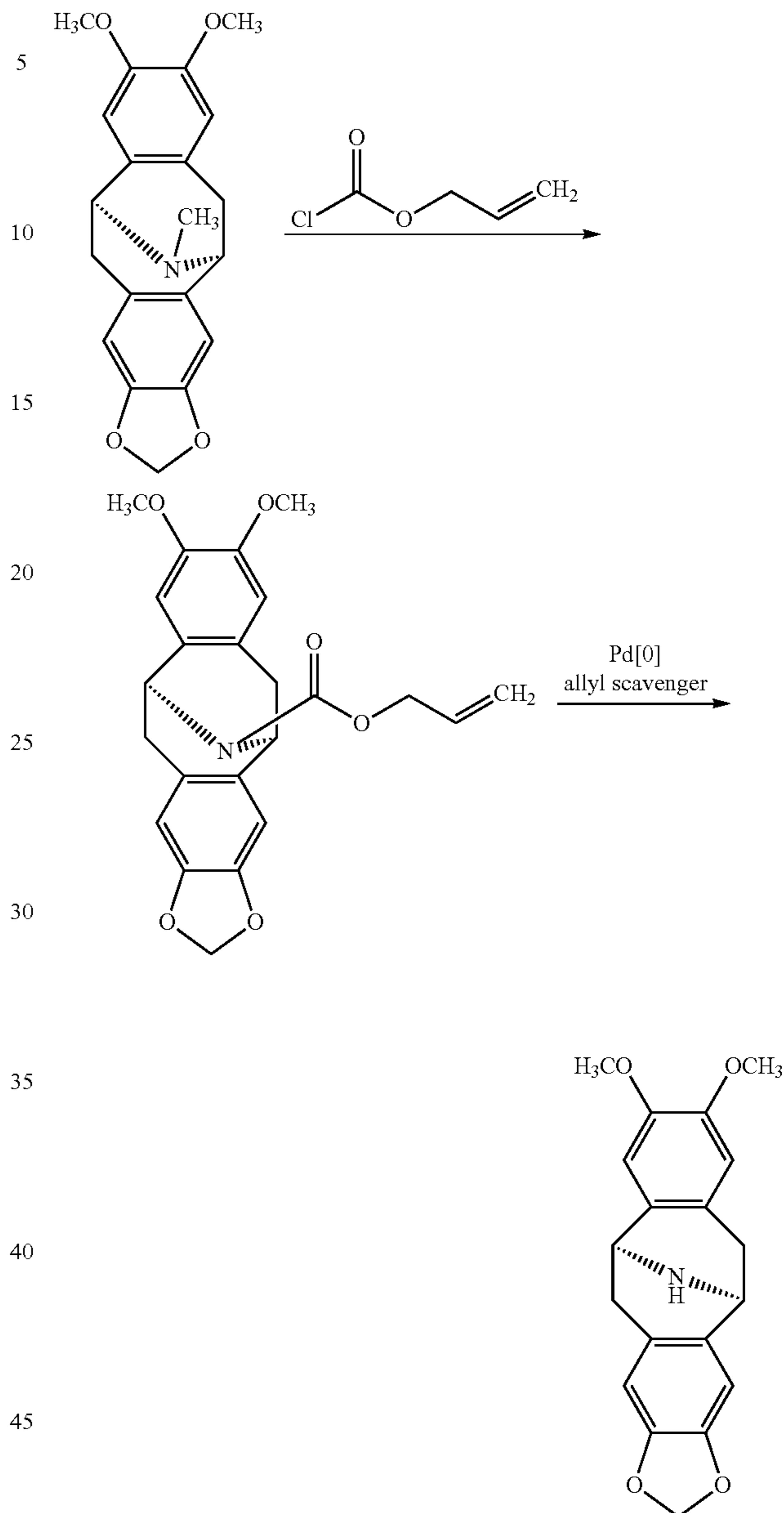
Scheme 26: (+)-Eschscholtzidine
