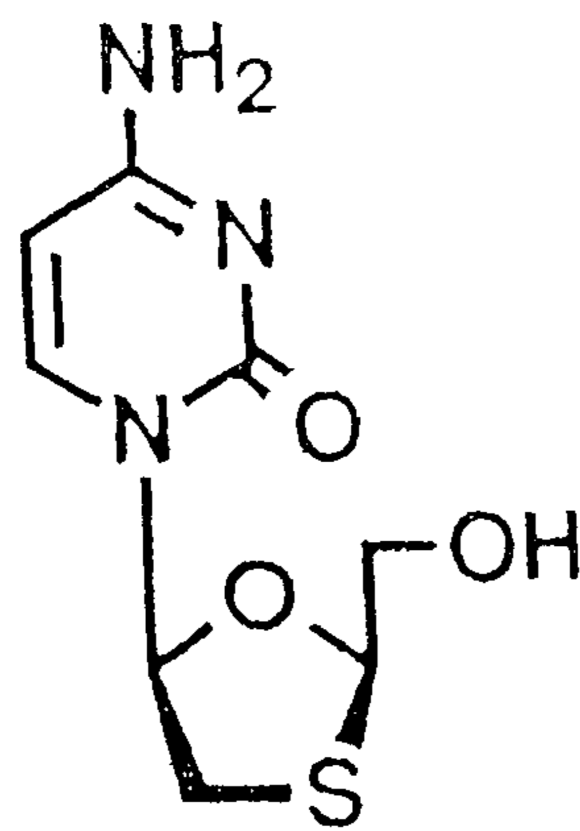
L(-)SddC (3TC)
