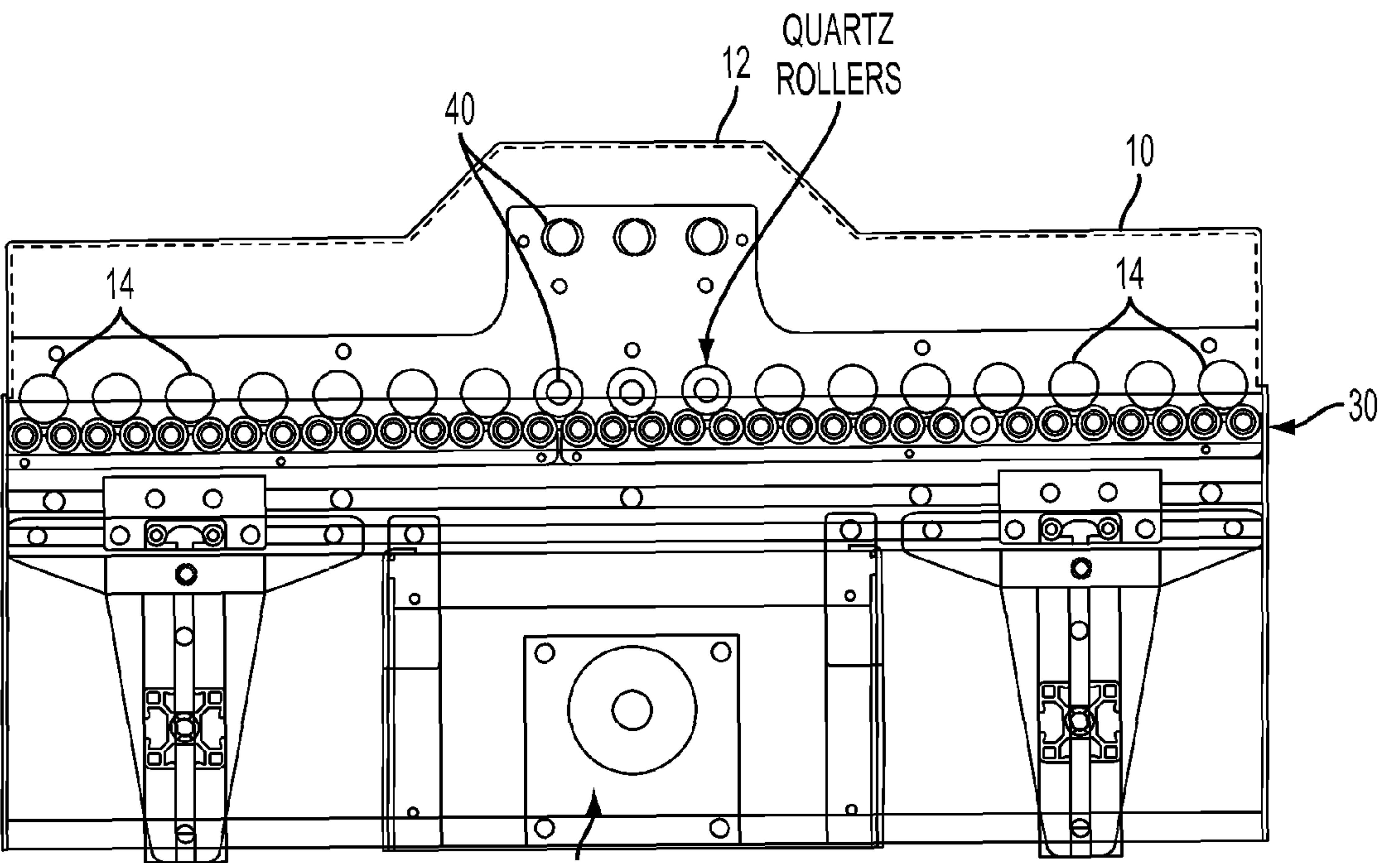
MOTOR FIG. 3
