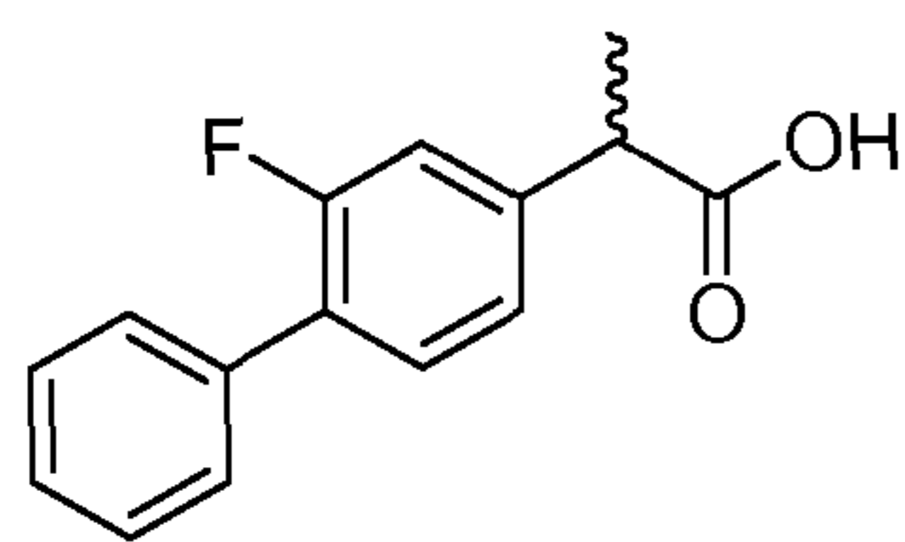
flurbiprofen
