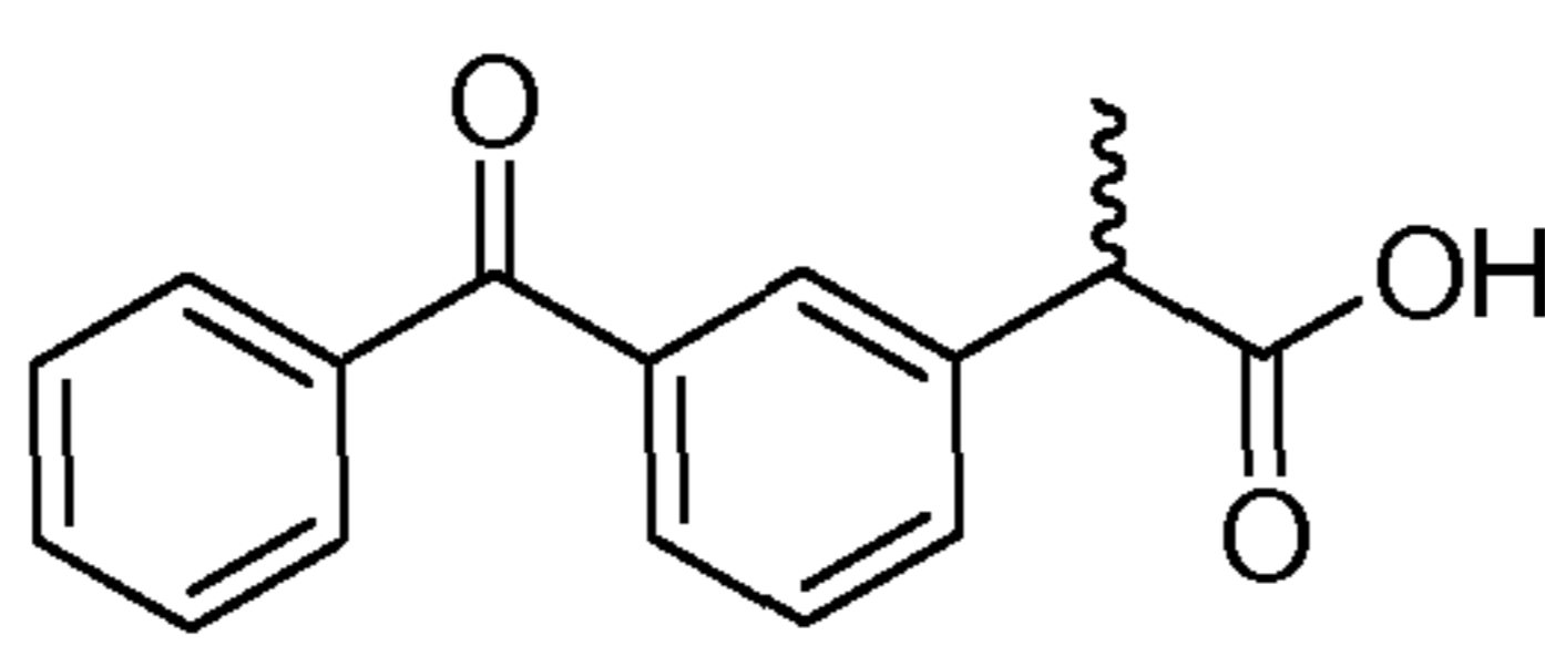
ketoprofen
