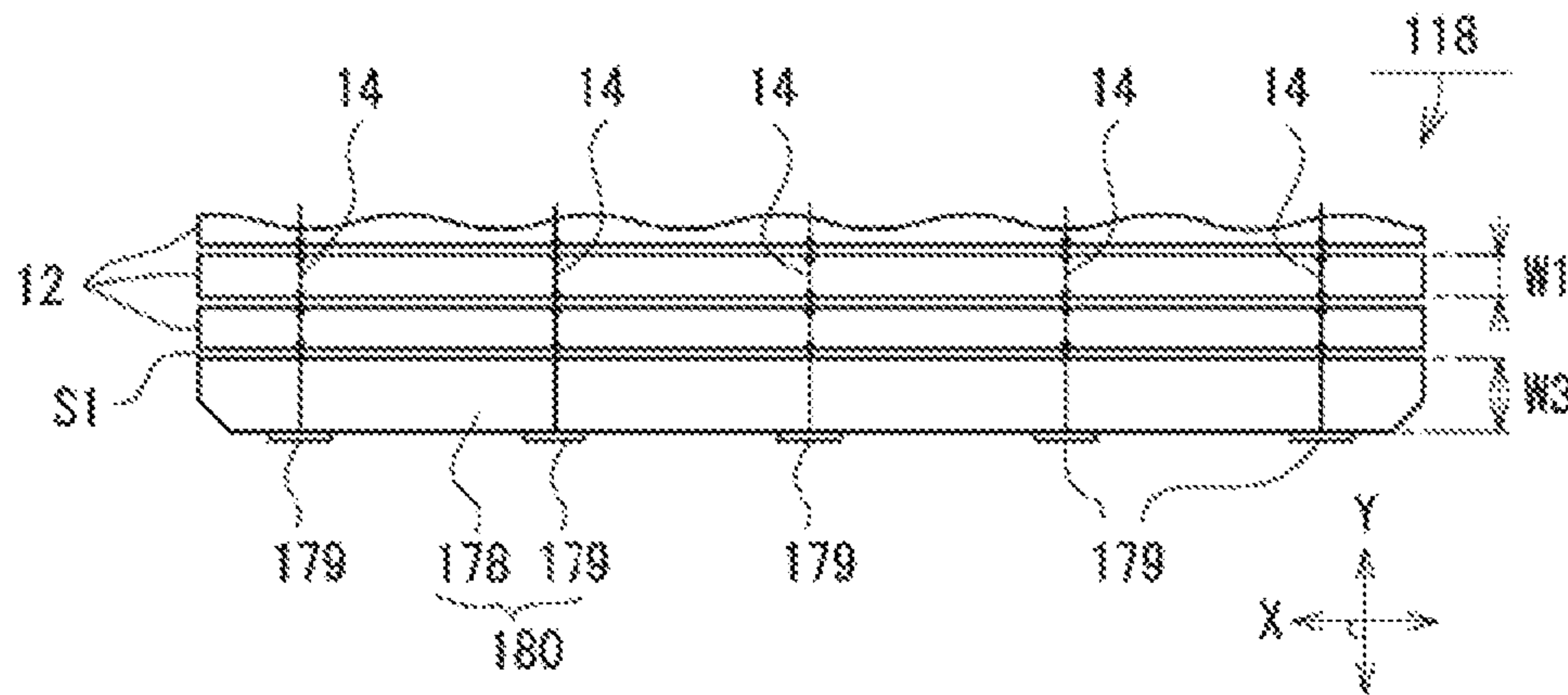
Fig. 19(c)
