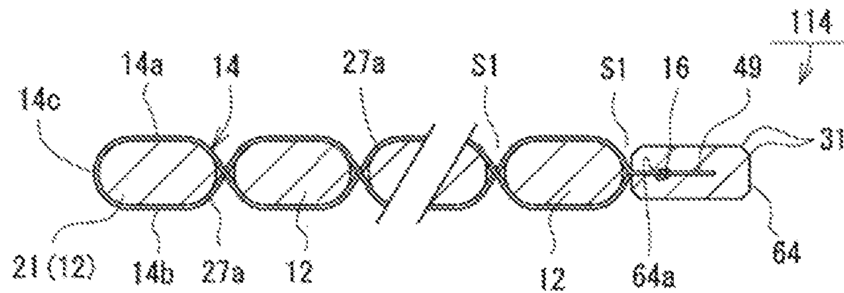
Fig. 15(d)
