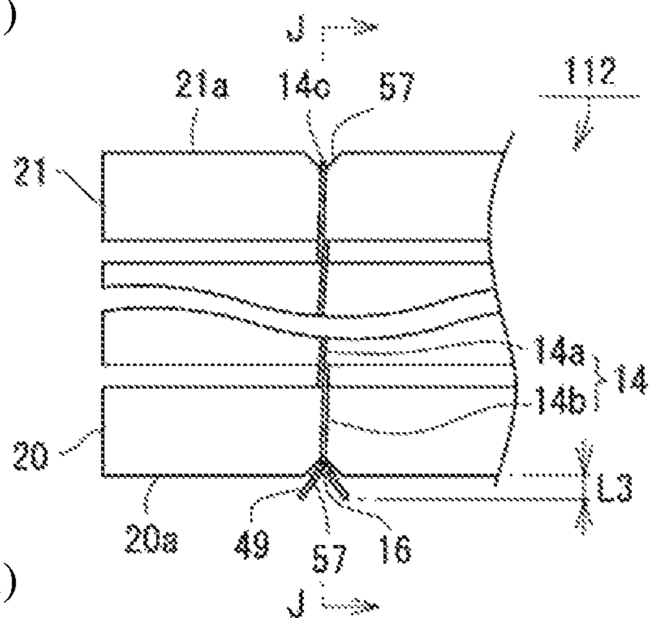
Fig. 14(c)
