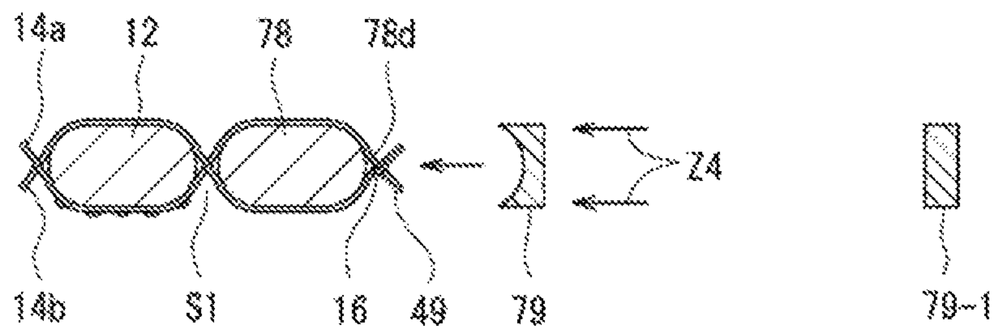
Fig. 18(e)
