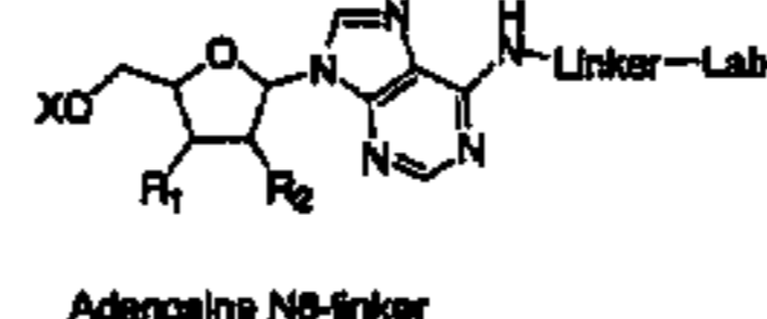
Adenosine N6-linker
