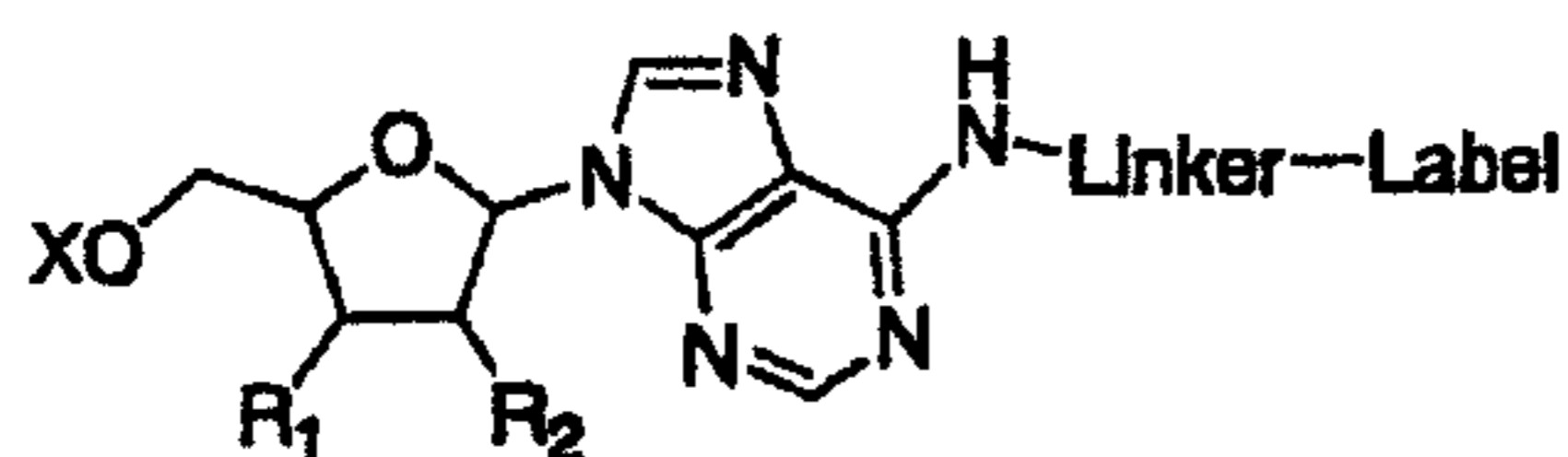
Adenosine N6-linker
