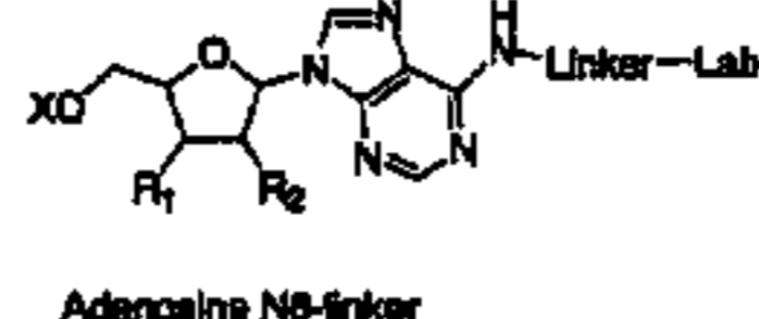
Adenosine N6-linker
