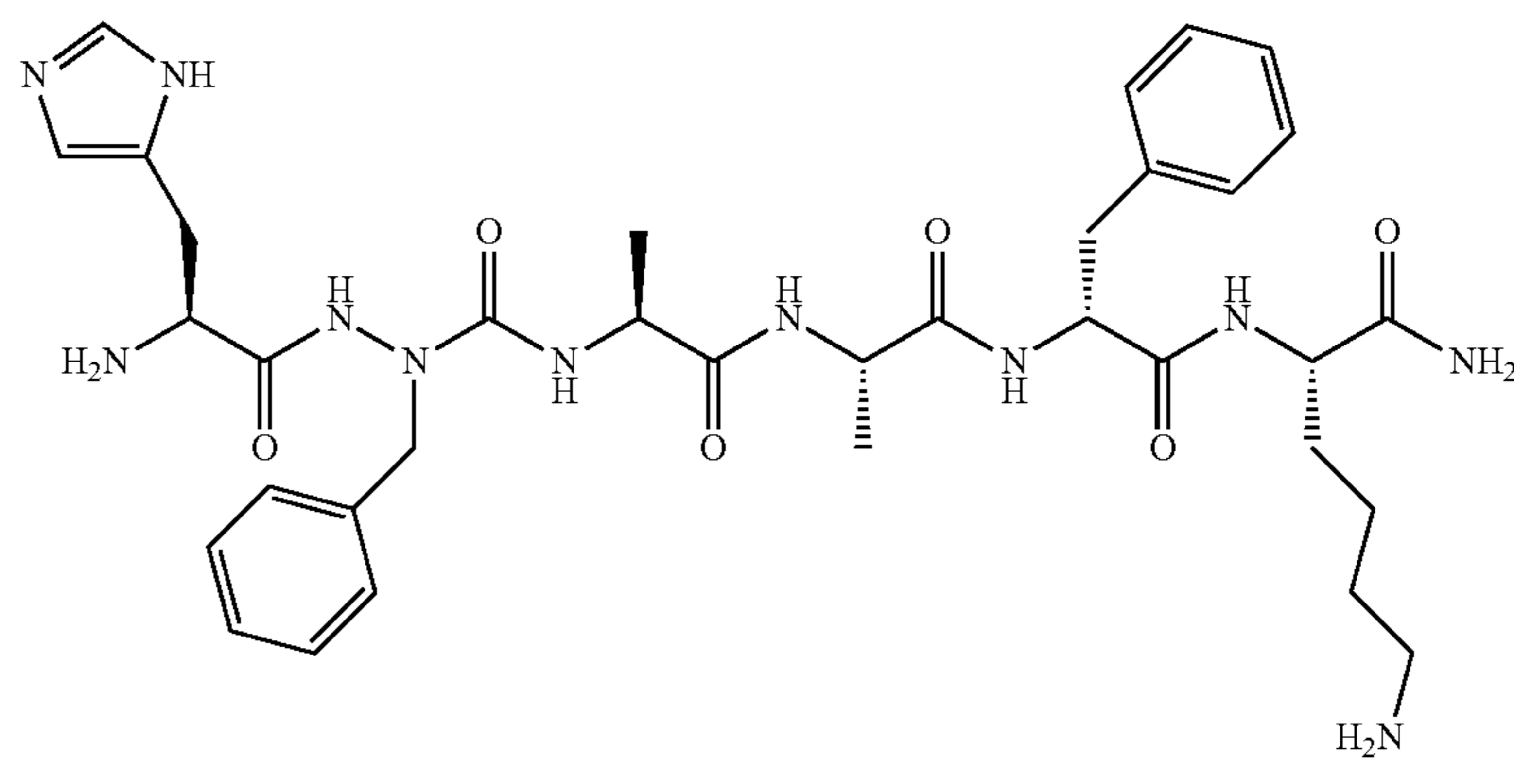
(D/L)His-azaPhe-Ala-Ala-D-Phe-Lys-NH 2
