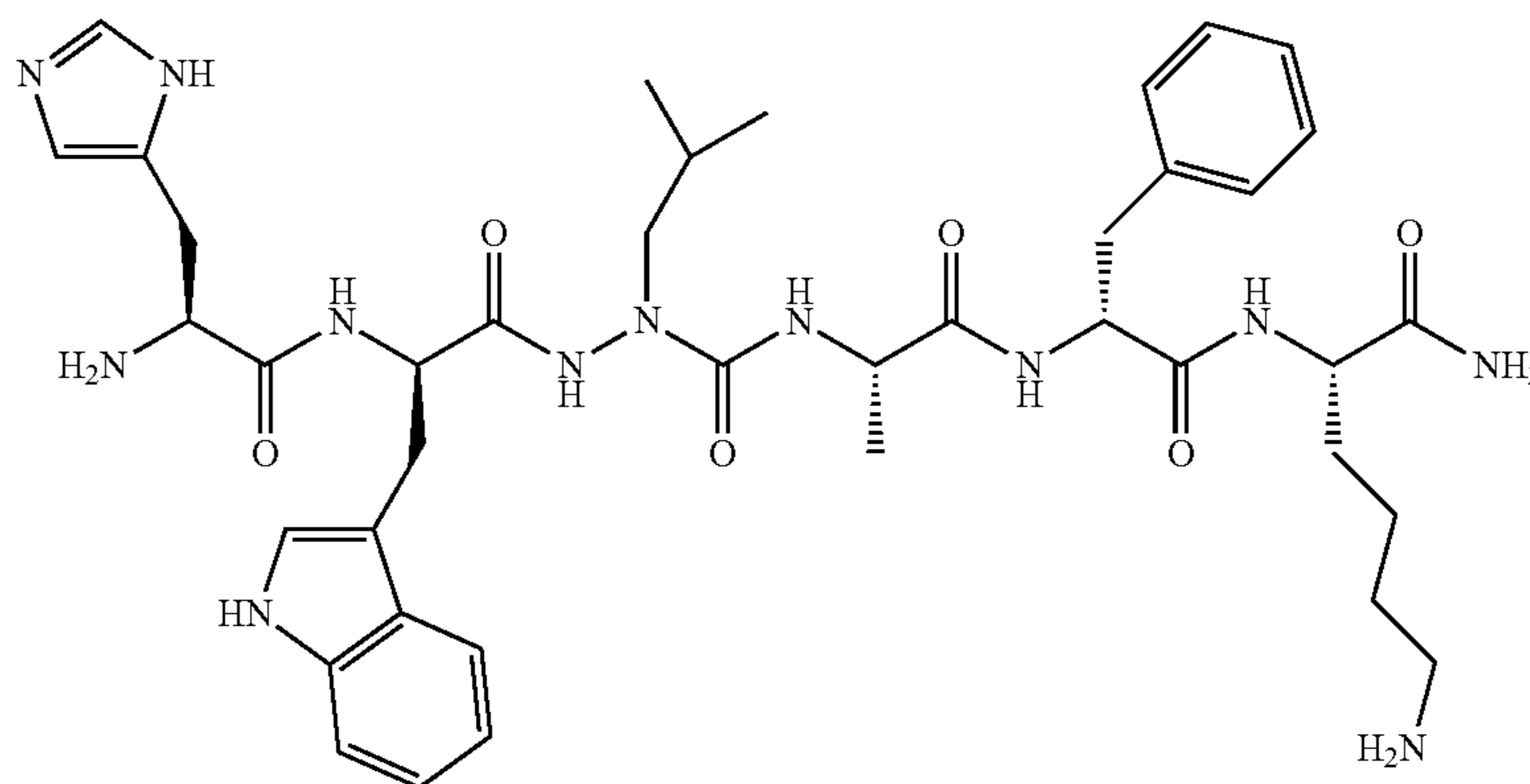
His-D-Trp-azaLeu-Ala-D-Phe-Lys-NH 2
