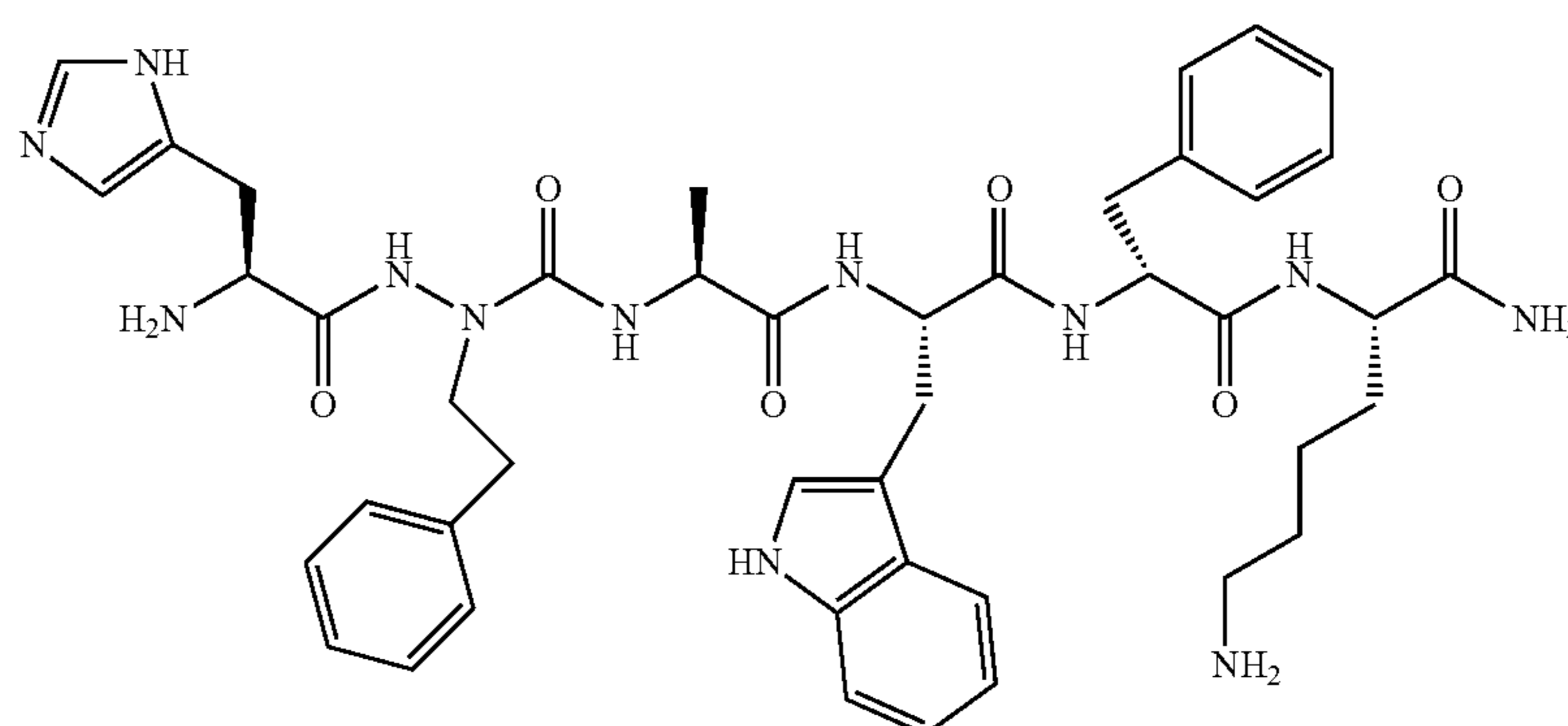
His-azahomoPhe-Ala-Trp-D-Phe-Lys-NH 2
