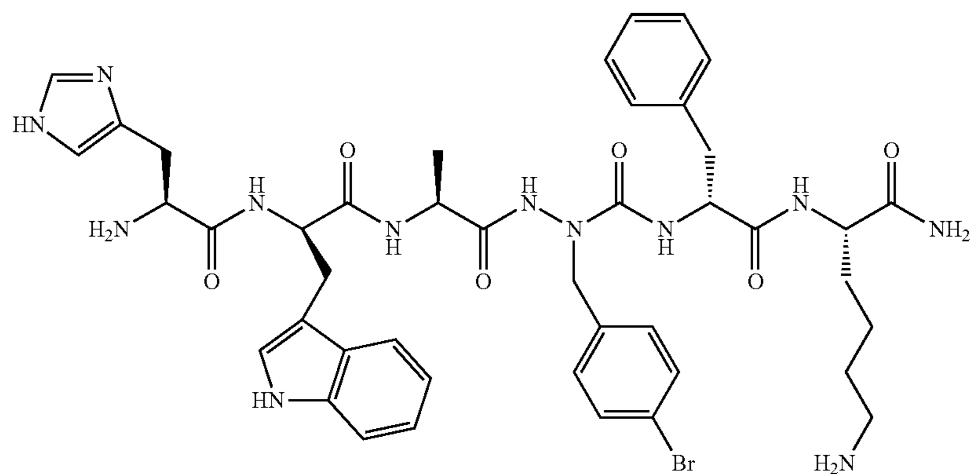
His-D-Trp-Ala-aza-(p-bromo)Phe-D-Phe-Lys-NH 2
