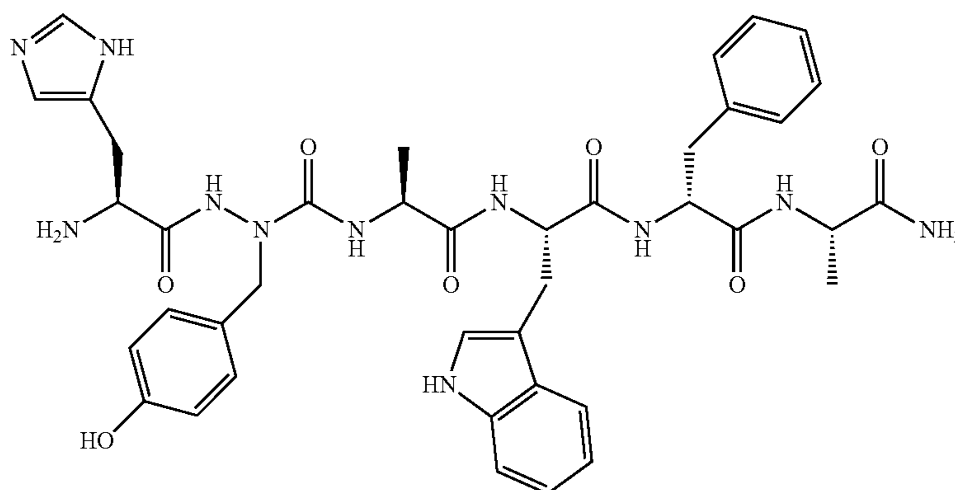
His-azaTyr-Ala-Trp-D-Phe-Ala-NH 2
