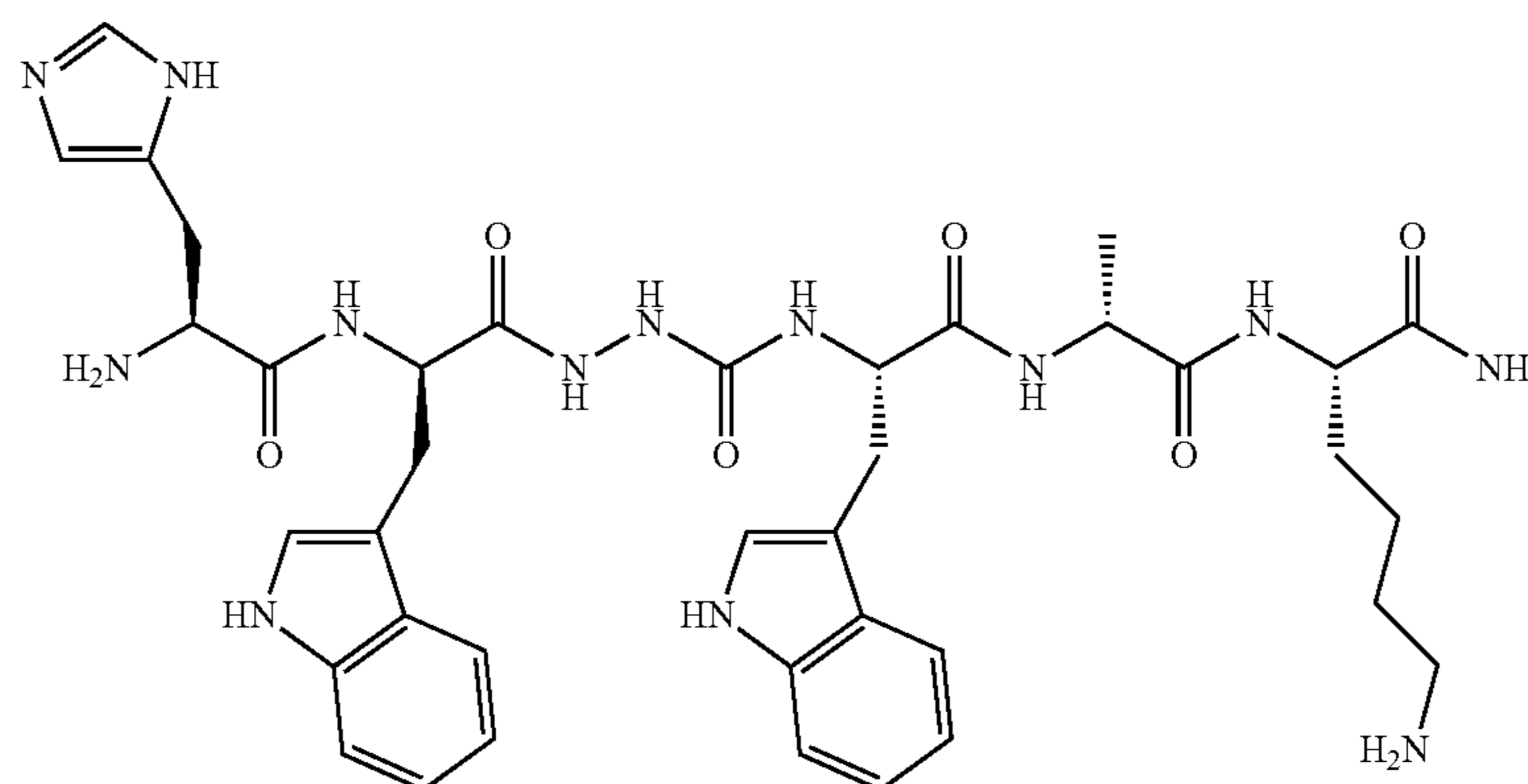
His-D-Trp-azaGly-Trp-D-Ala-Lys-NH 2
