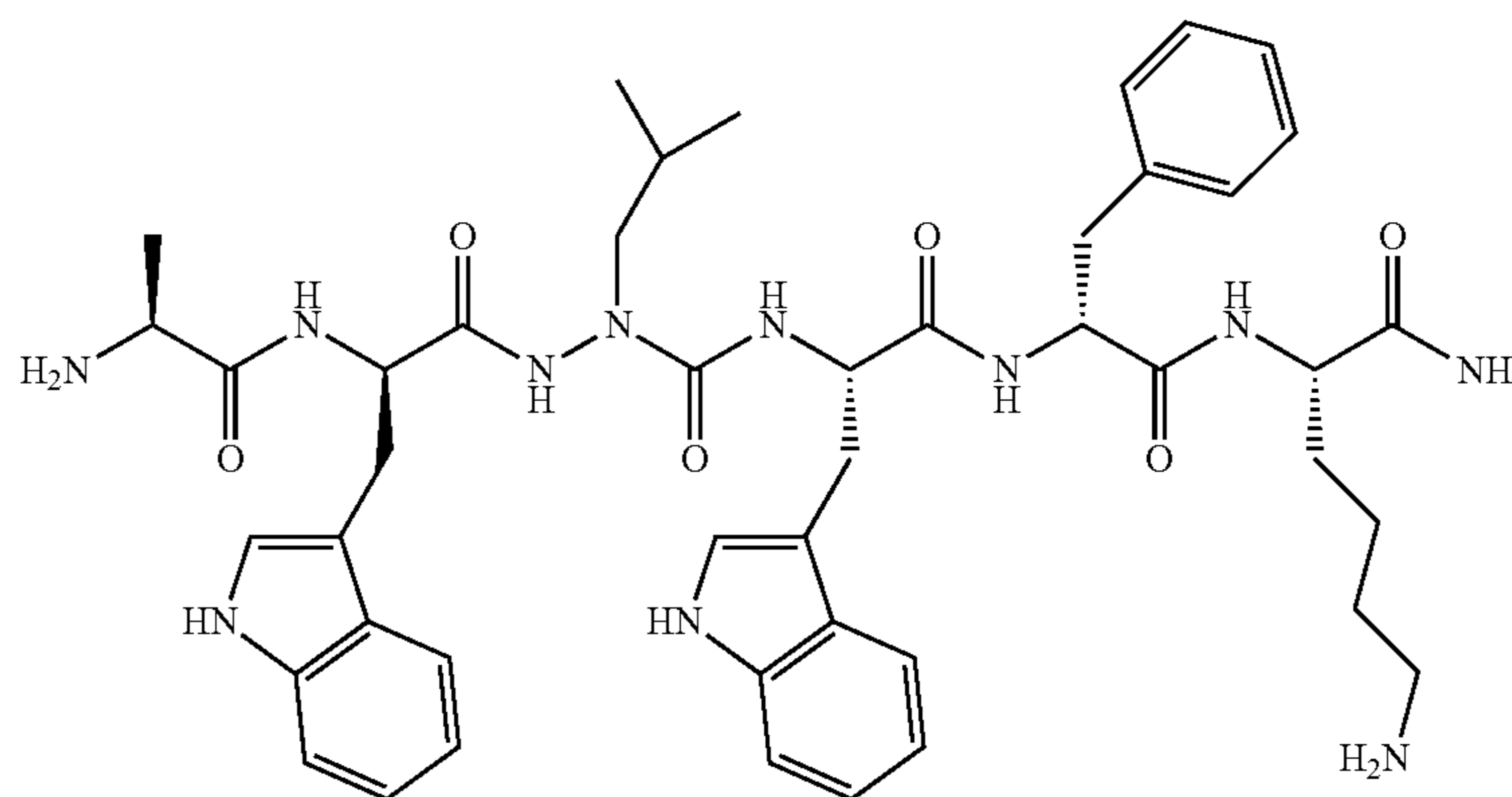
Ala-D-Trp-azaLeu-Trp-D-Phe-Lys-NH 2
