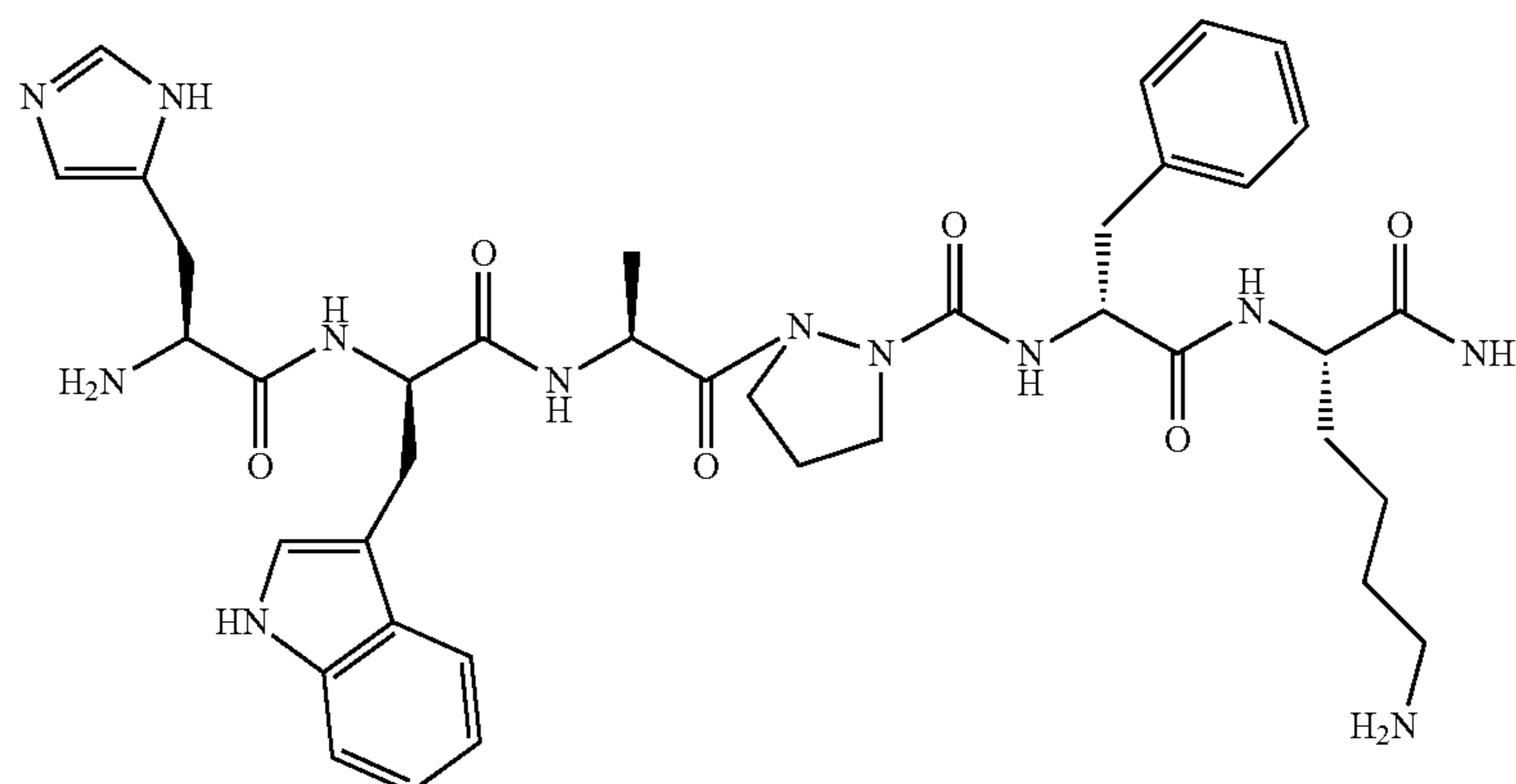
His-D-Trp-Ala-azaPro-D-Phe-Lys-NH 2
