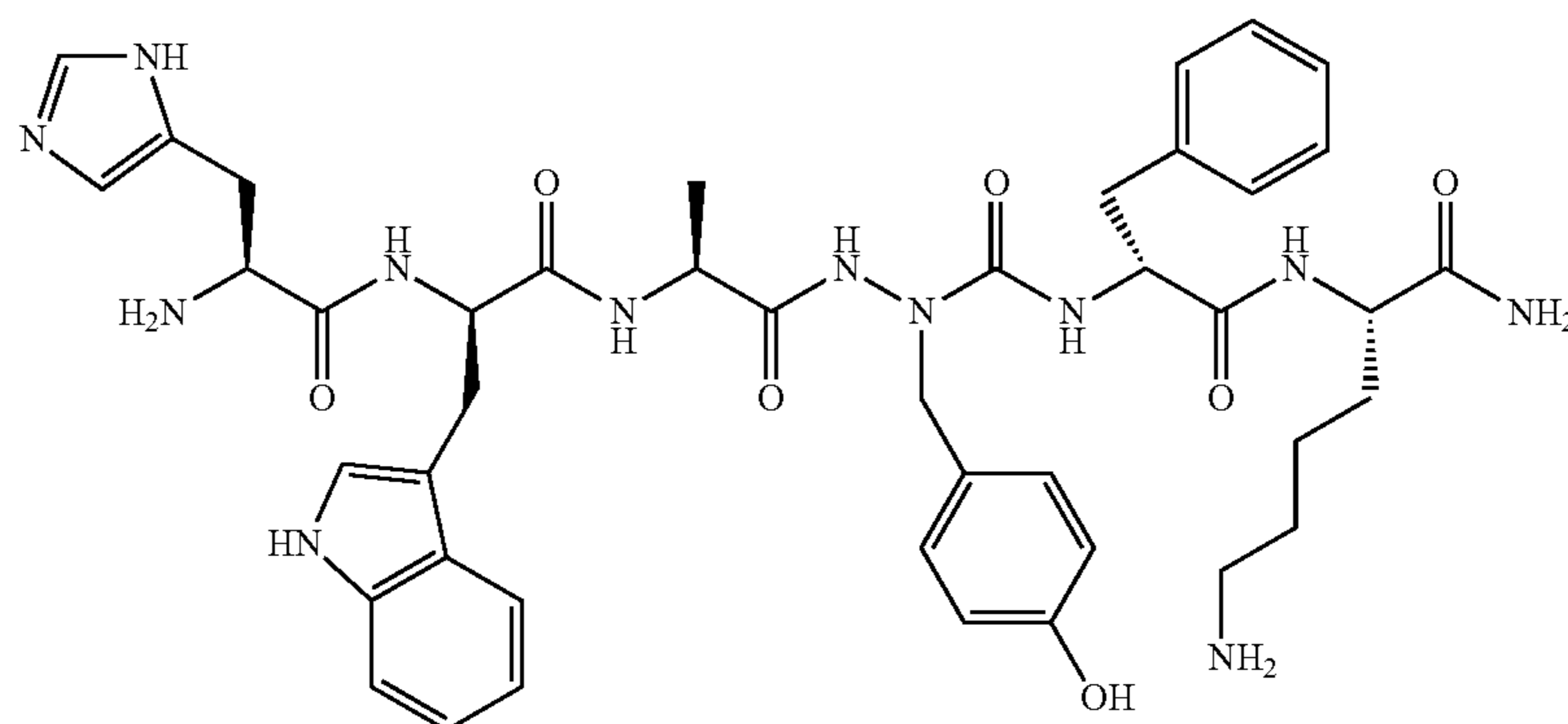
His-D-Trp-Ala-azaTyr-D-Phe-Lys-NH 2
