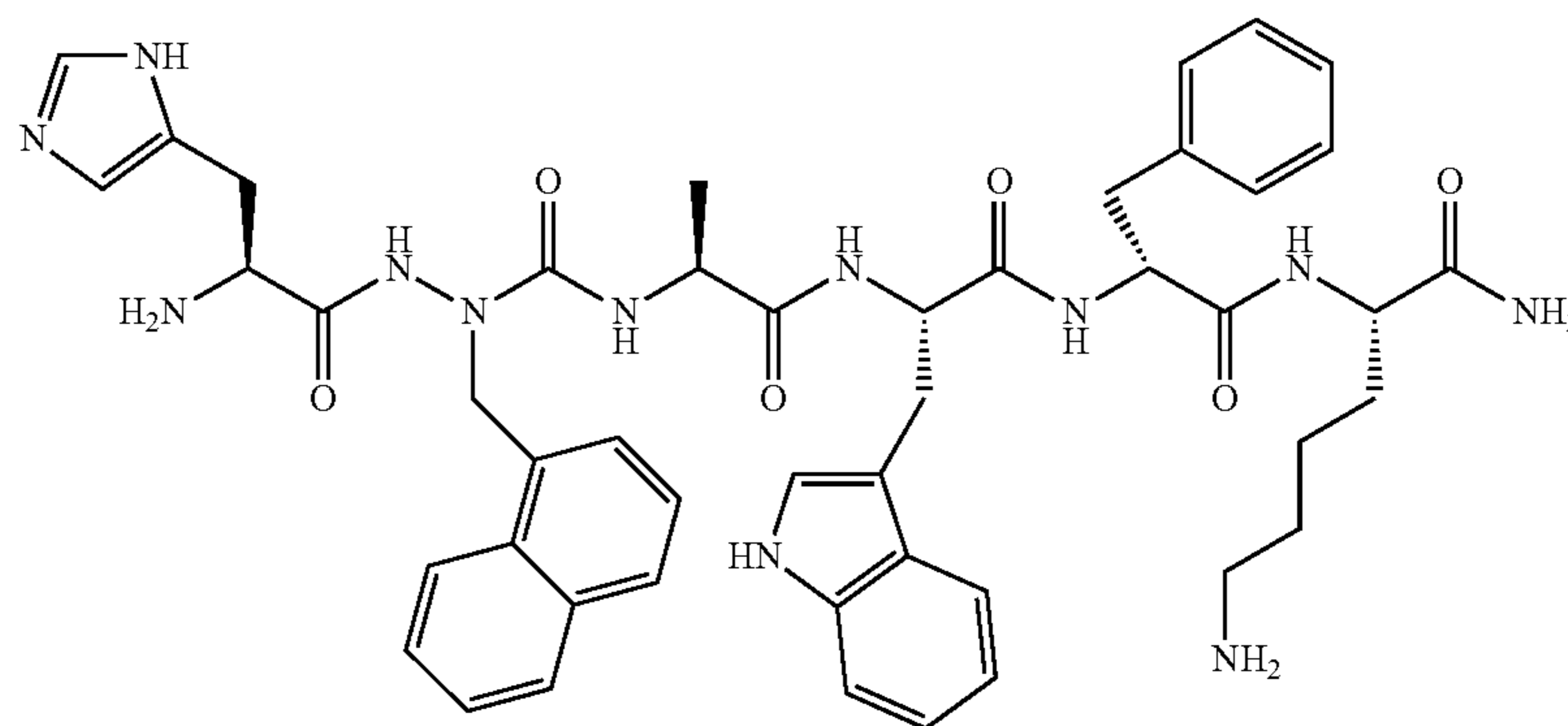
His-azaNal-1-Ala-Trp-D-Phe-Lys-NH 2
