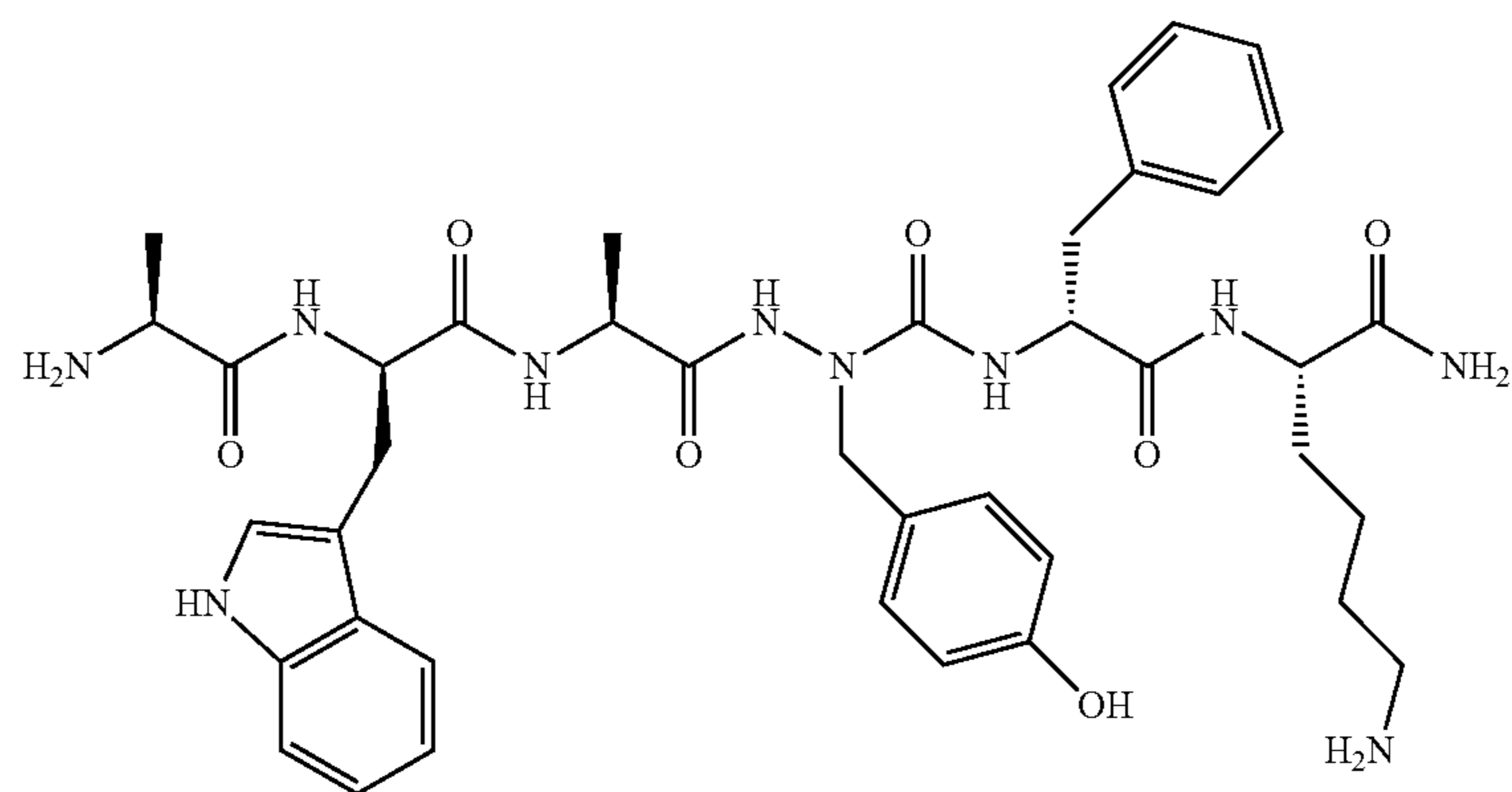
Ala-D-Trp-Ala-AzaTyr-D-Phe-Lys-NH 2
