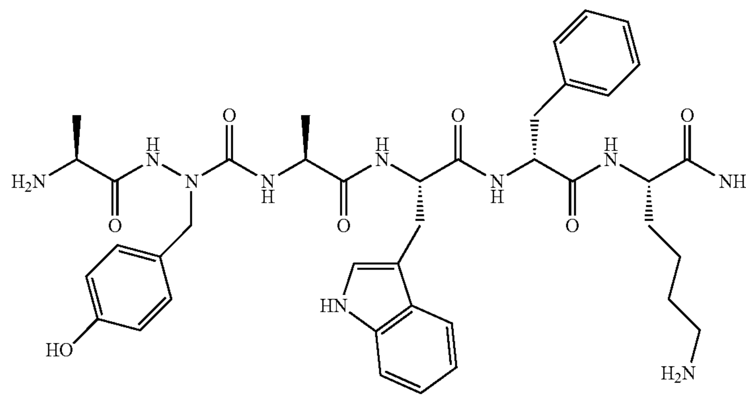
Ala-azaTyr-Ala-Trp-D-Phe-Lys-NH 2
