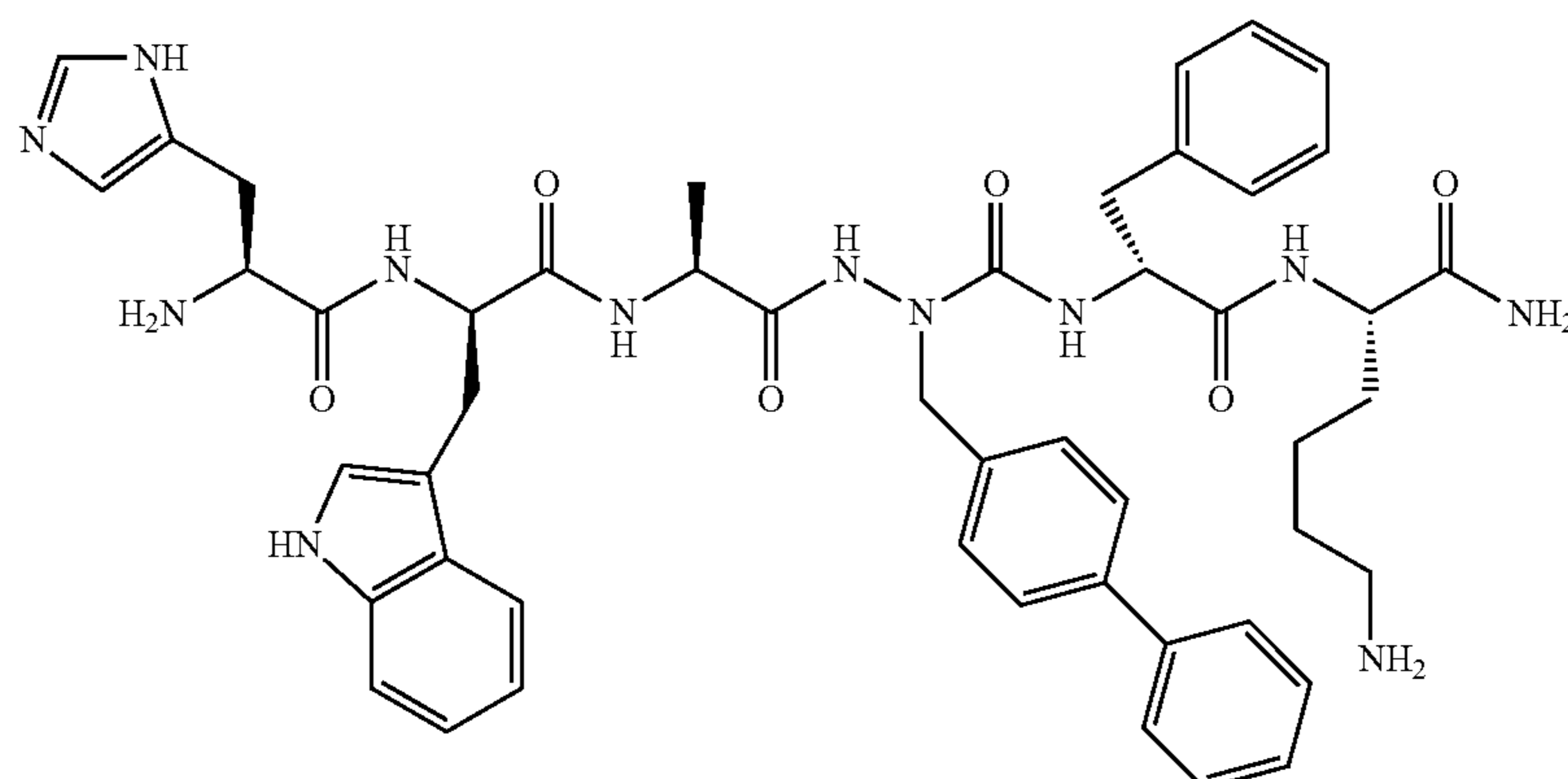
His-D-Trp-Ala-azaBip-D-Phe-Lys-NH 2
