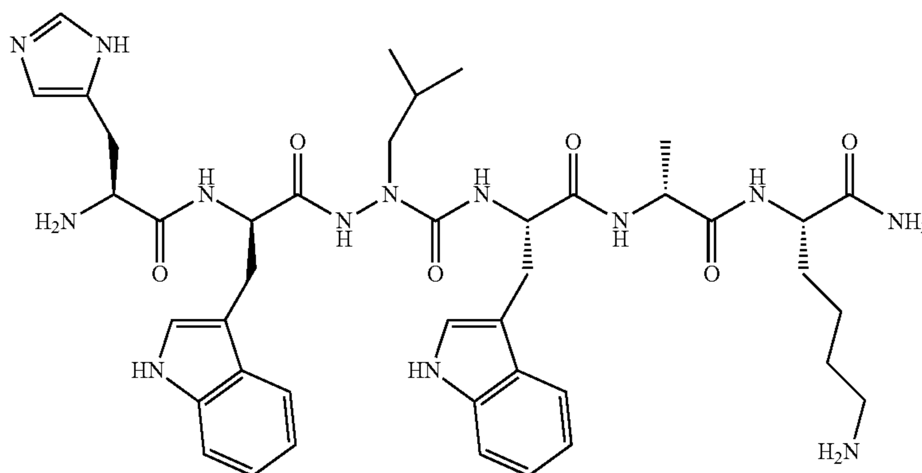
His-D-Trp-azaLeu-Trp-D-Ala-Lys-NH 2
