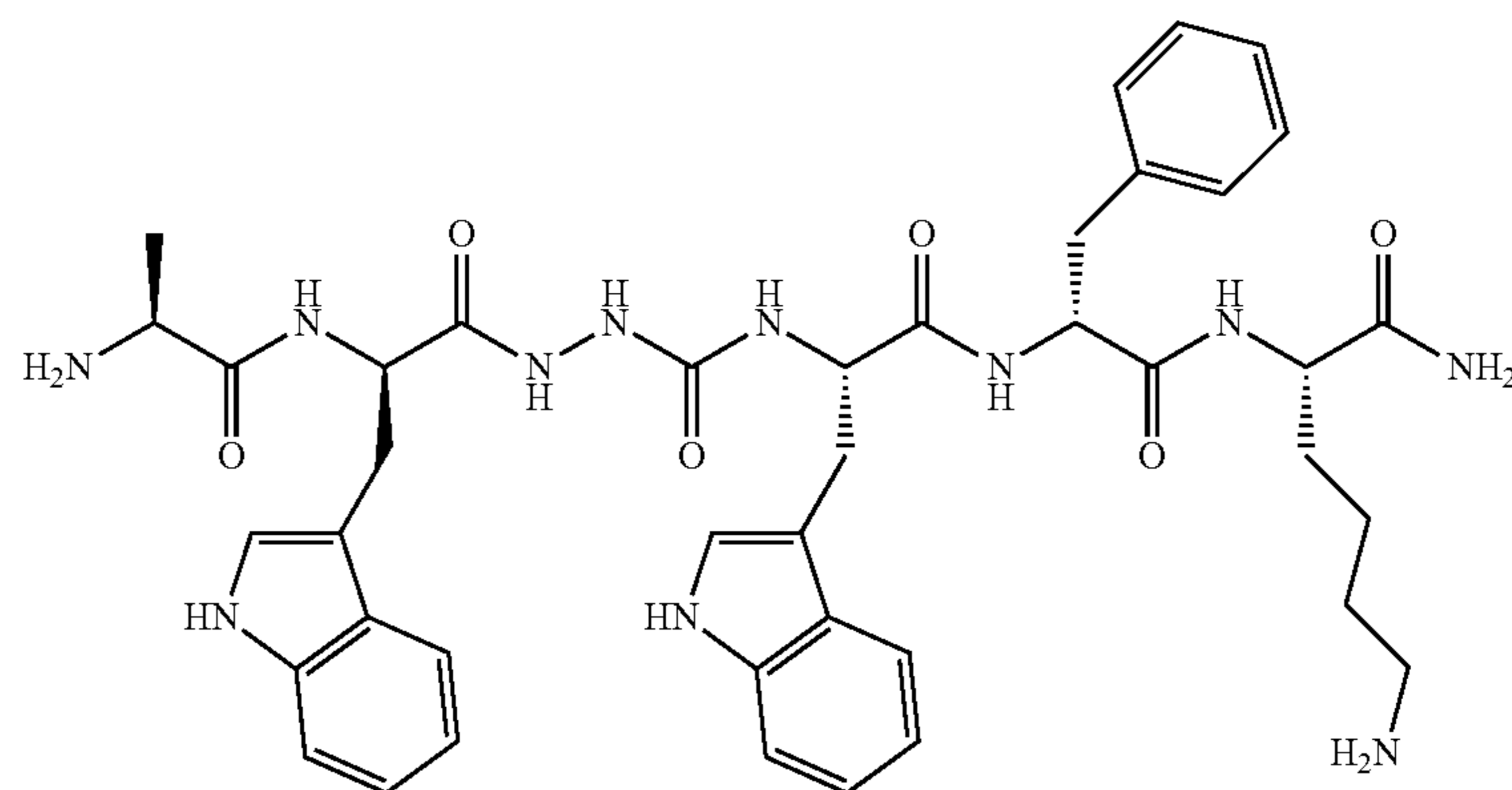
Ala-D-Trp-azaGly-Trp-D-Phe-Lys-NH 2
