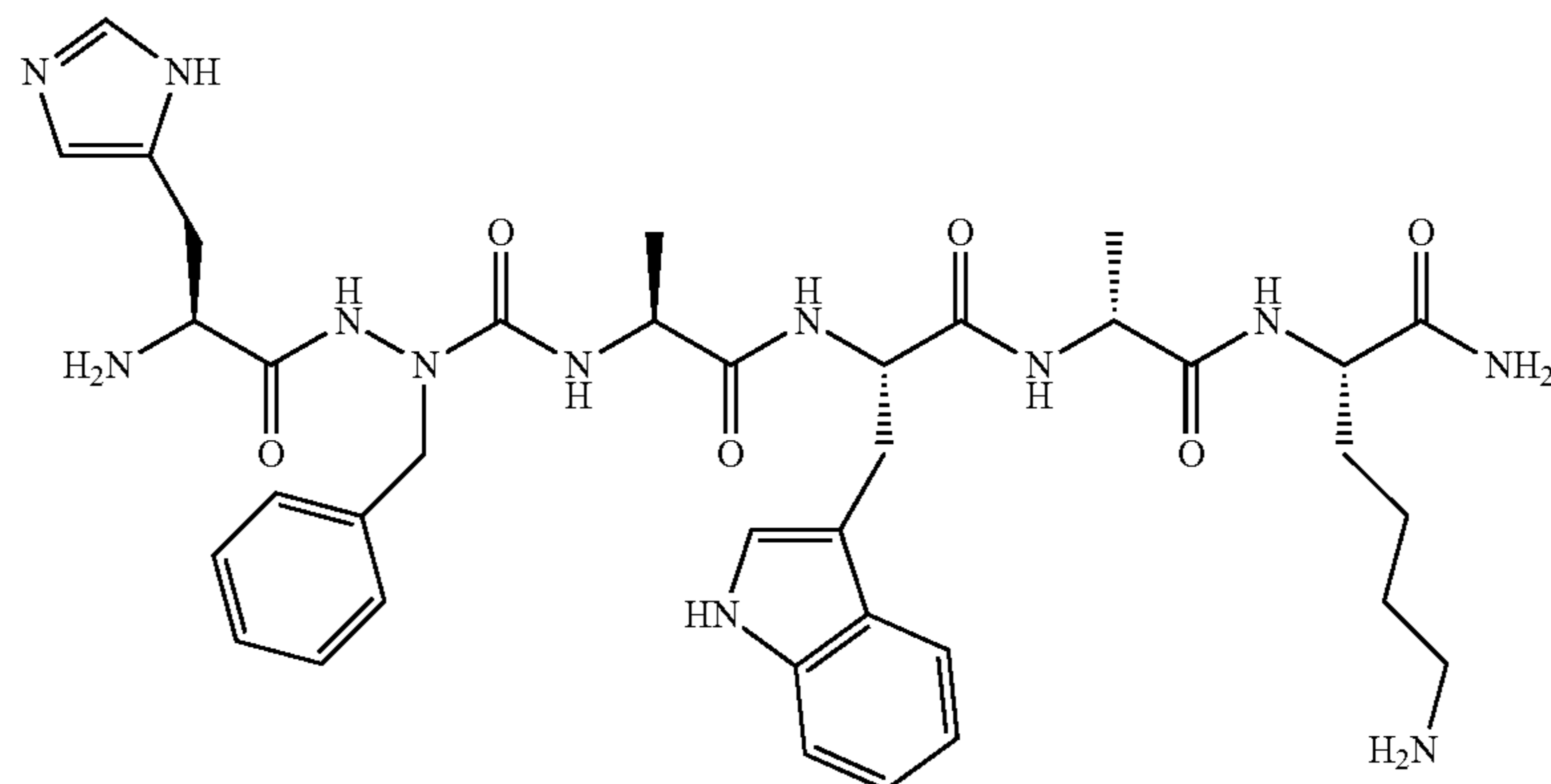
His-azaPhe-Ala-Trp-D-Ala-Lys-NH 2
