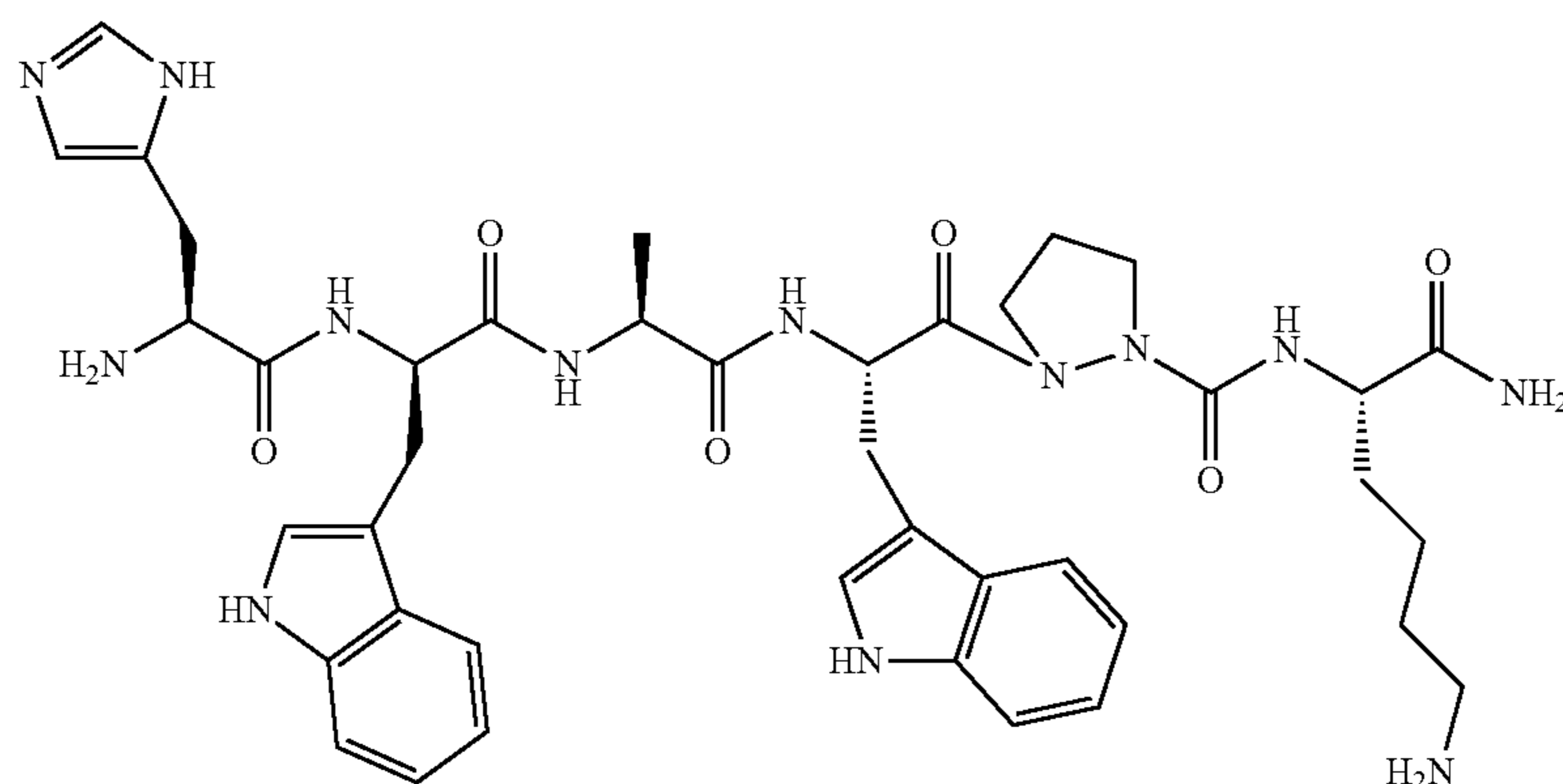
His-D-Trp-Ala-Trp-azaPro-Lys-NH 2
