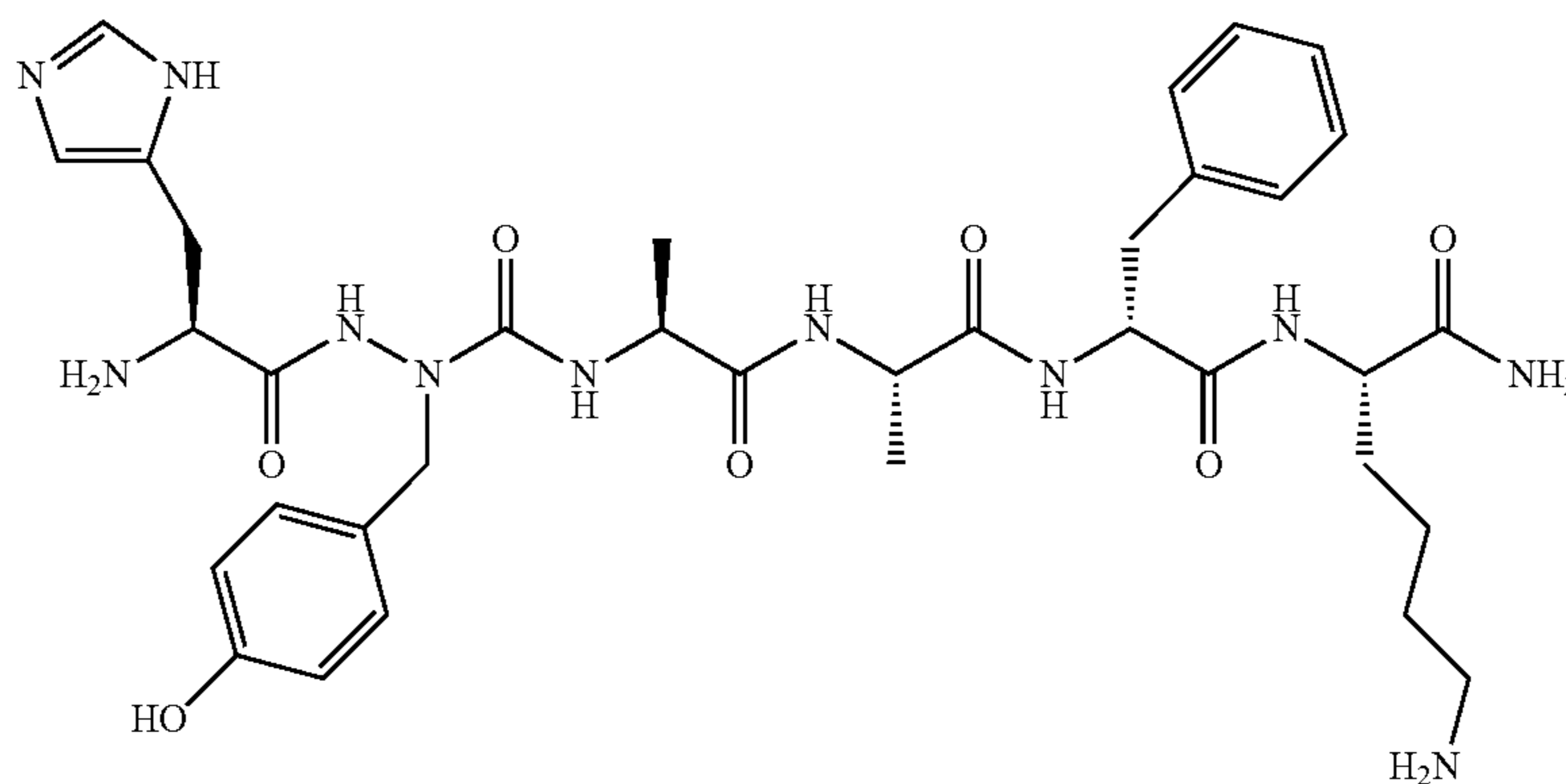
(D/L)His-azaTyr-Ala-Ala-D-Phe-Lys-NH 2
