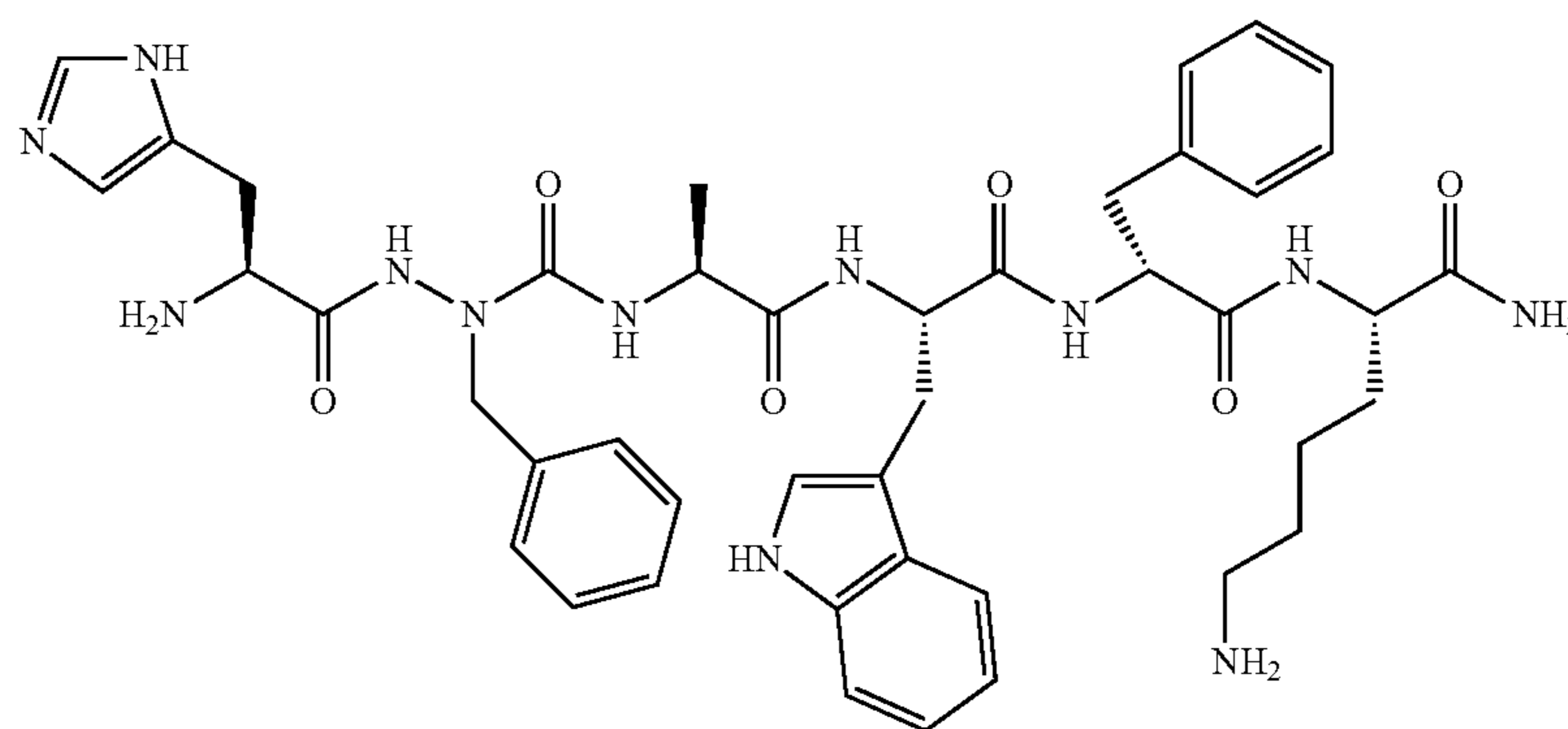
His-azaPhe-Ala-Trp-D-Phe-Lys-NH 2
