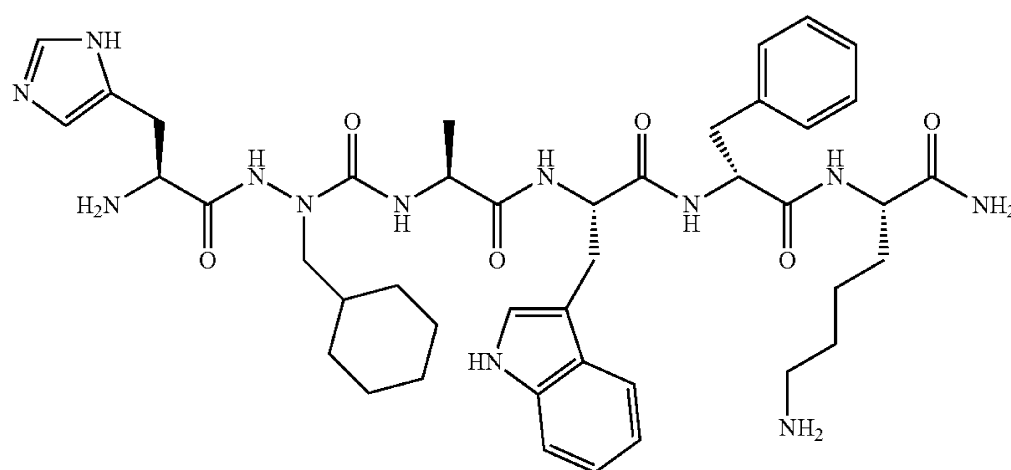
His-azaCha-Ala-Trp-D-Phe-Lys-NH 2
