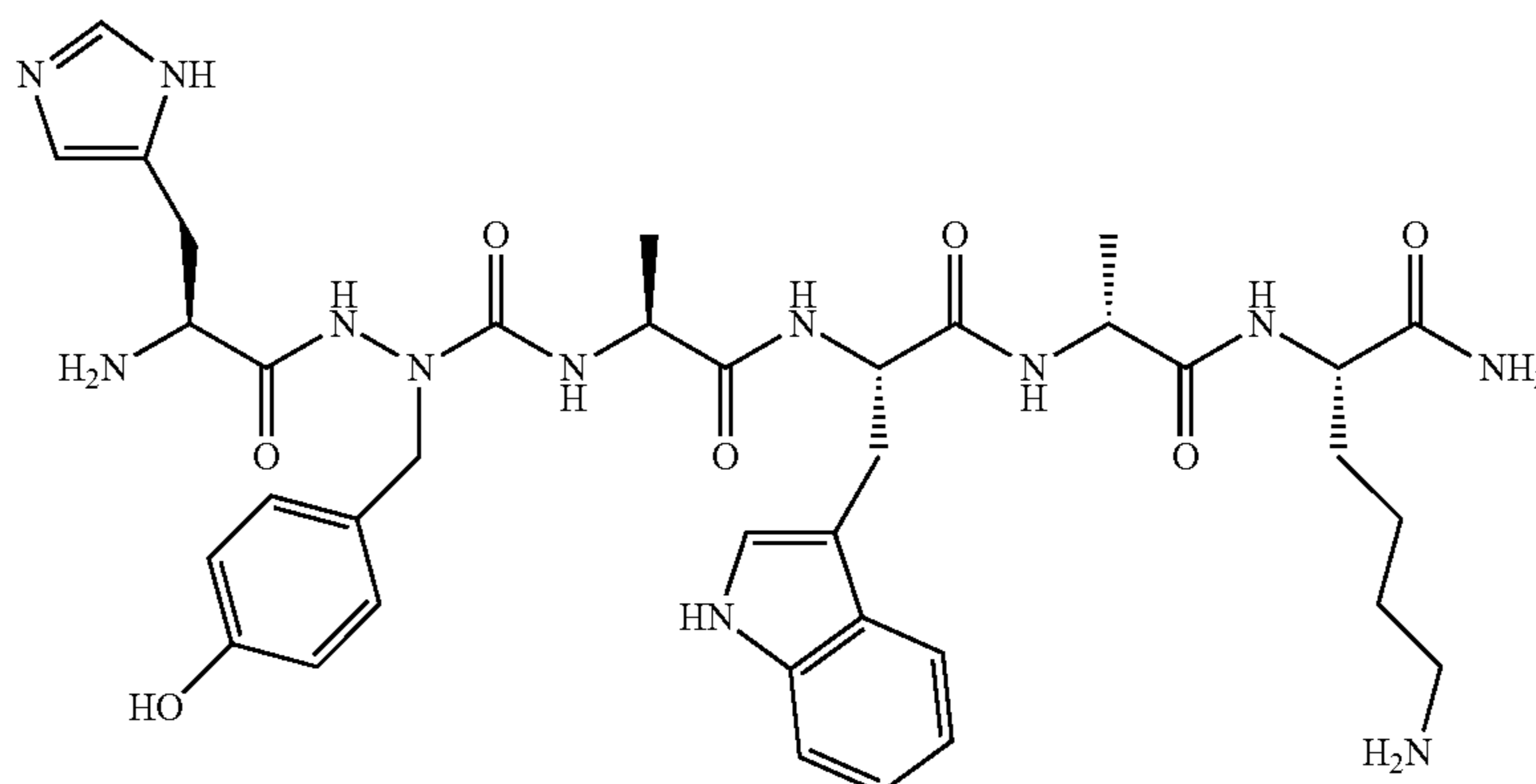
His-azaTyr-Ala-Trp-D-Ala-Lys-NH 2
