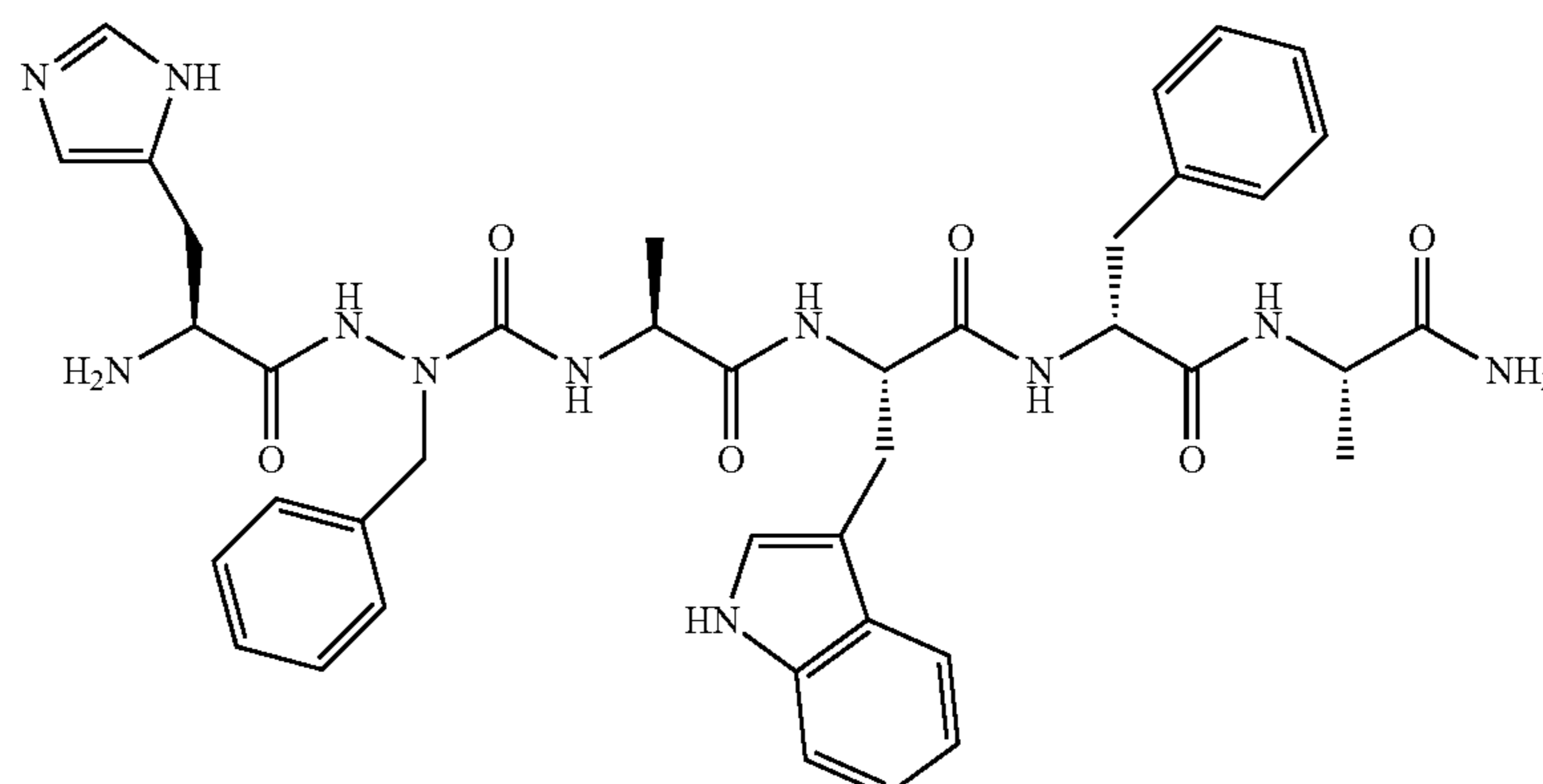
His-azaPhe-Ala-Trp-D-Phe-Ala-NH 2
