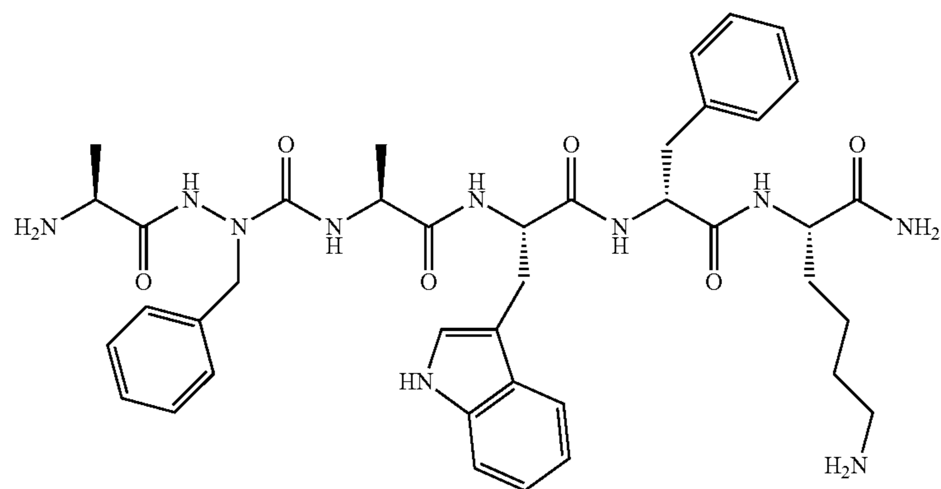
Ala-azaPhe-Ala-Trp-D-Phe-Lys-NH 2
