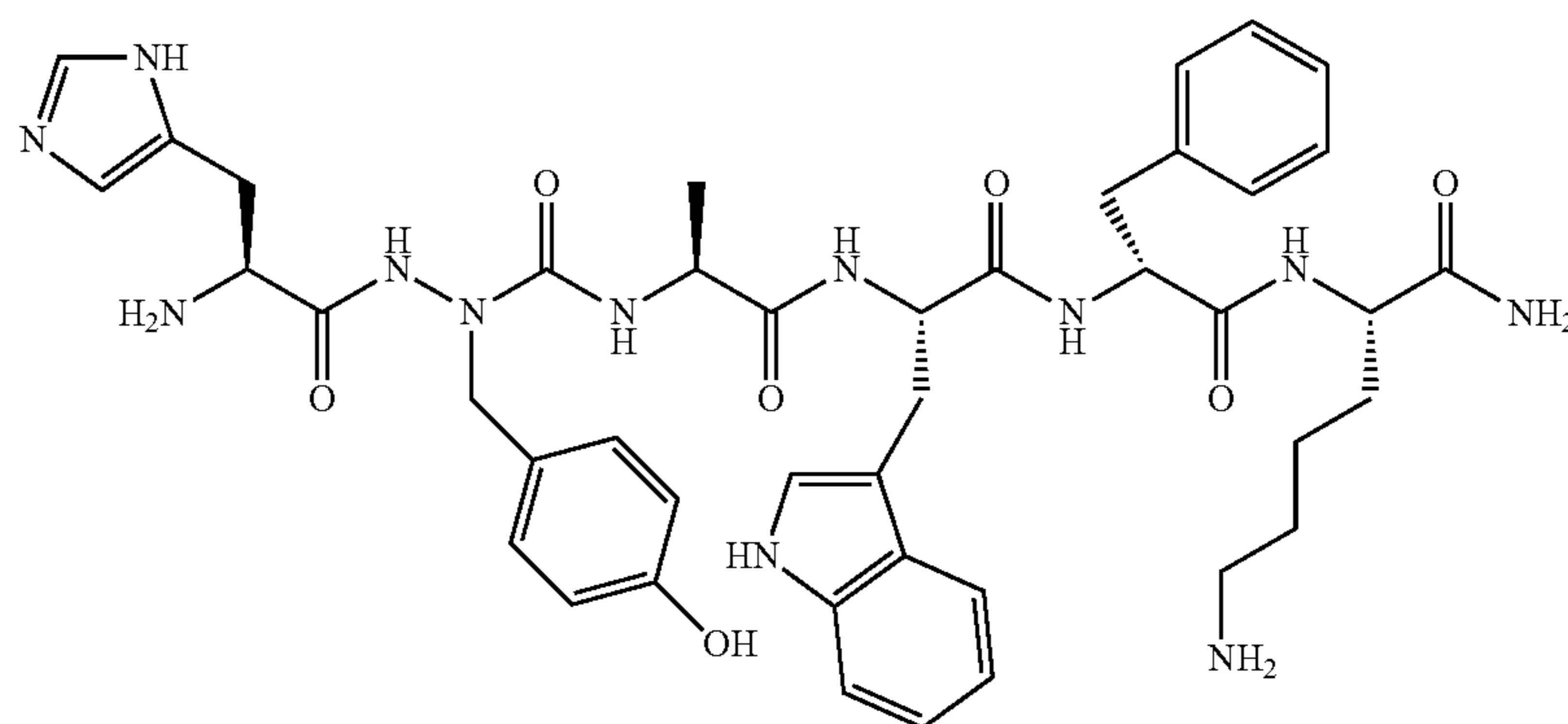
His-azaTyr-Ala-Trp-D-Phe-Lys-NH 2
