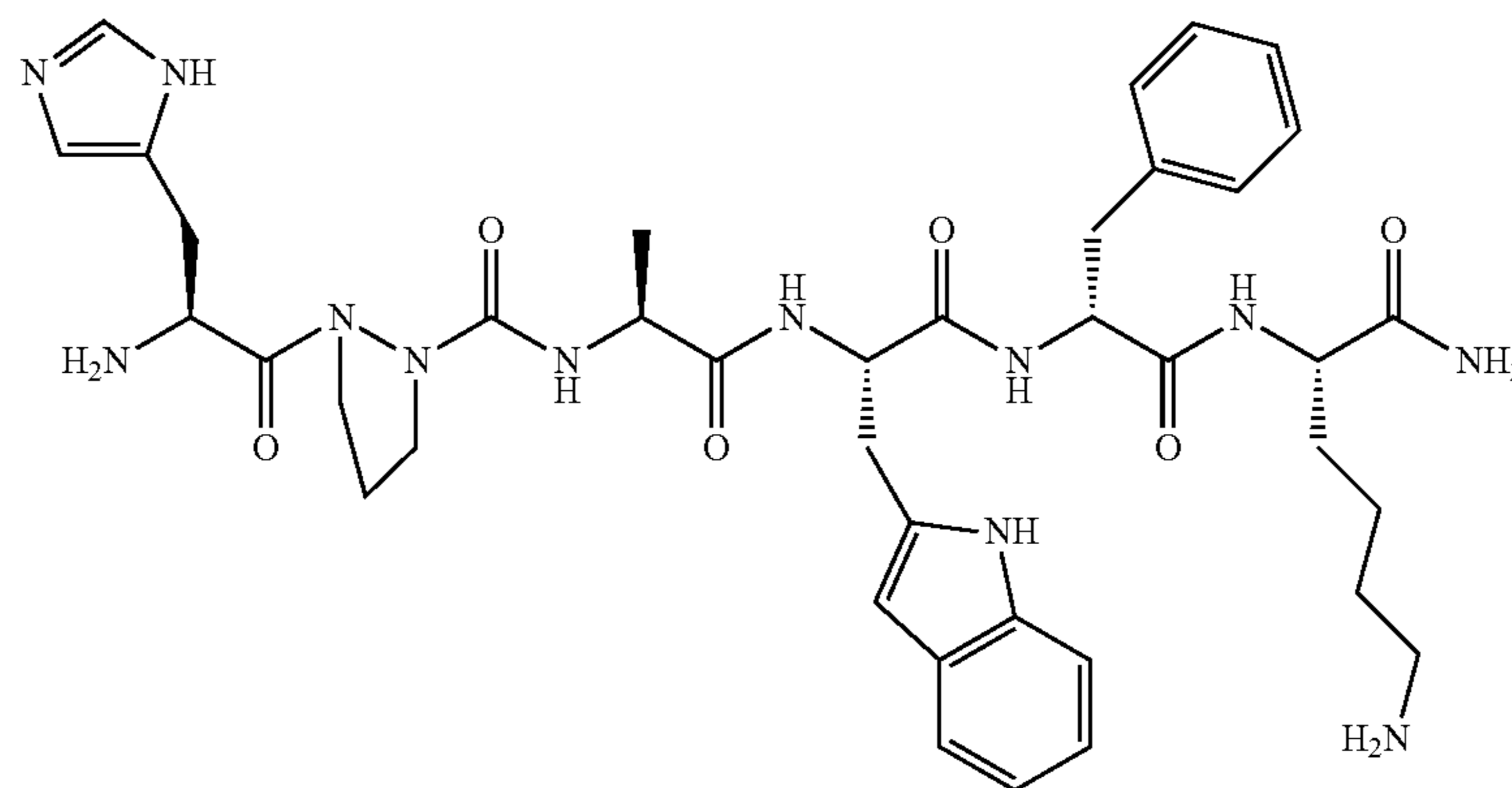
His-azaPro-Ala-Trp-D-Phe-Lys-NH 2
