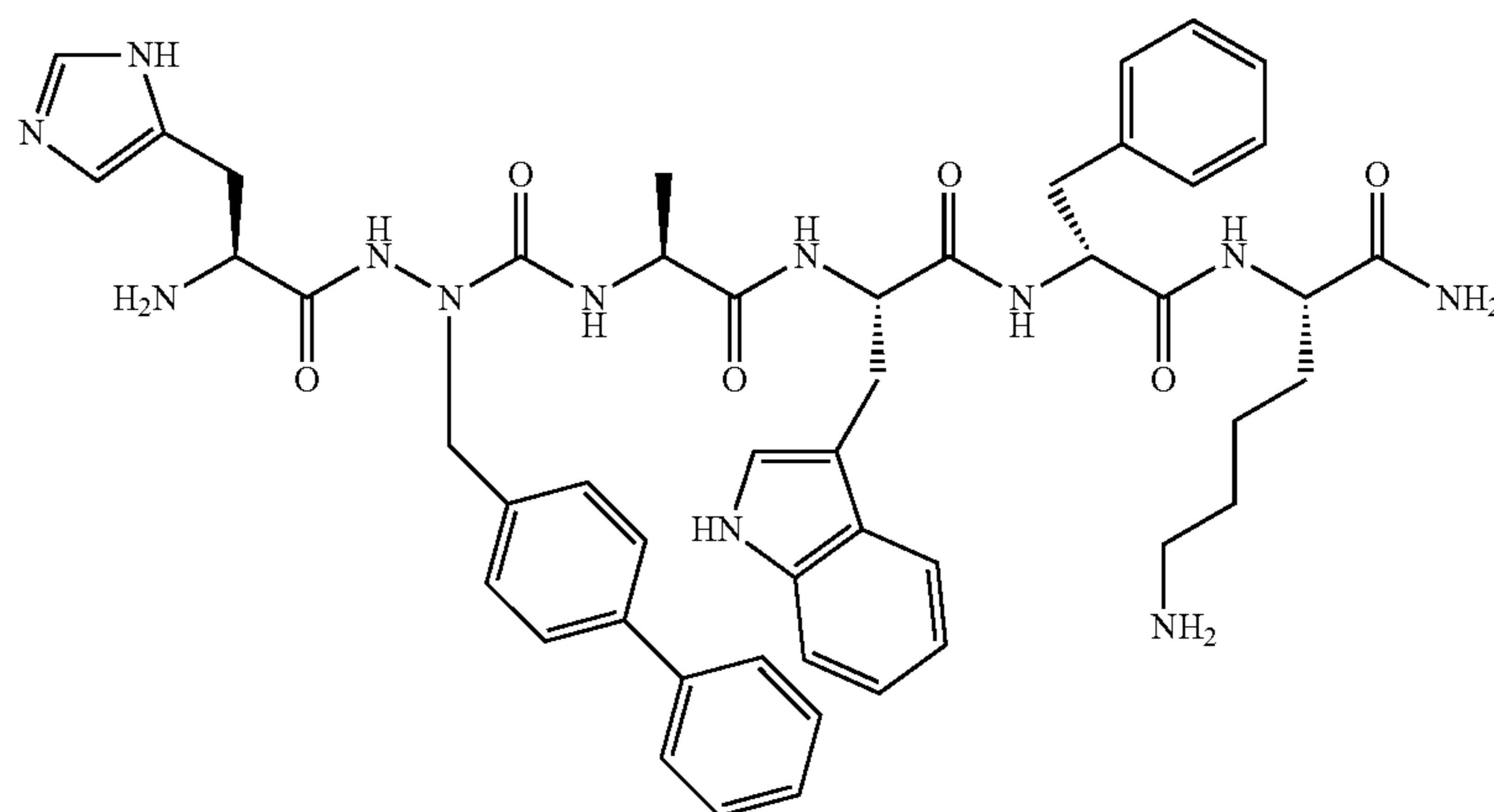
His-azaBip-Ala-Trp-D-Phe-Lys-NH 2
