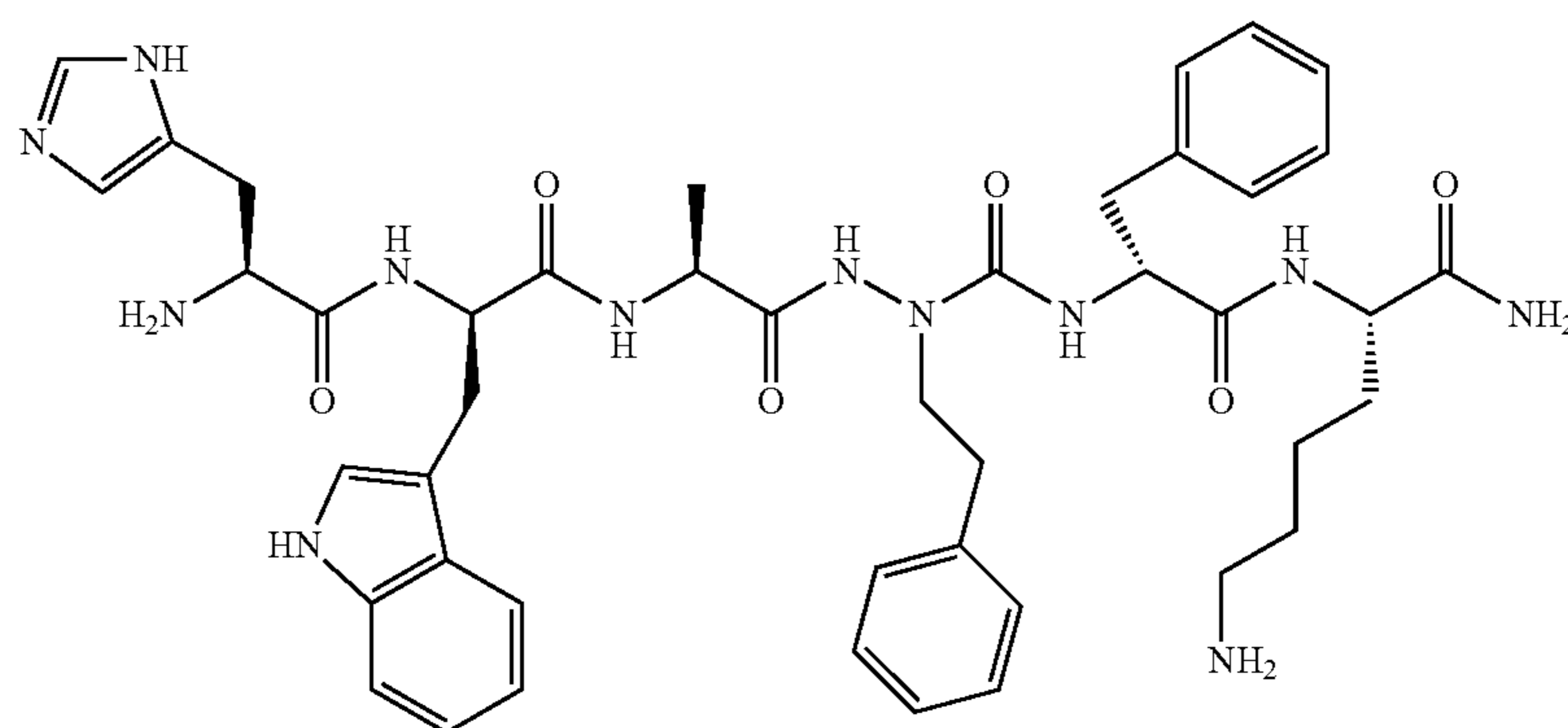
His-D-Trp-Ala-azahomoPhe-D-Phe-Lys-NH 2
