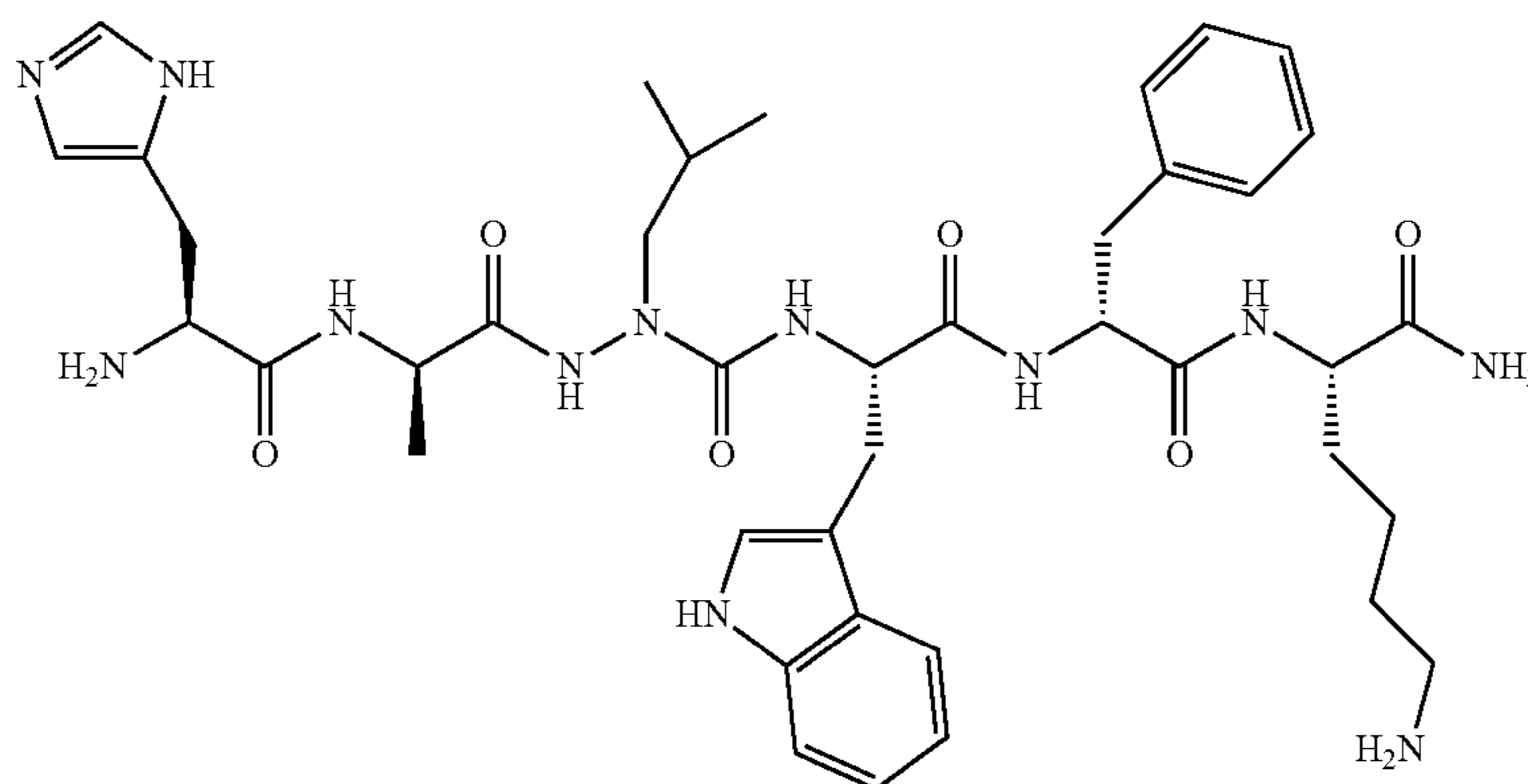
His-D-Ala-azaLeu-Trp-D-Phe-Lys-NH 2
