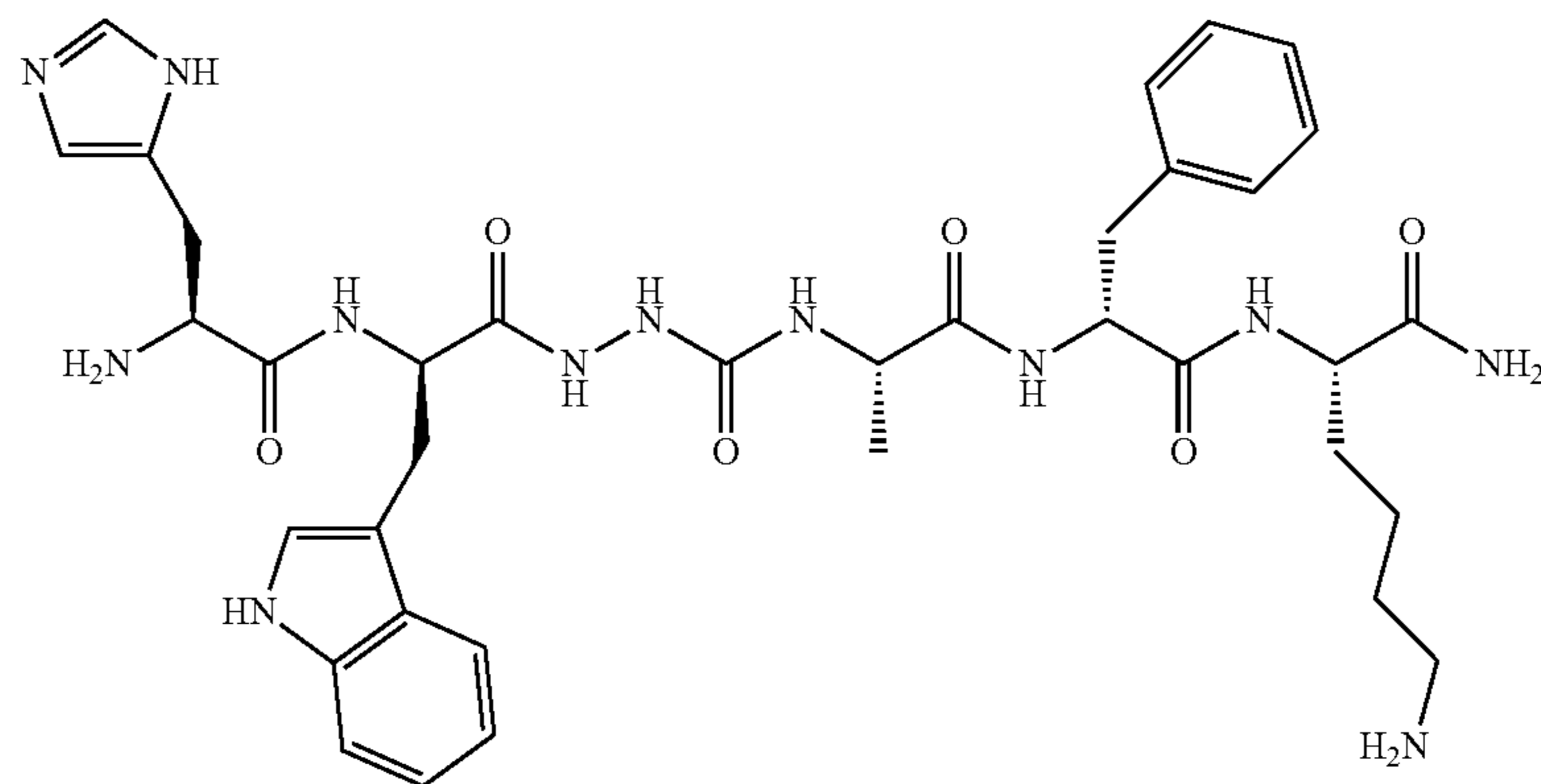
His-D-Trp-azaGly-Ala-D-Phe-Lys-NH 2
