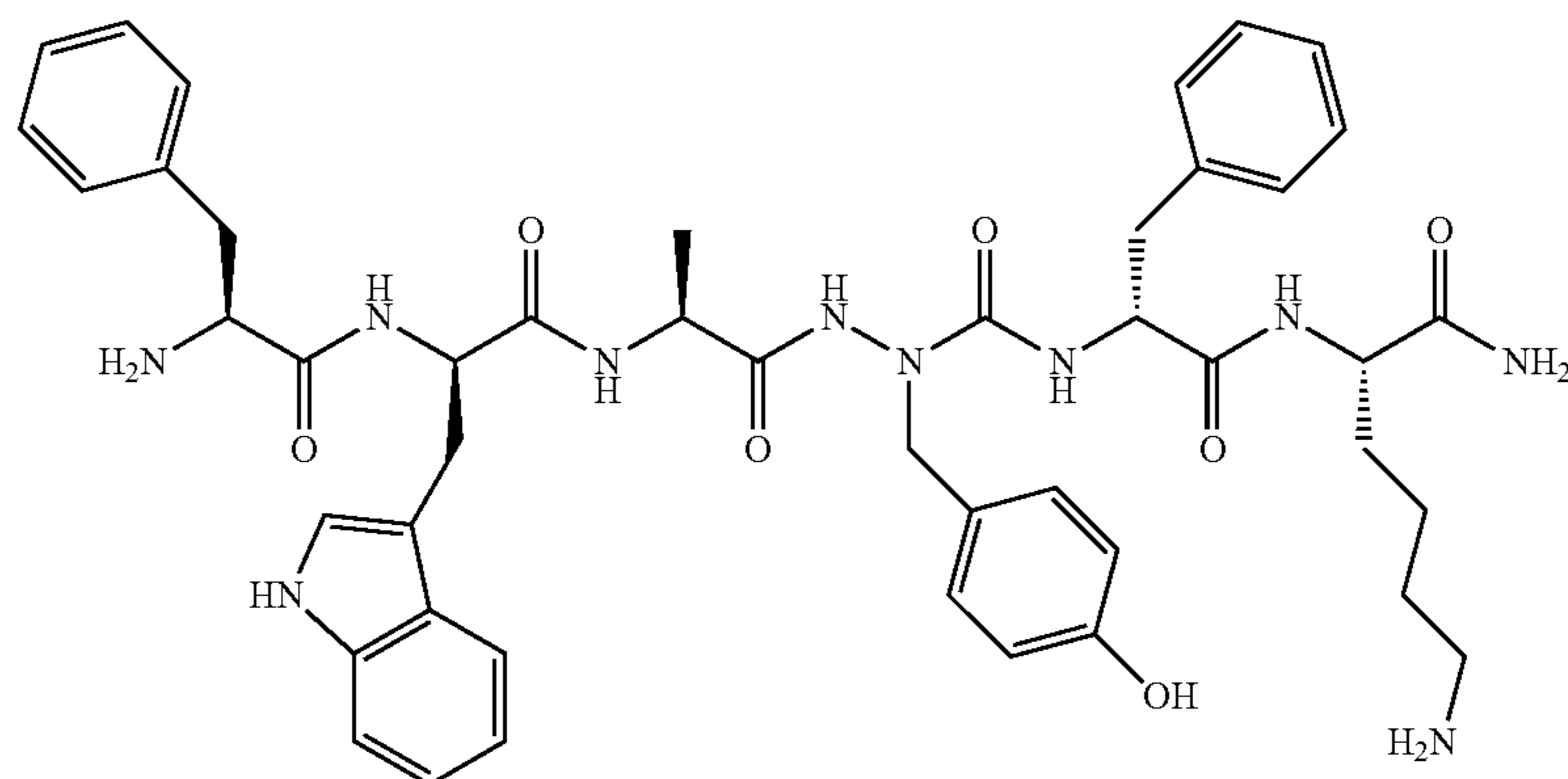
Phe-D-Trp-Ala-AzaTyr-D-Phe-Lys-NH 2
