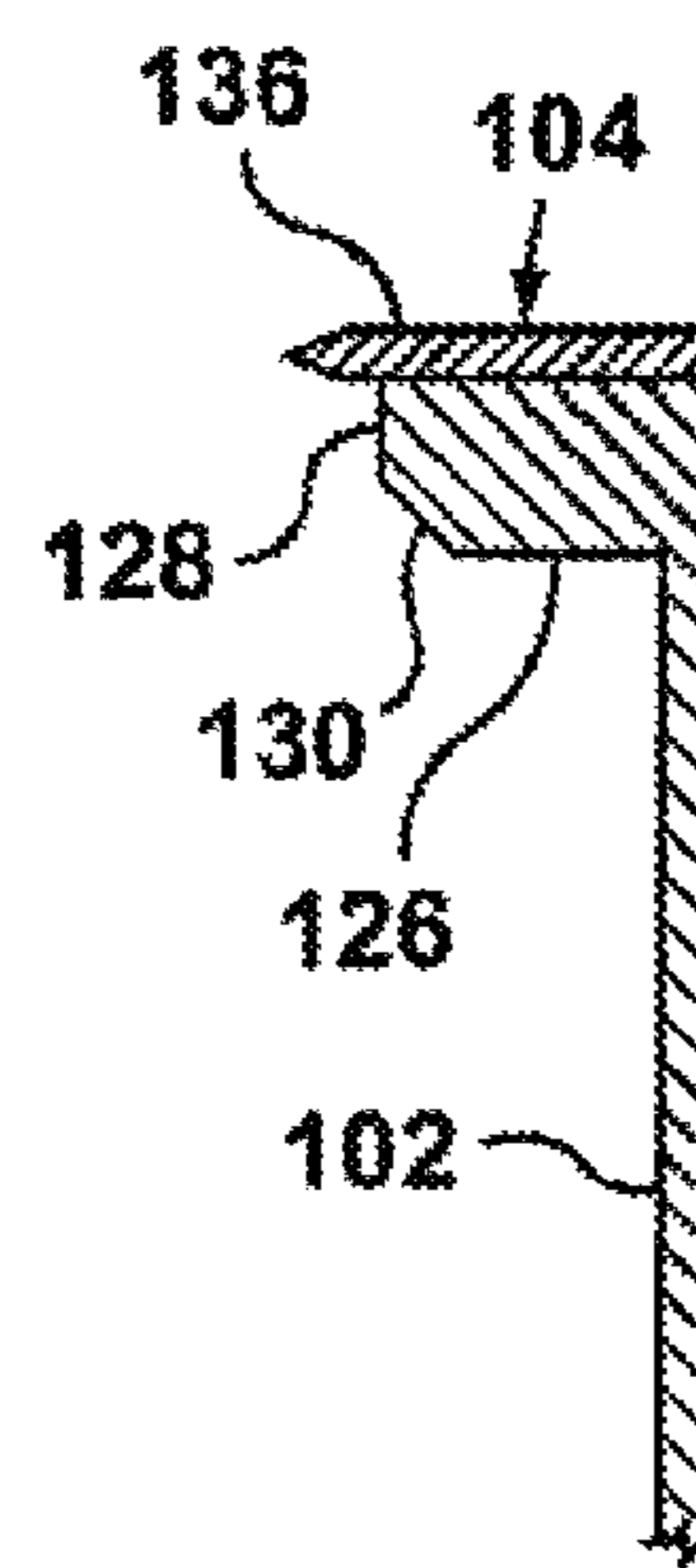
FIG. 10
