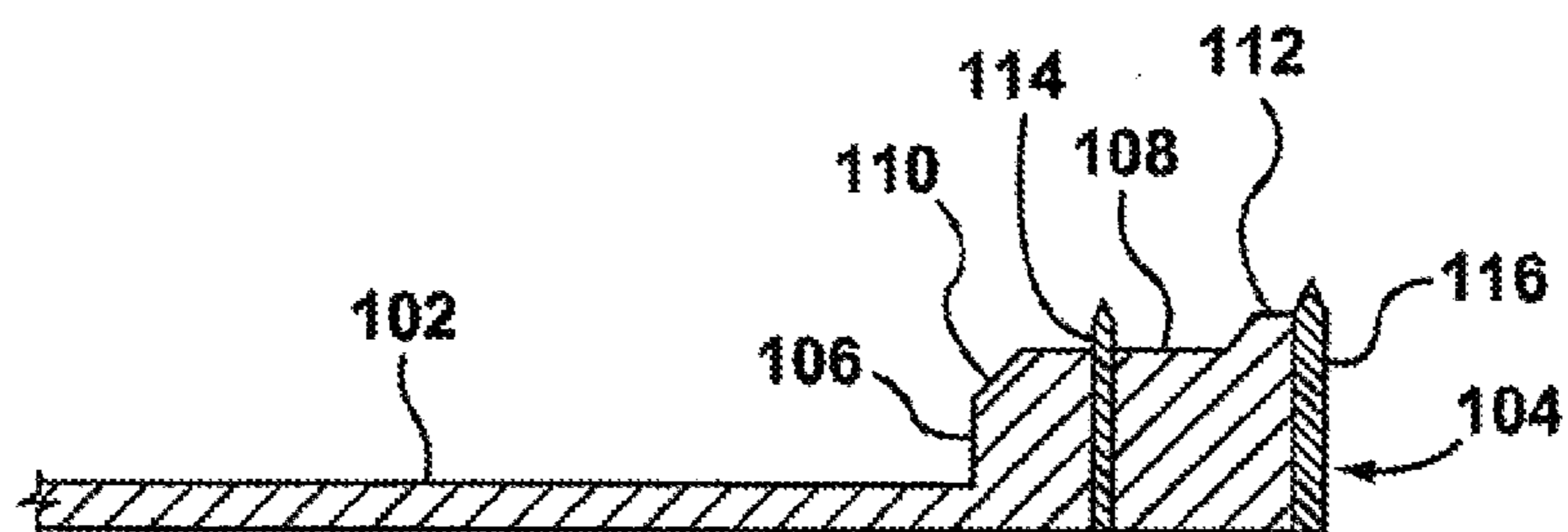
FIG. 8
