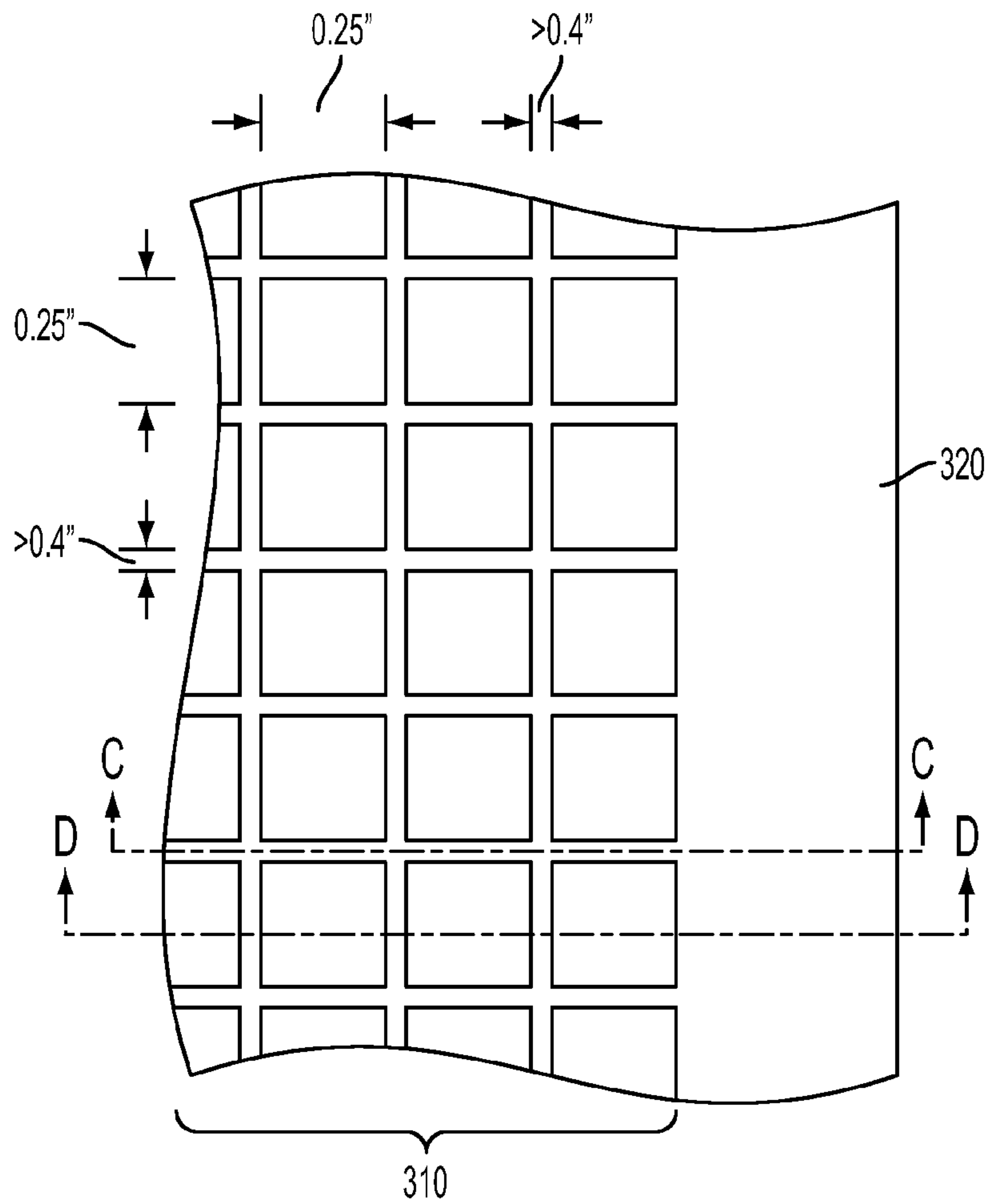
FIG. 3B
