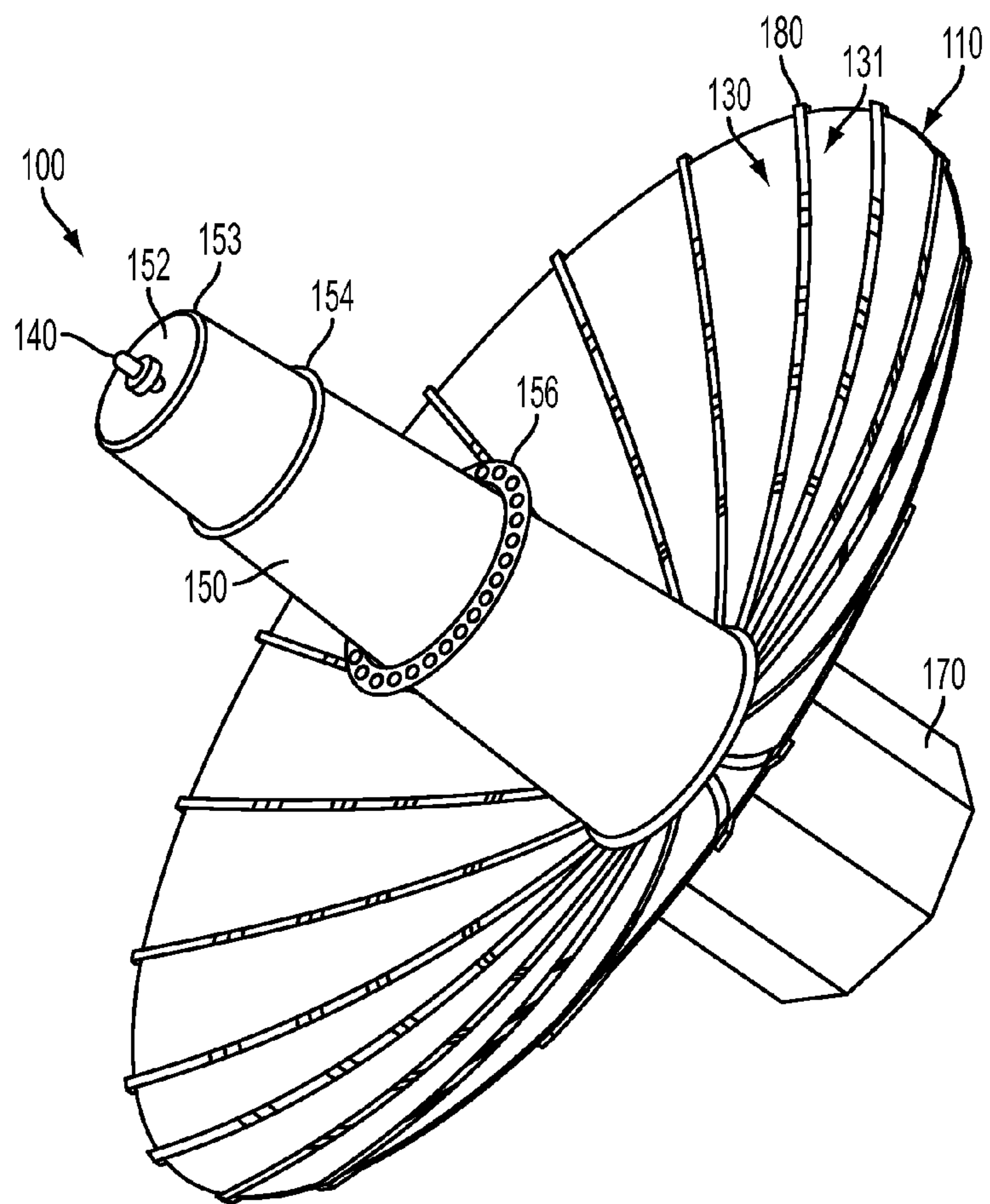
FIG. 1A
