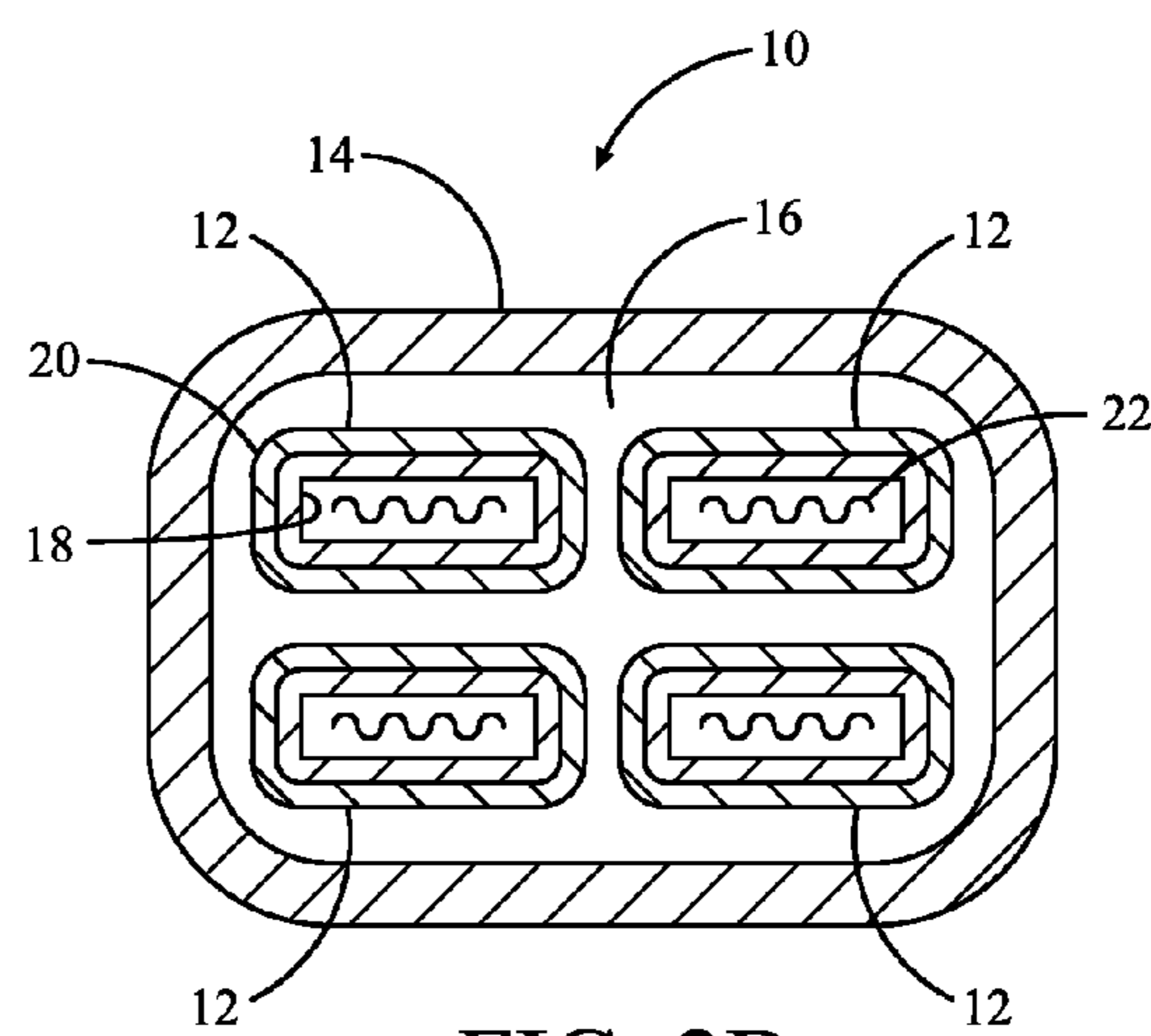
FIG. 2B
