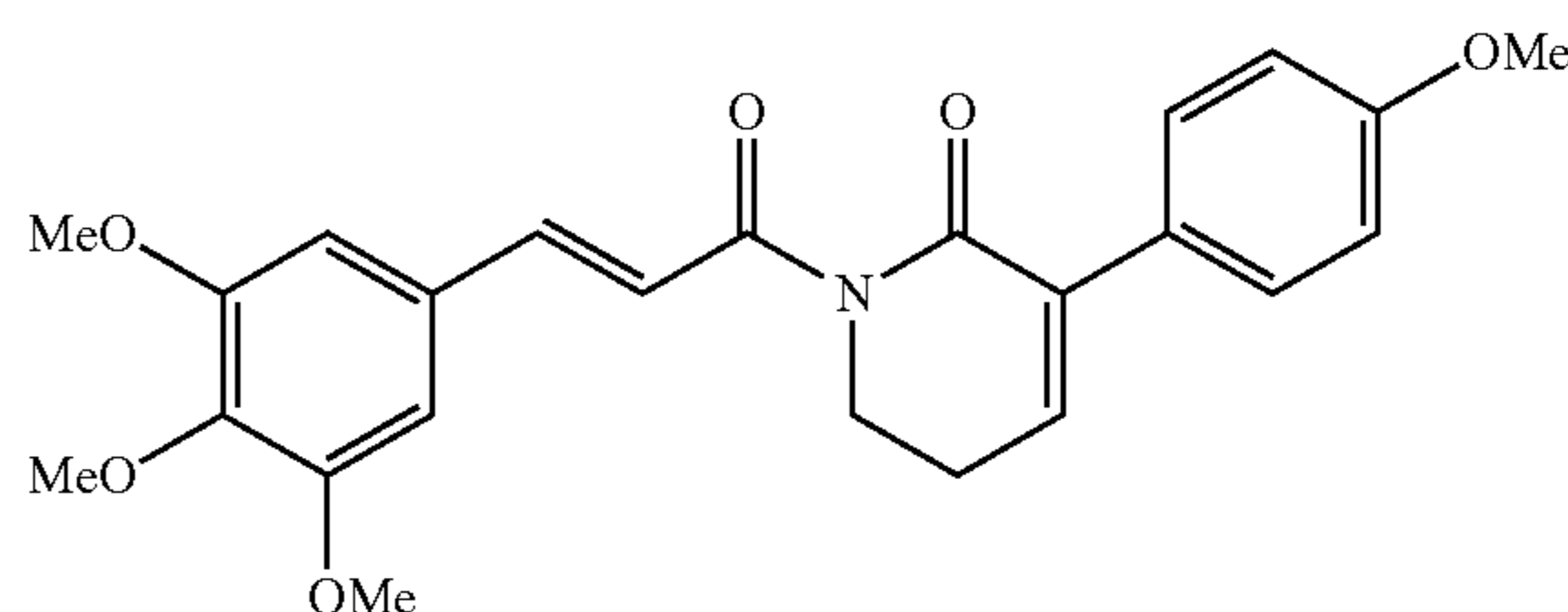
(E)-3-(4-methoxyphenyl)-1-(3-(3,4,5-trimethoxyphenyl)prop-2-enyl)-5,6-dihydropyridin-2(1H)-one
