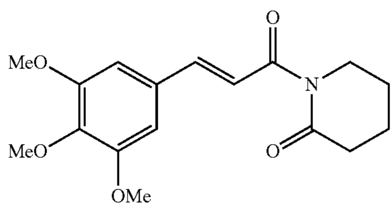
1-[(2E)-3-(3,4,5-trimethoxyphenyl)prop-2-enoyl] piperidin-2-one
