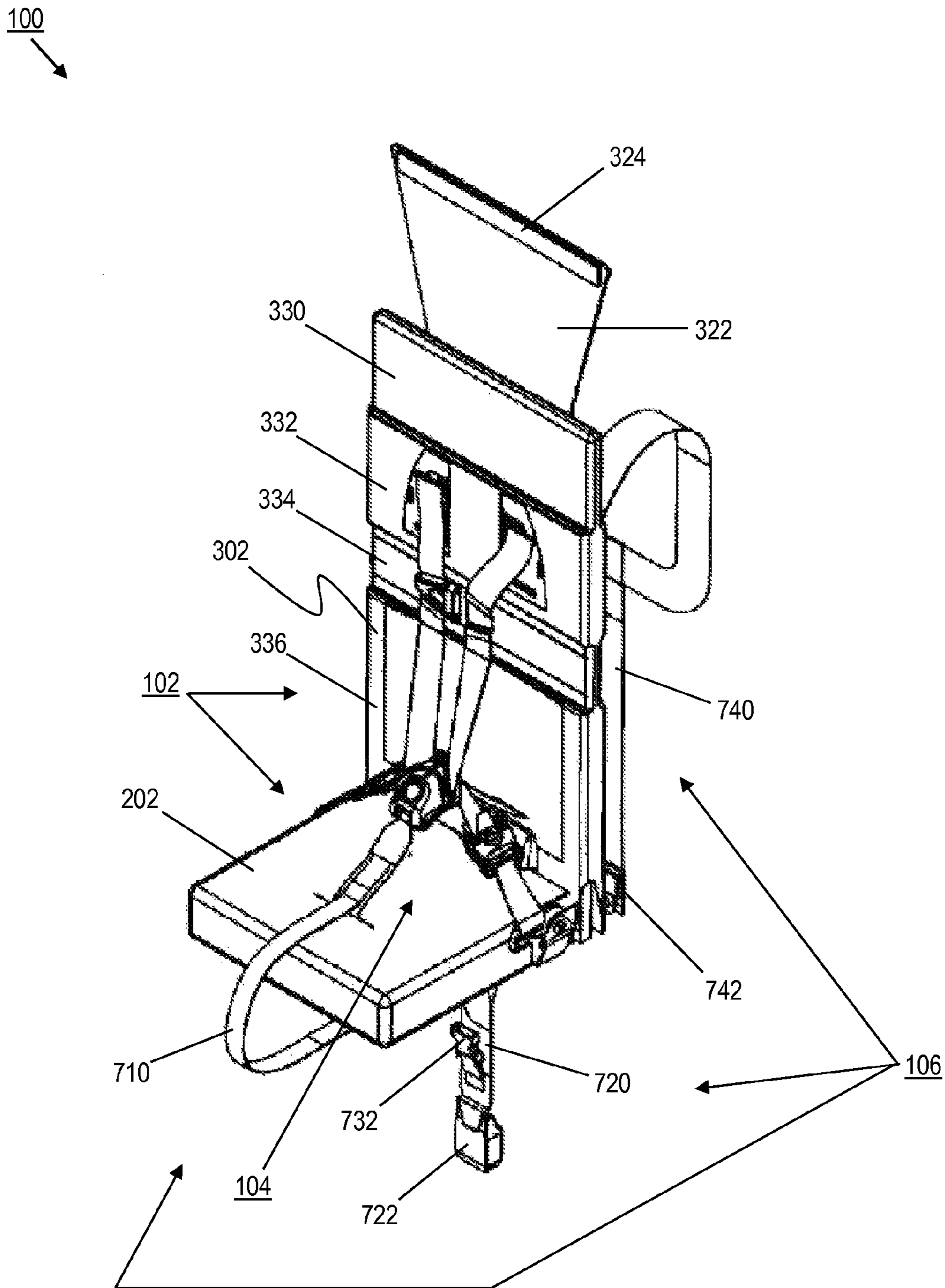
FIG. 1A
