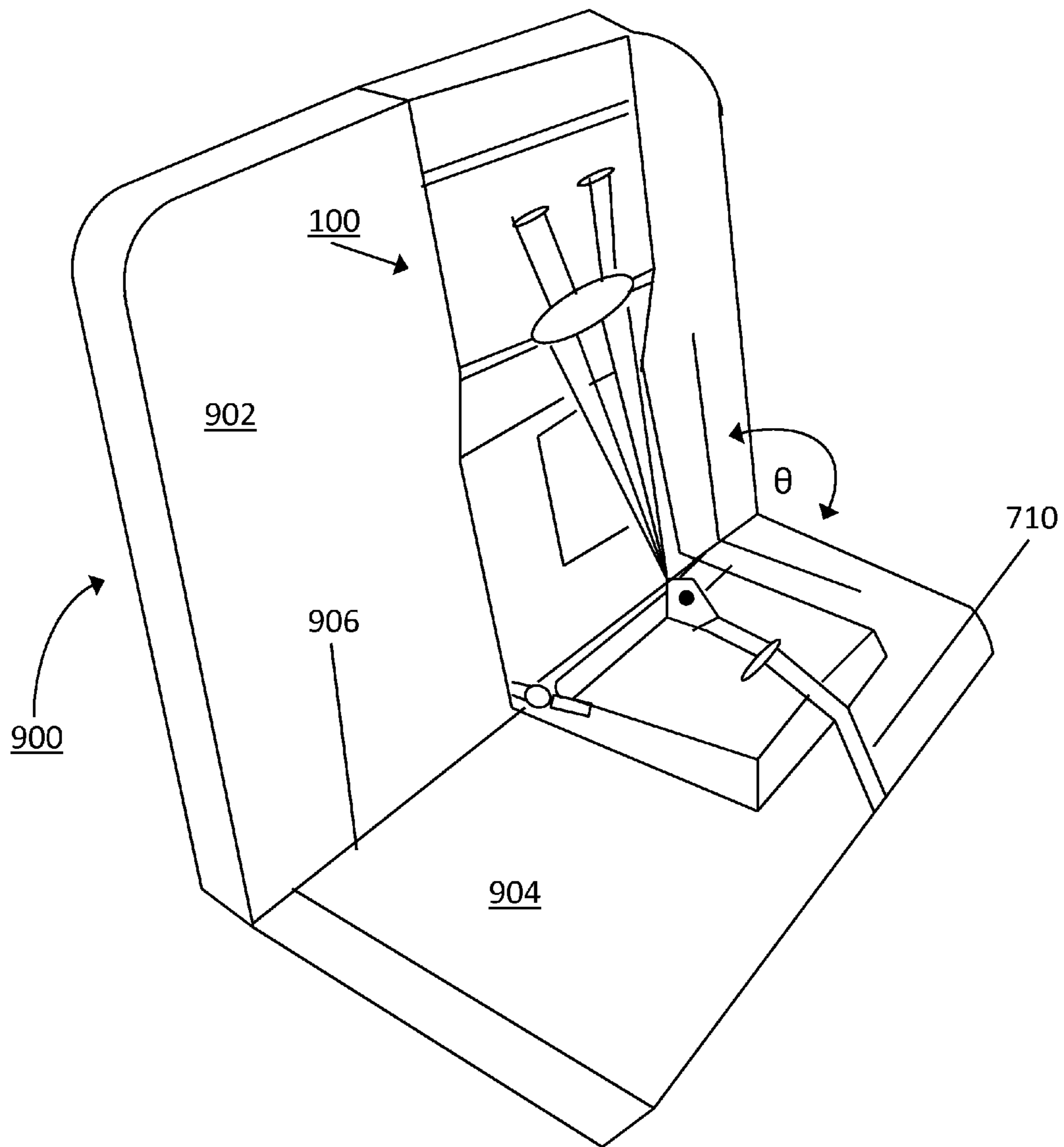
FIG. 20A
