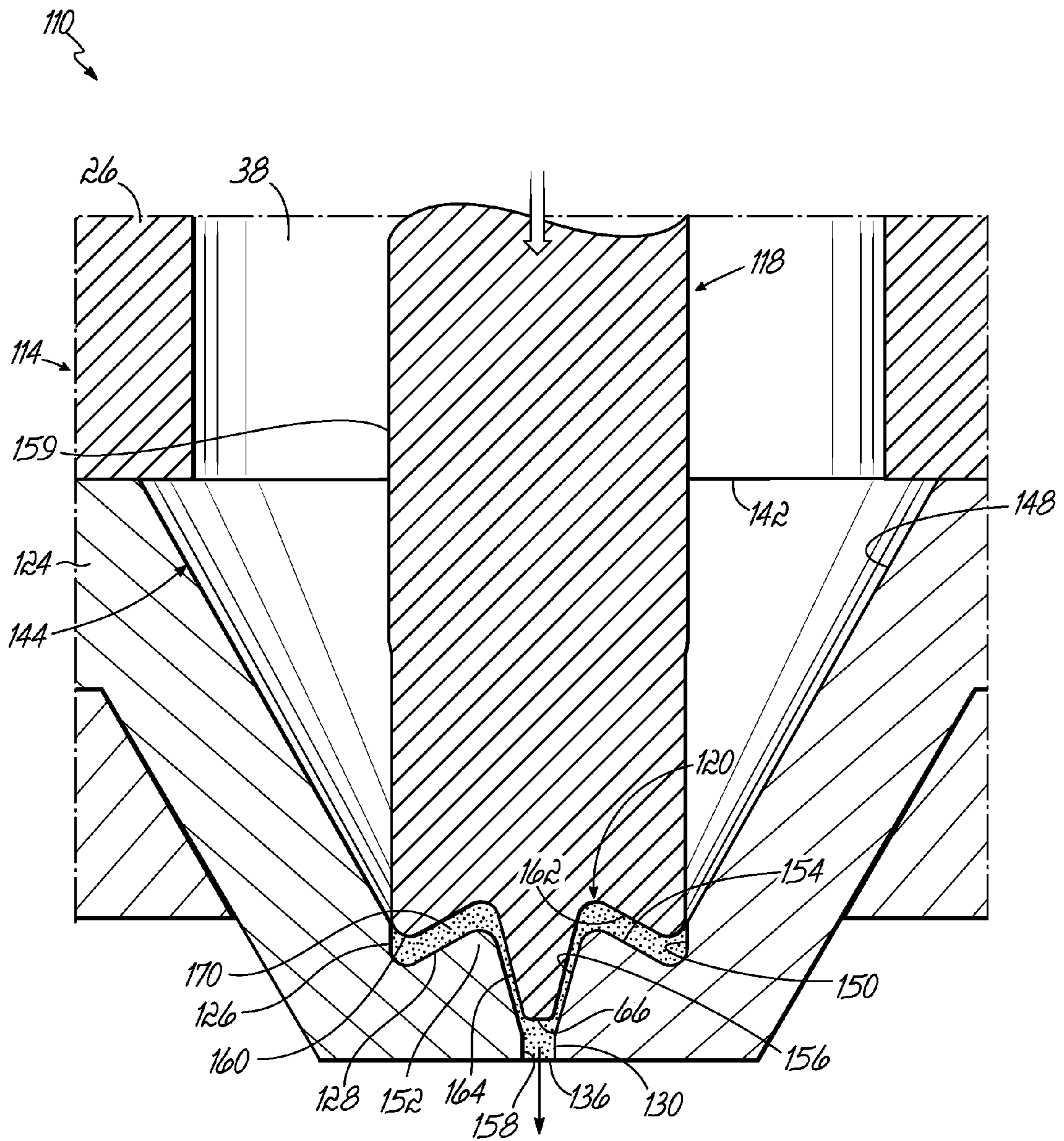
FIG. 3B
