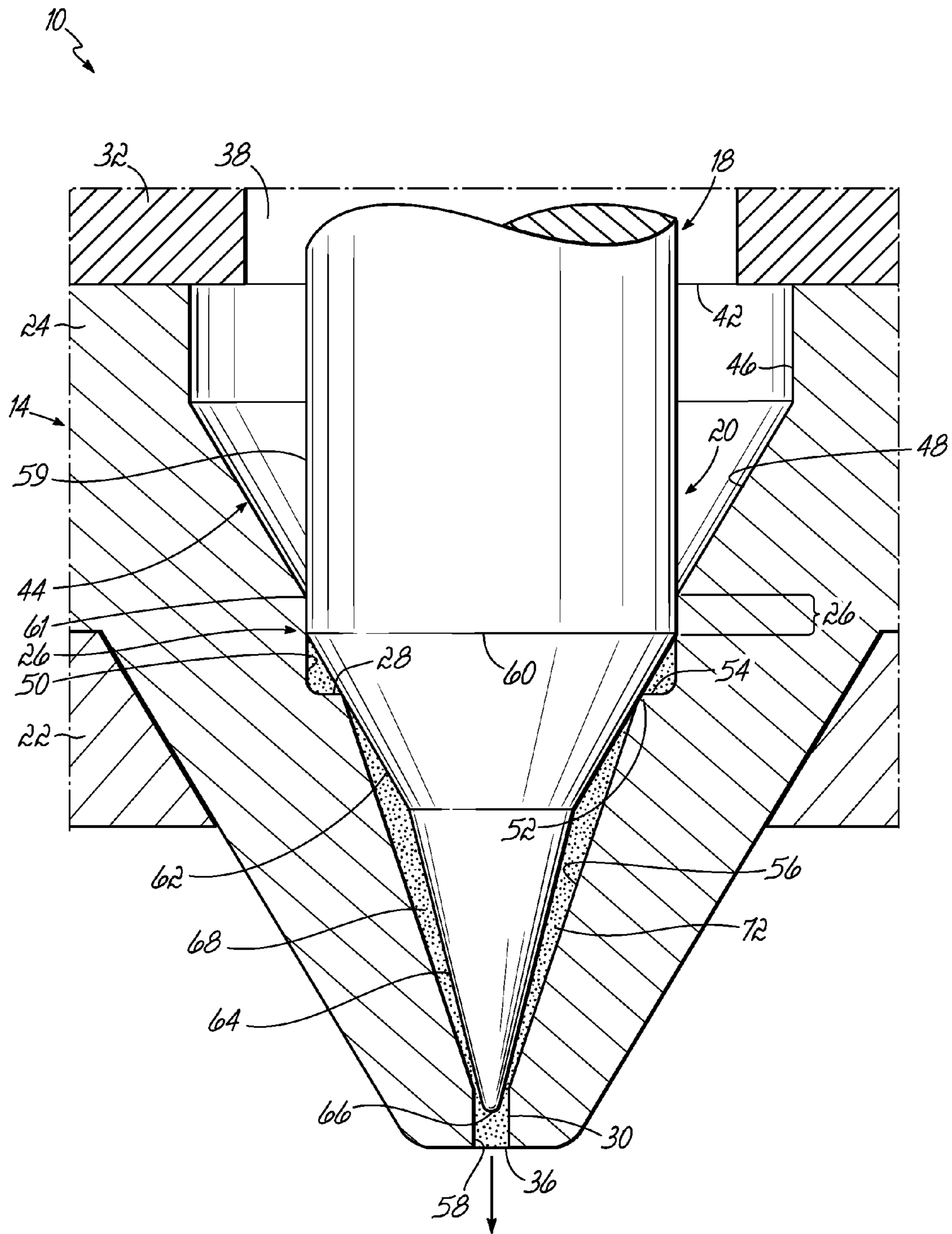
FIG. 2C
