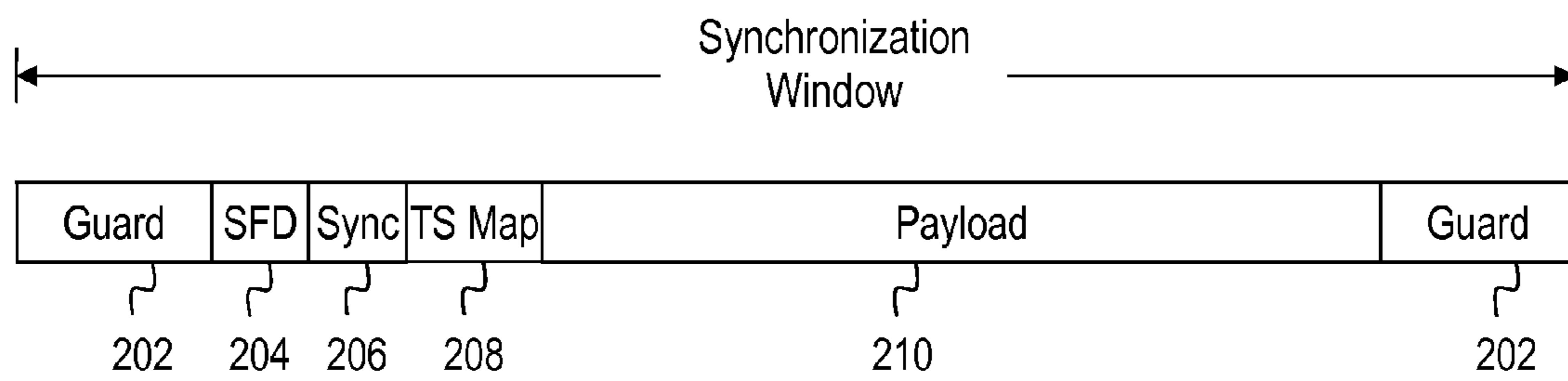
Fig. 2A
