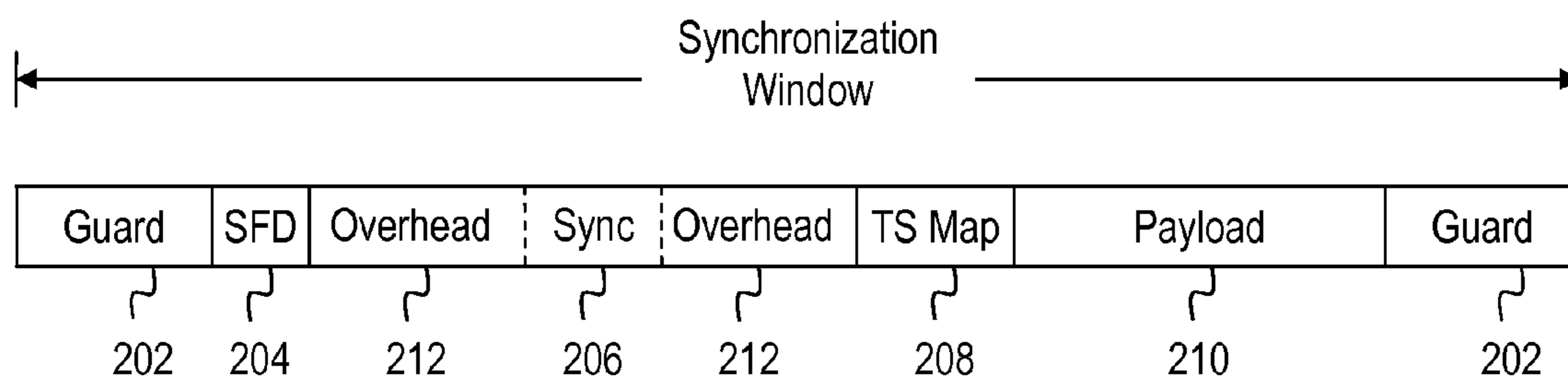
Fig. 2B
