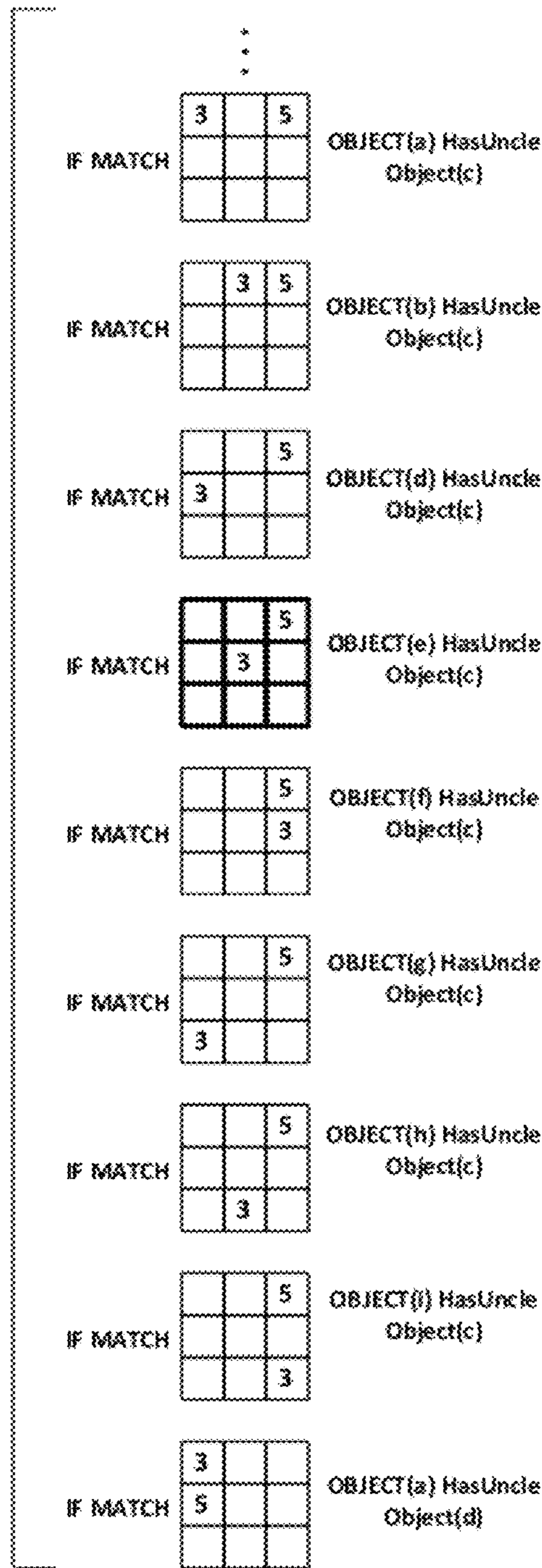
FIG. 26 – PREDICATE TEMPLATES
