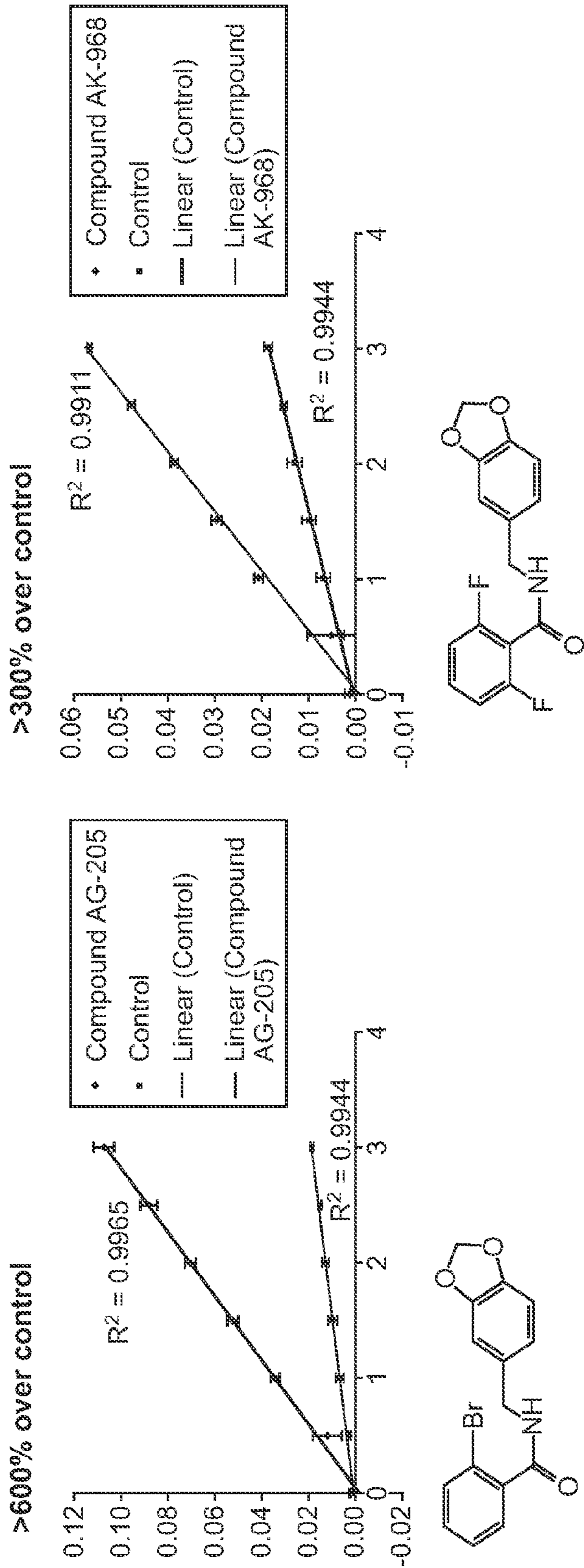
N-(1,3-benzodioxol-5-ylmethyl)-2-bromobenzamide N-(1,3-benzodioxol-5-ylmethyl)-2,6-difluorobenzamide
