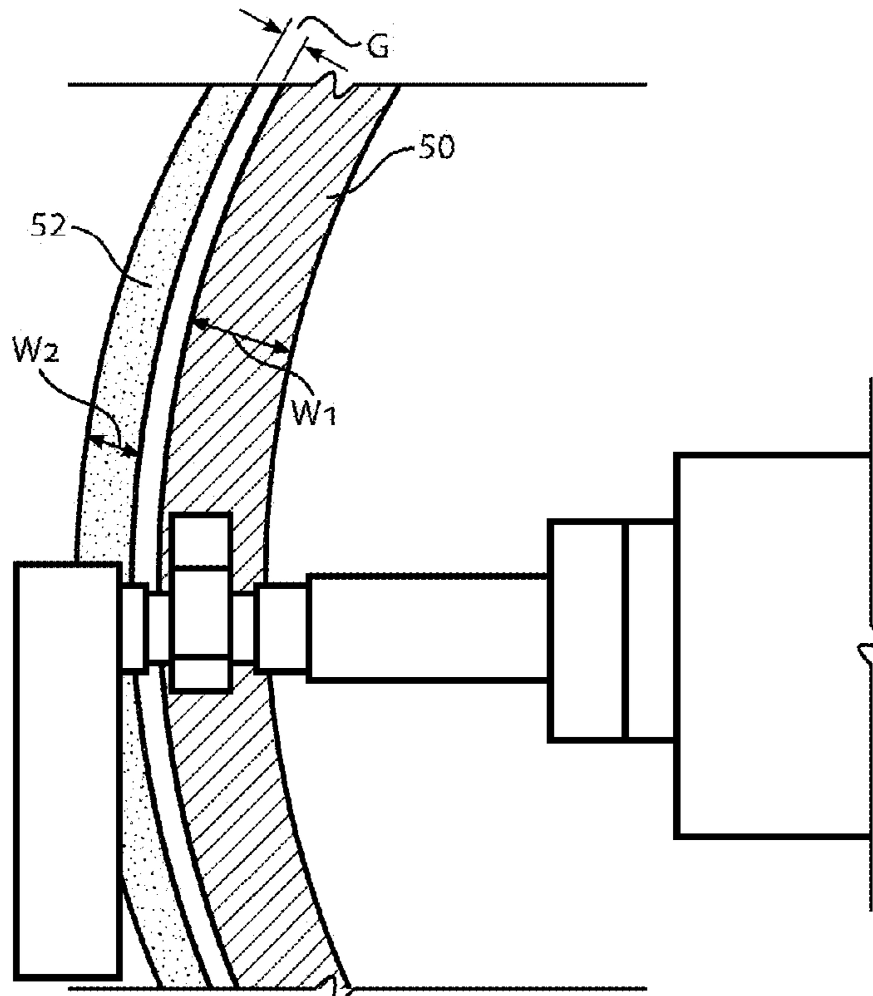
FIG. 1A
