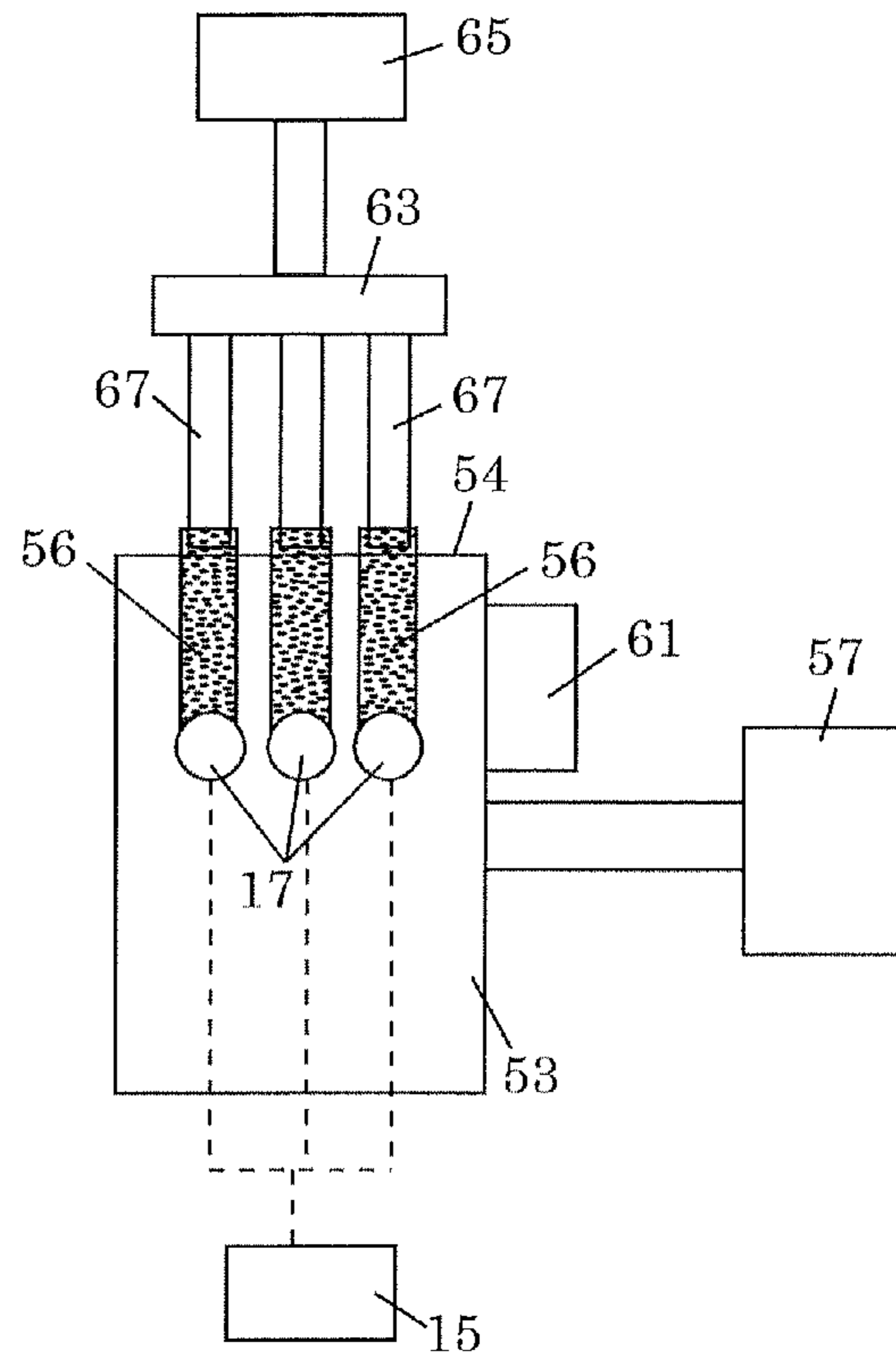
FIG. 9
