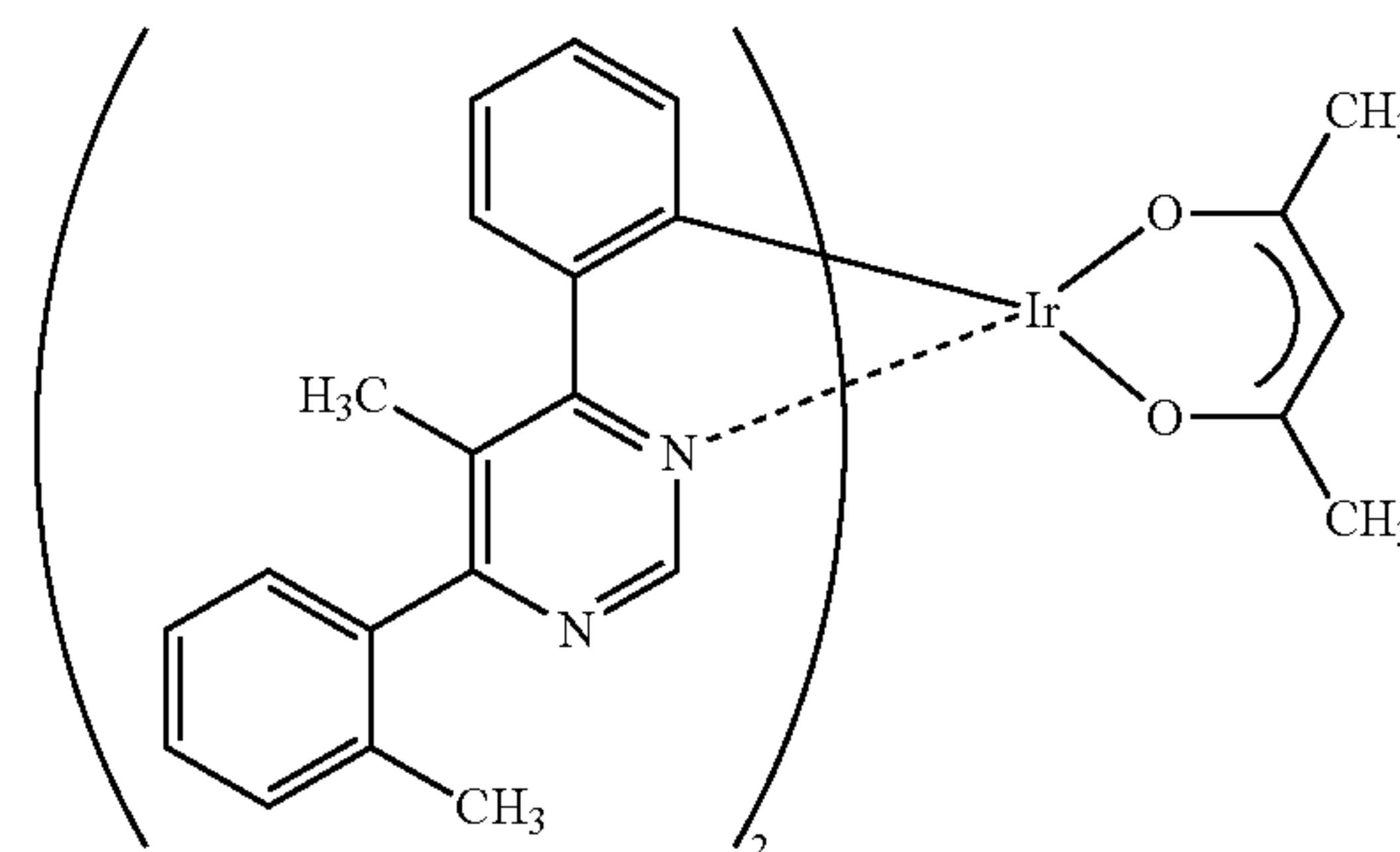
(xii) Ir(mpmppm) 2 (acac)
