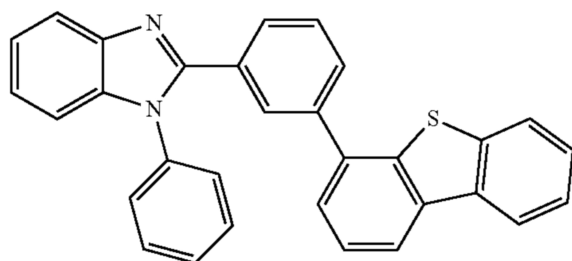
mDBTIm-II
