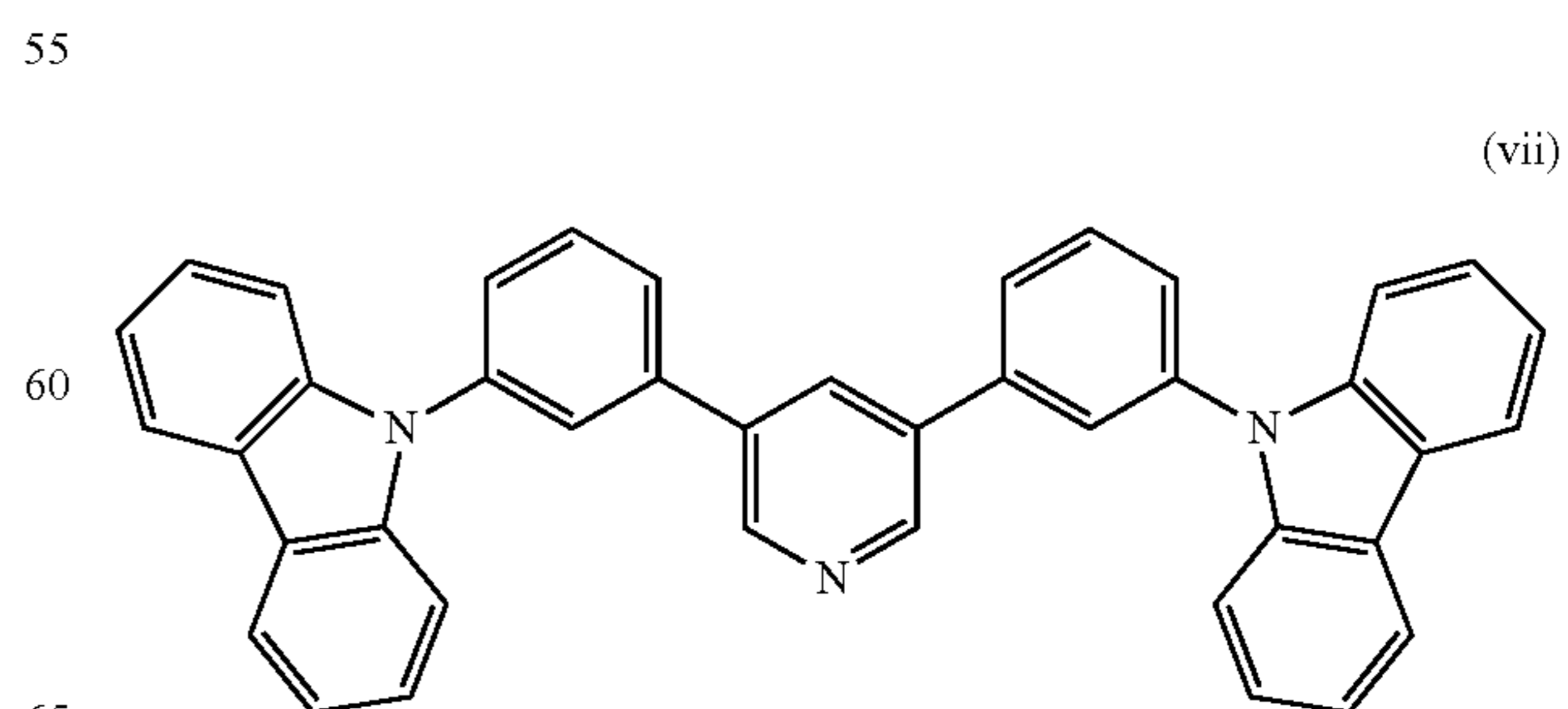
3,5DCzPPy
