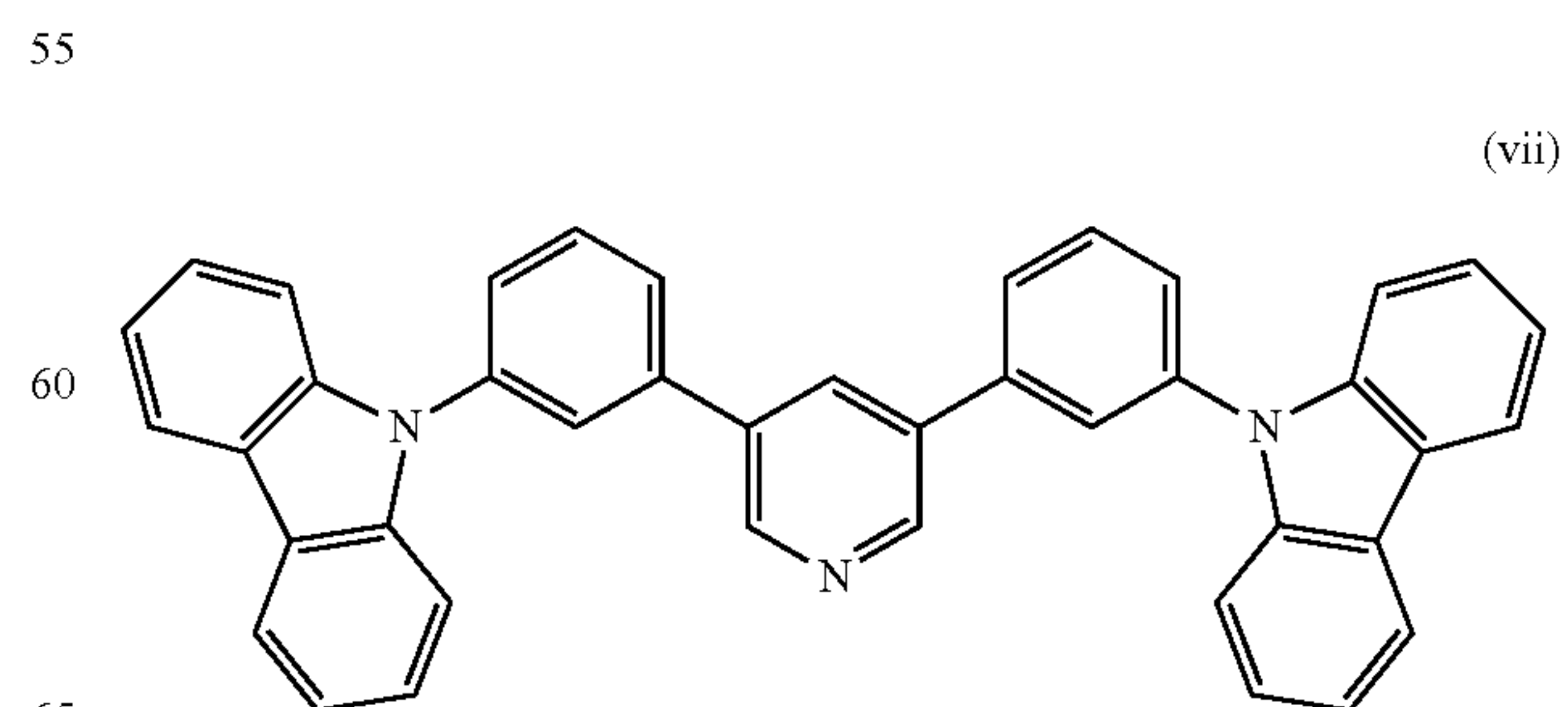
3,5DCzPPy
