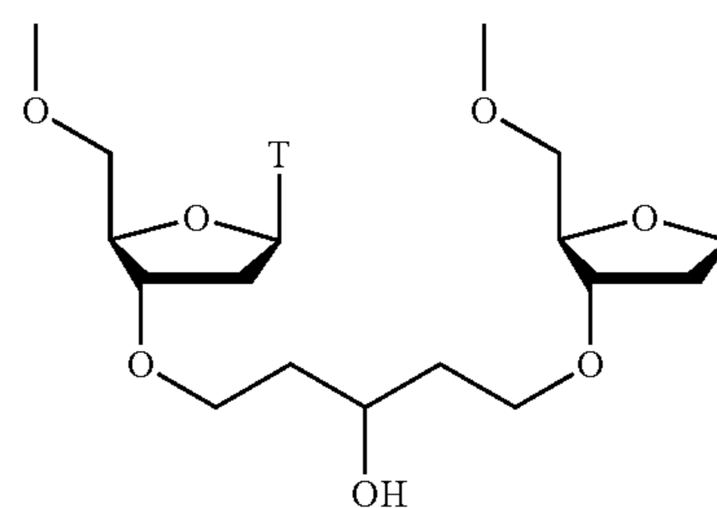
Bis-1,5-O-(3'-thymidyl)-1,3,5-pentanetriol Linker
