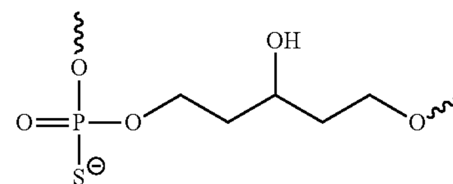
1,3,5-Pentanetriol Linker
