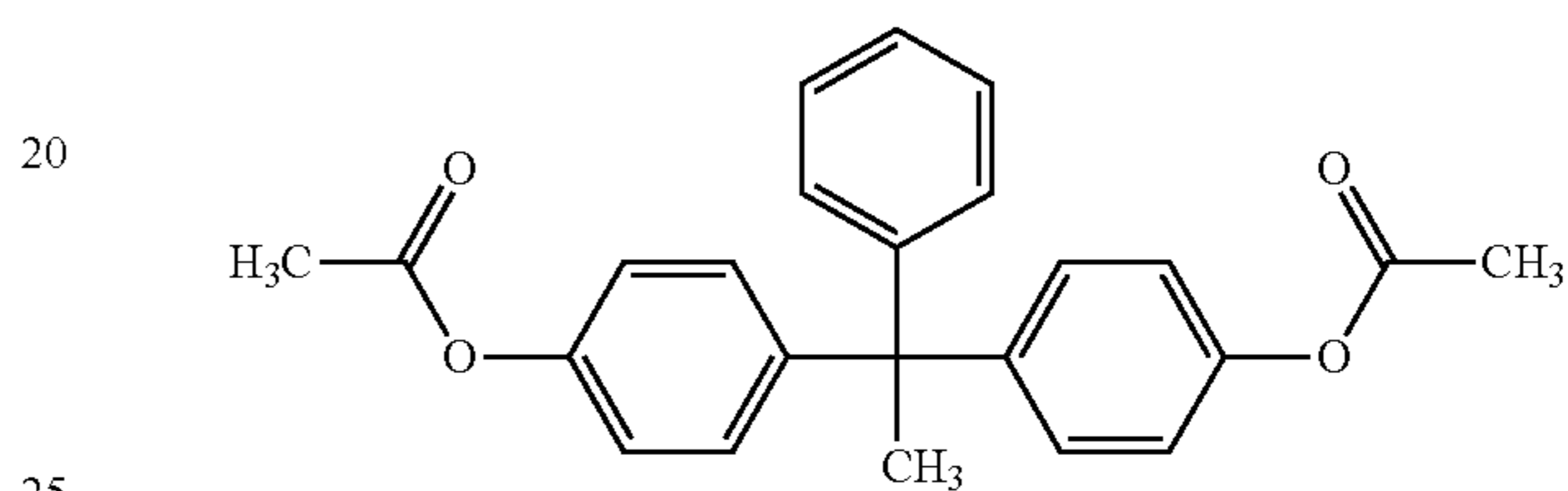
1,1-Bis-(4-acetoxyphenyl)-1-phenyl-ethane (I-10)
