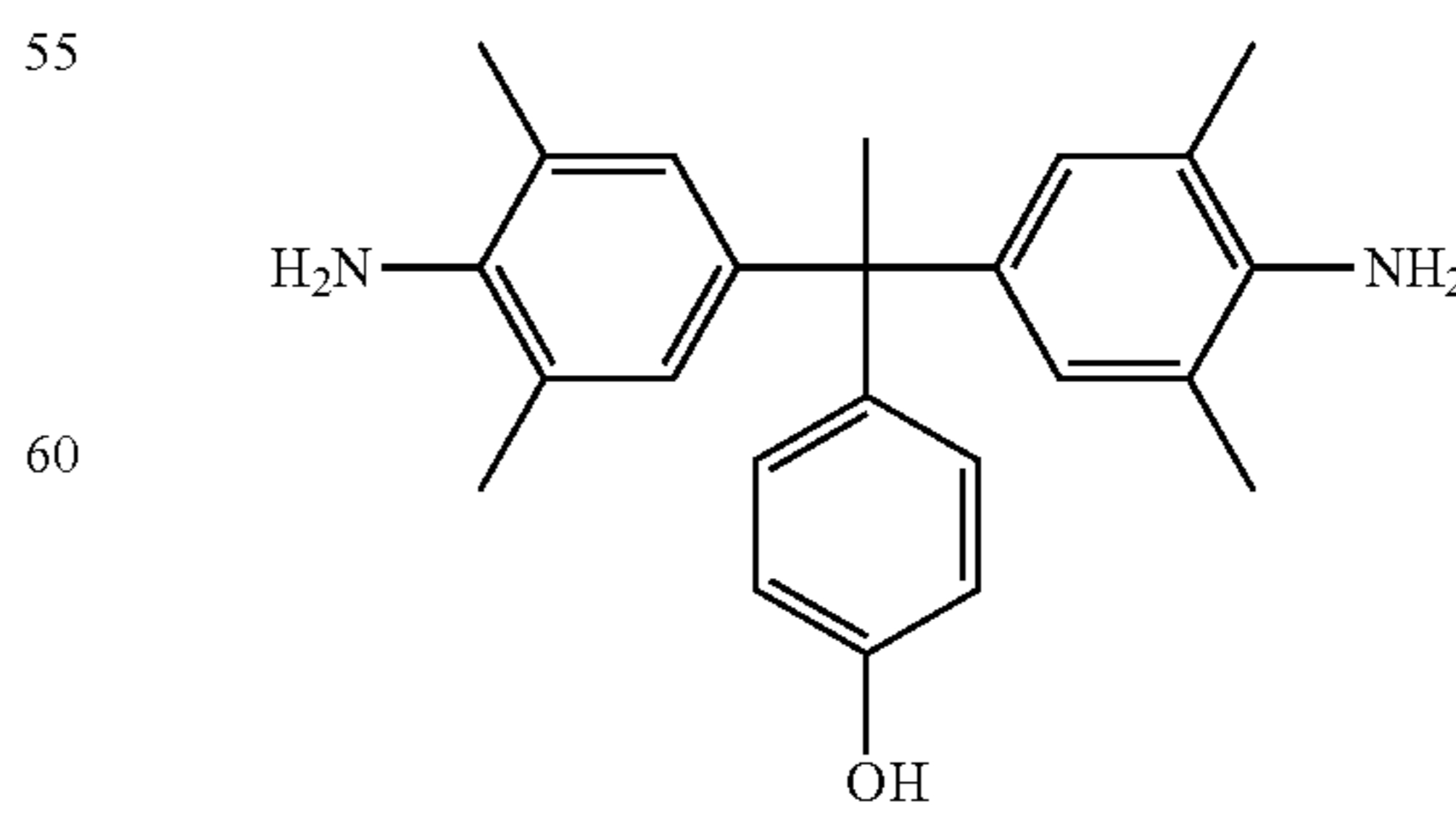
1,1-Bis(4-amino-3,5-dimethylphenyl)-1-(4-hydroxyphenyl)-ethane (I-18)
