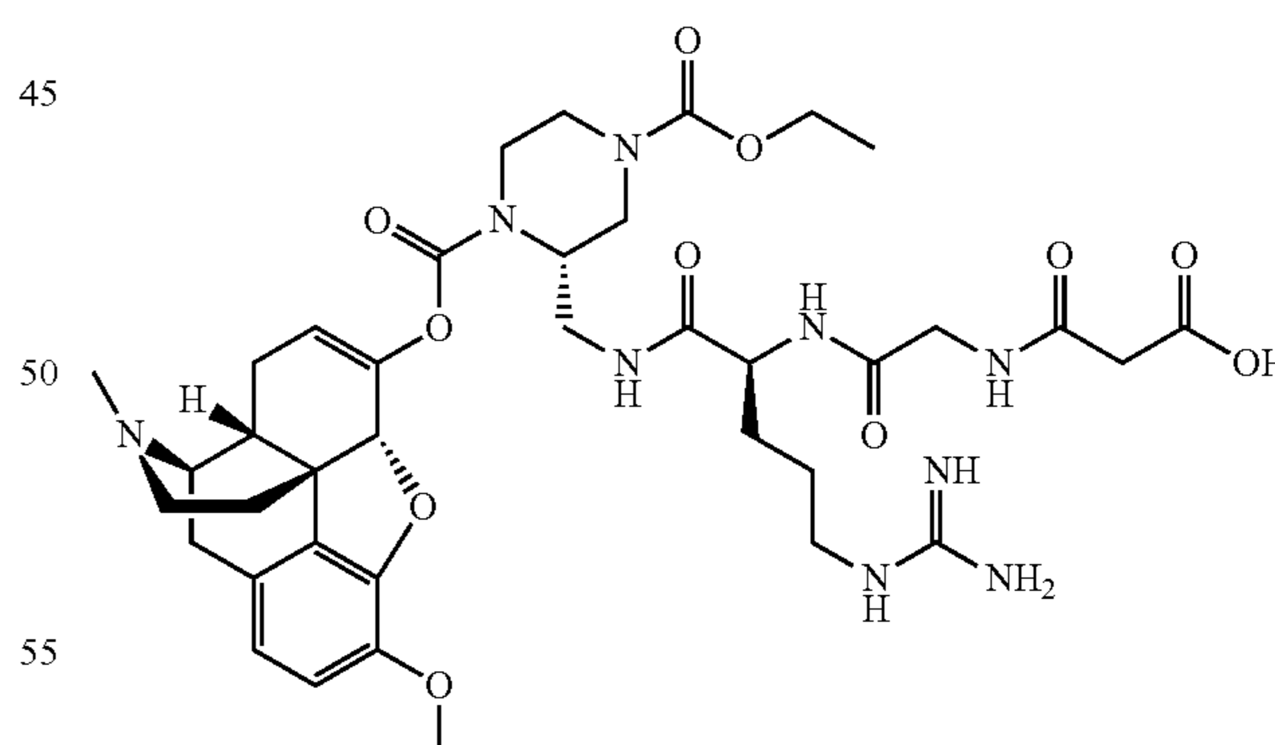
KC-45
