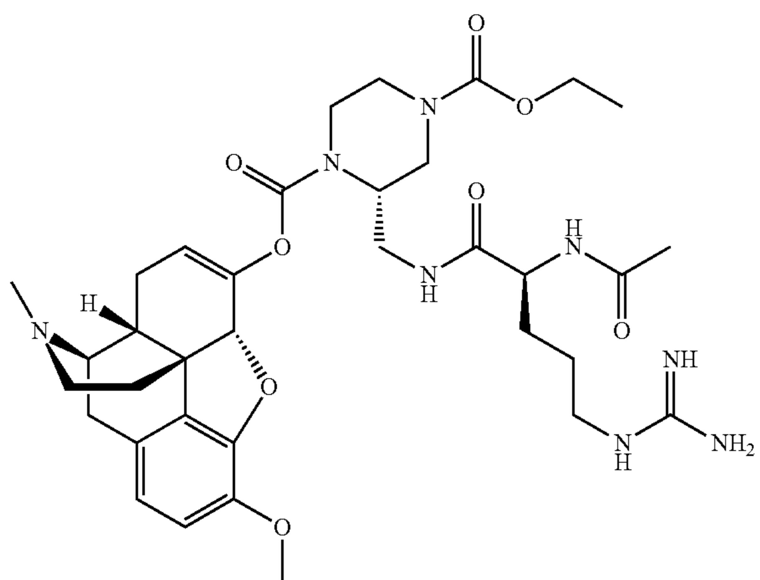
KC-43
