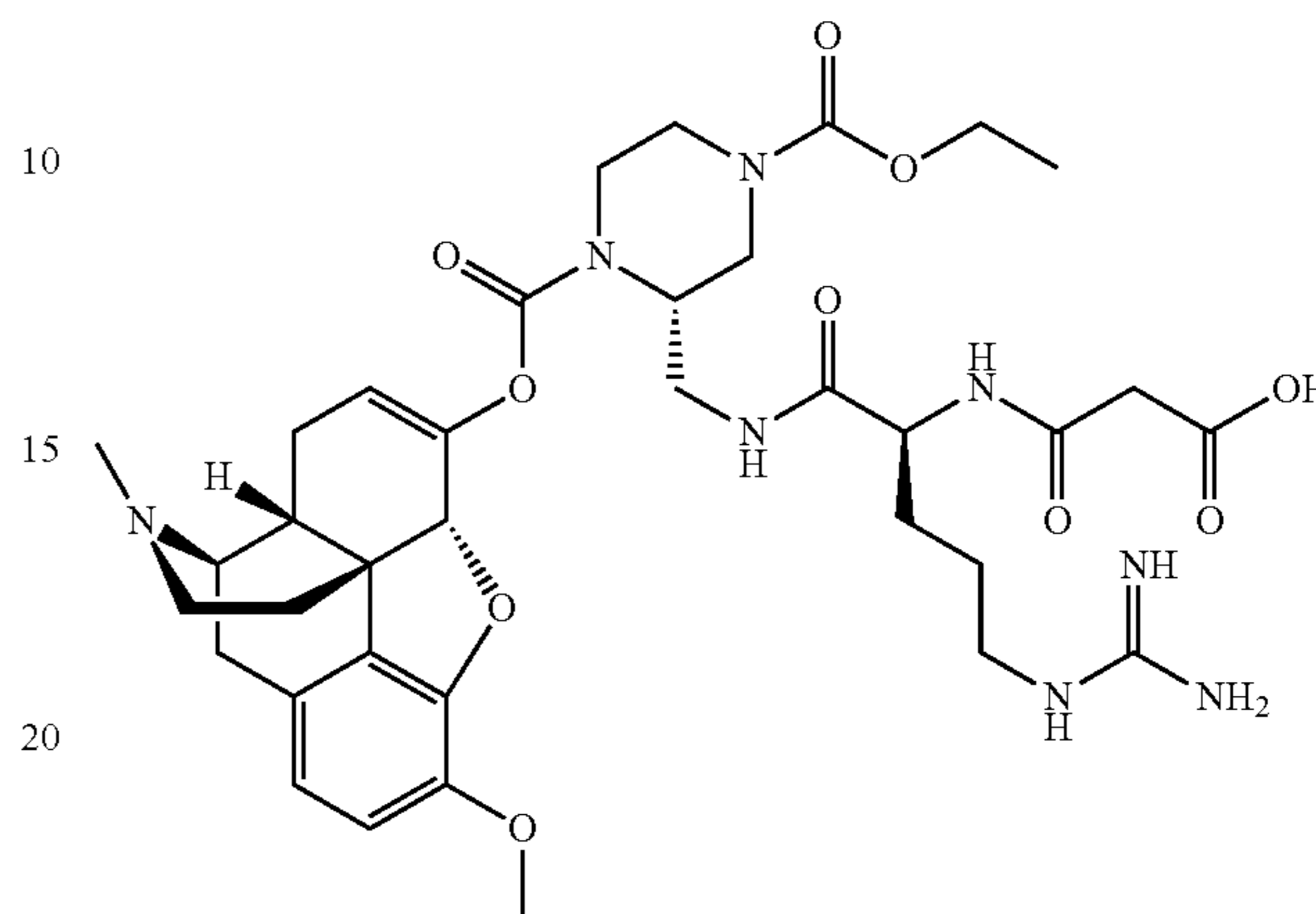
KC-44
