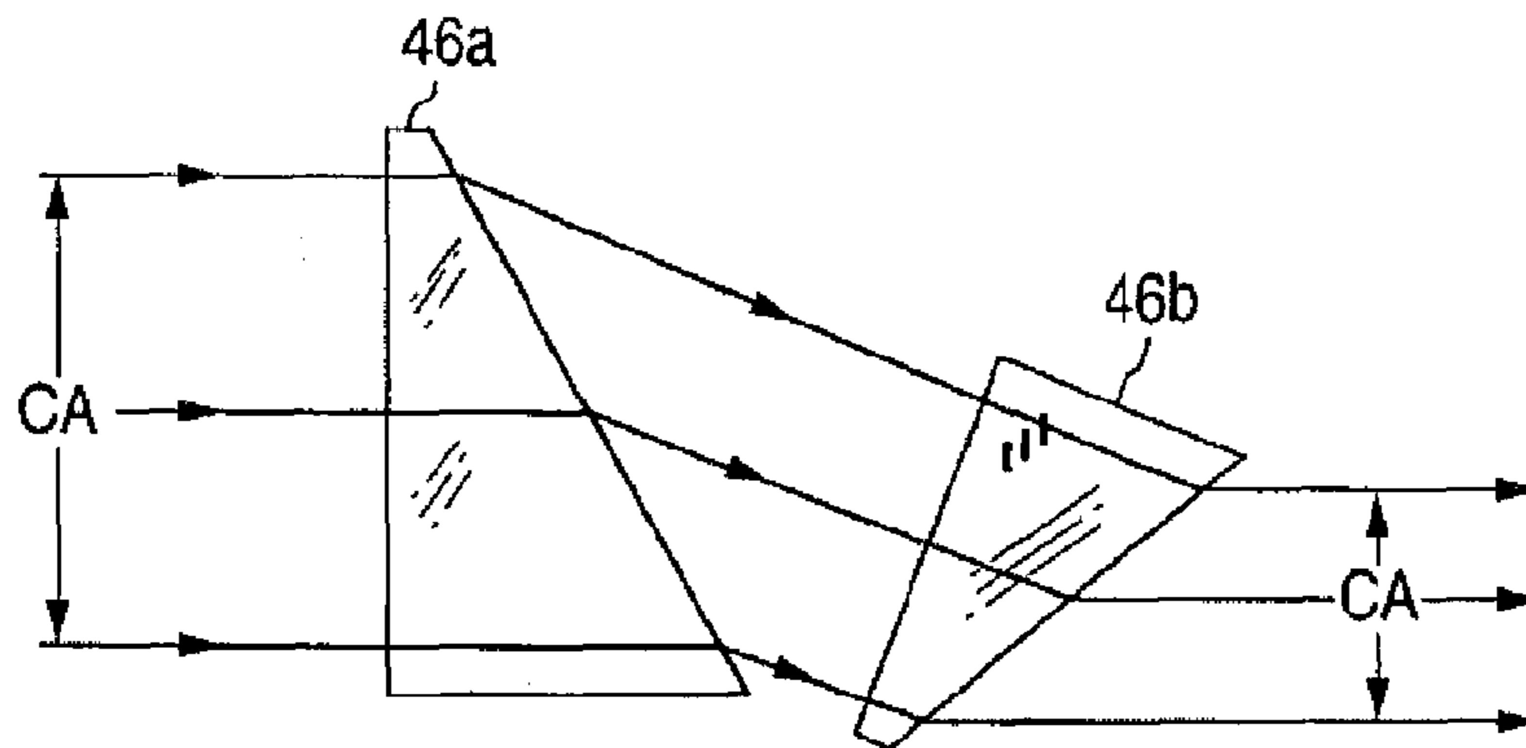
FIG. 18
