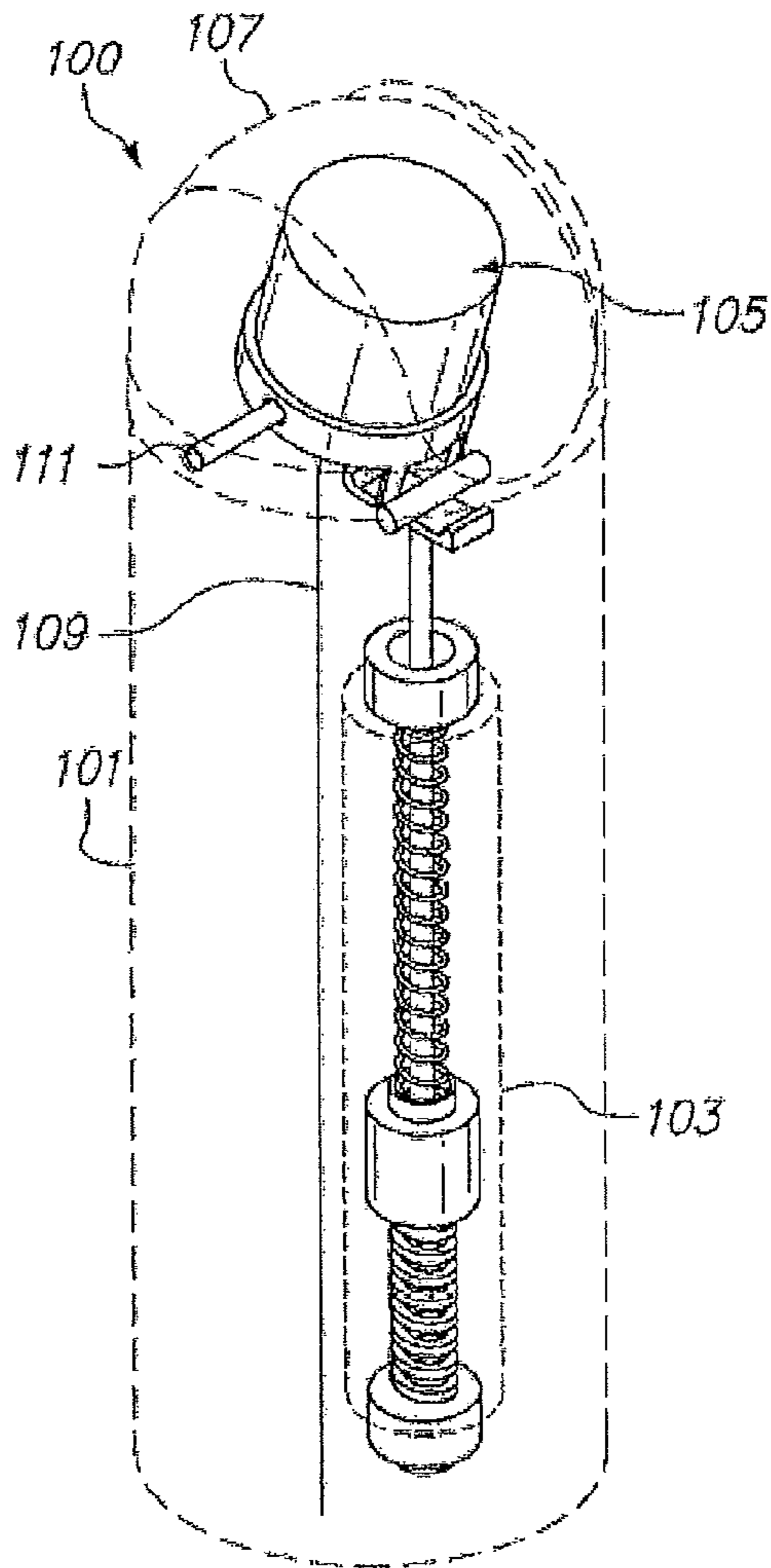
PRIOR ART Fig. 1A
