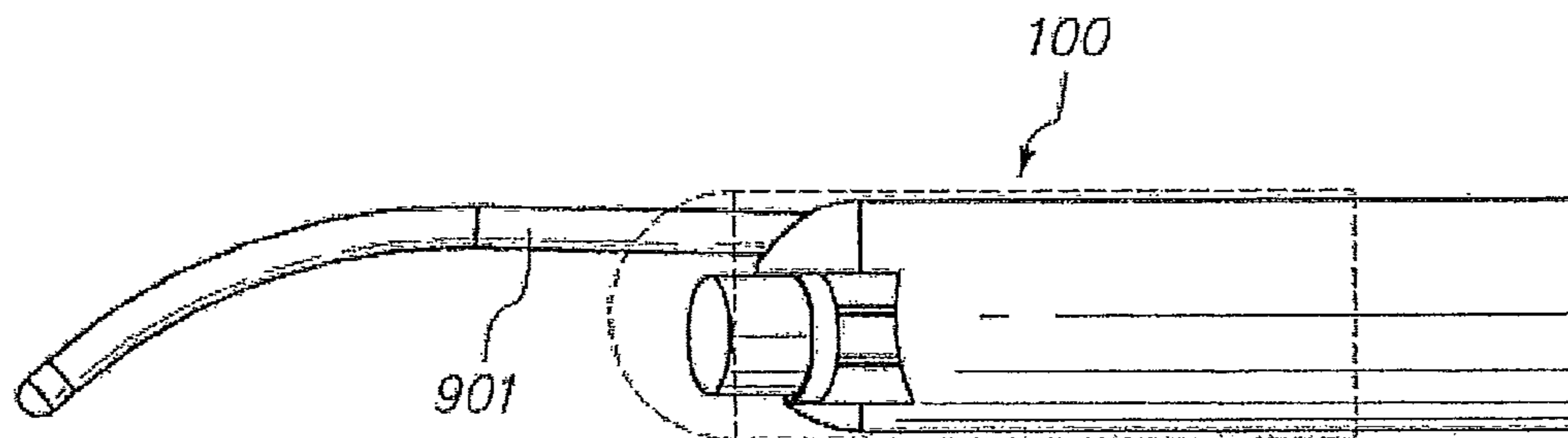
PRIOR ART Fig. 1E
