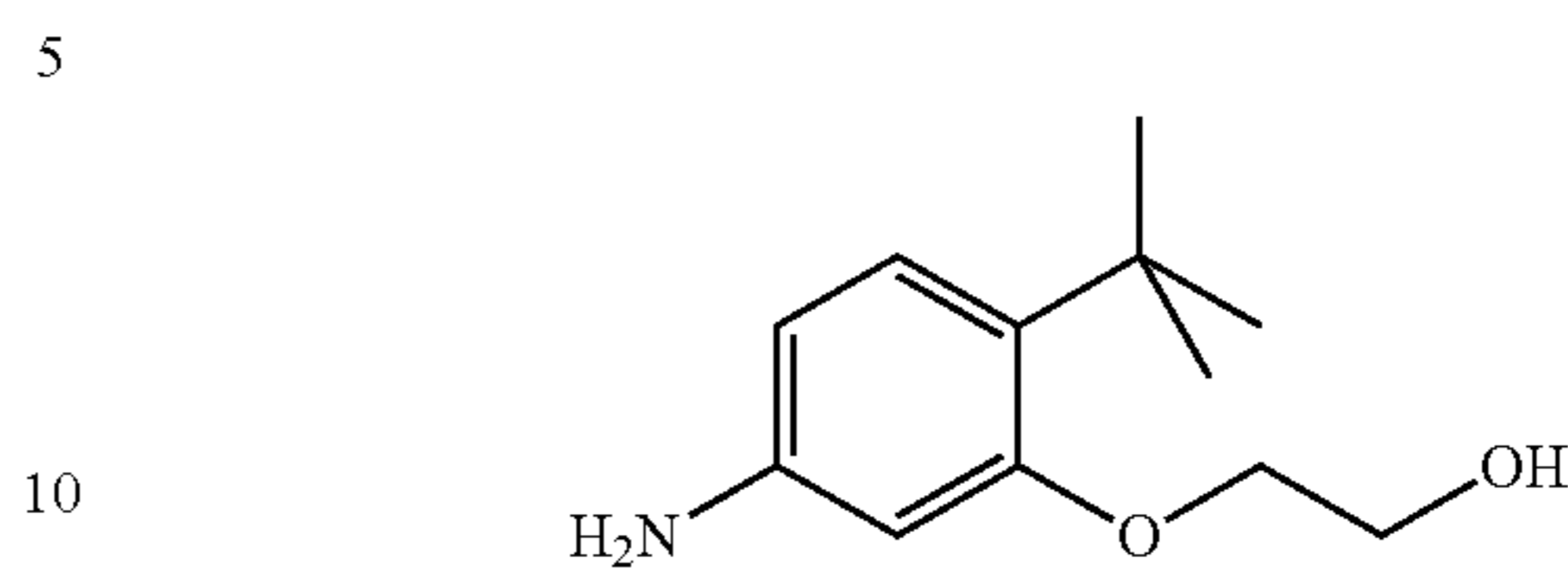
C-4; 2-(2-tert-Butyl-5-aminophenoxy)ethanol
