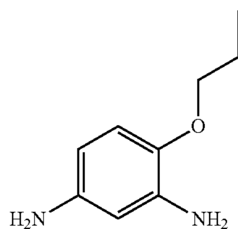
D-5; 4-Propoxybenzene-1,3-diamine
