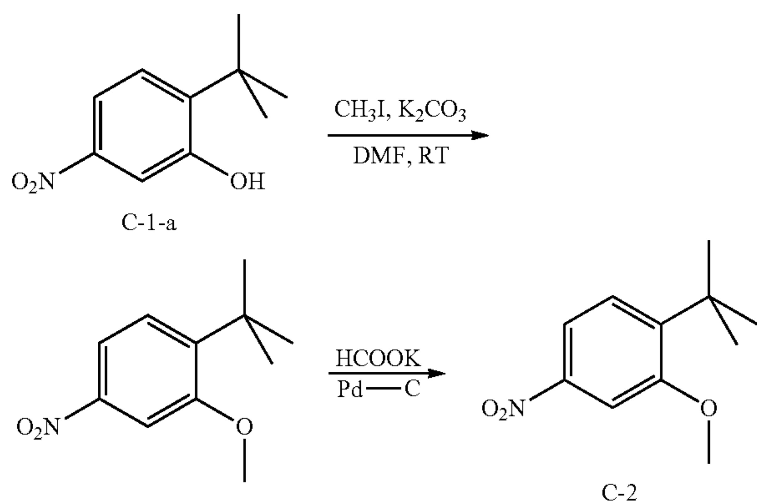
1-tert-Butyl-2-methoxy-4-nitrobenzene
