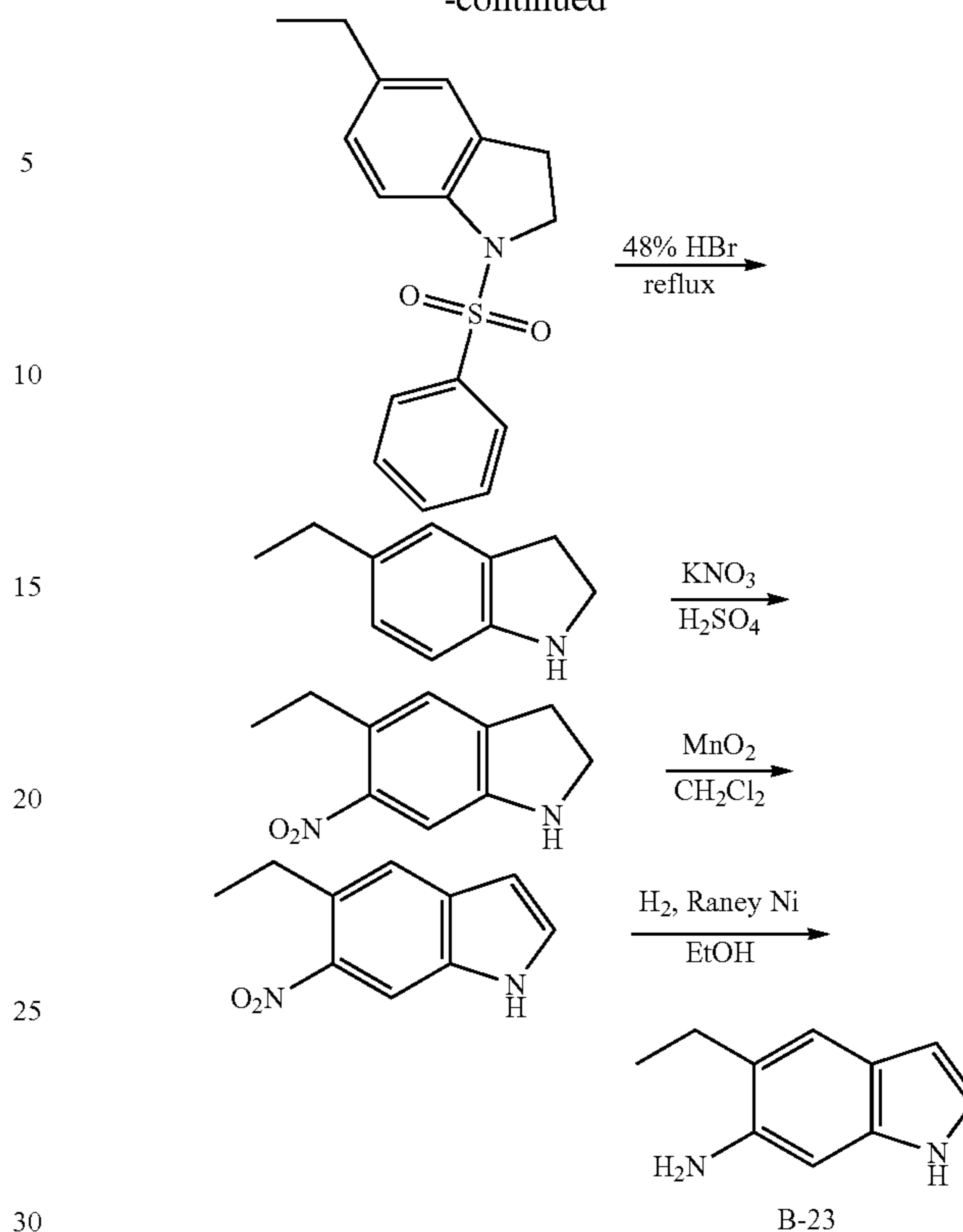
1-Benzenesulfonyl-2,3-dihydro-1H-indole
