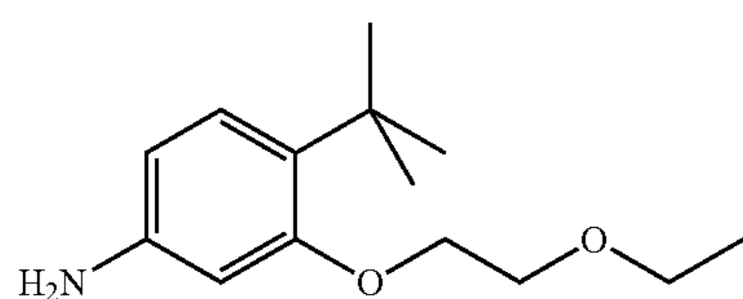
C-3; 3-(2-Ethoxyethoxy)-4-tert-butylbenzenamine
