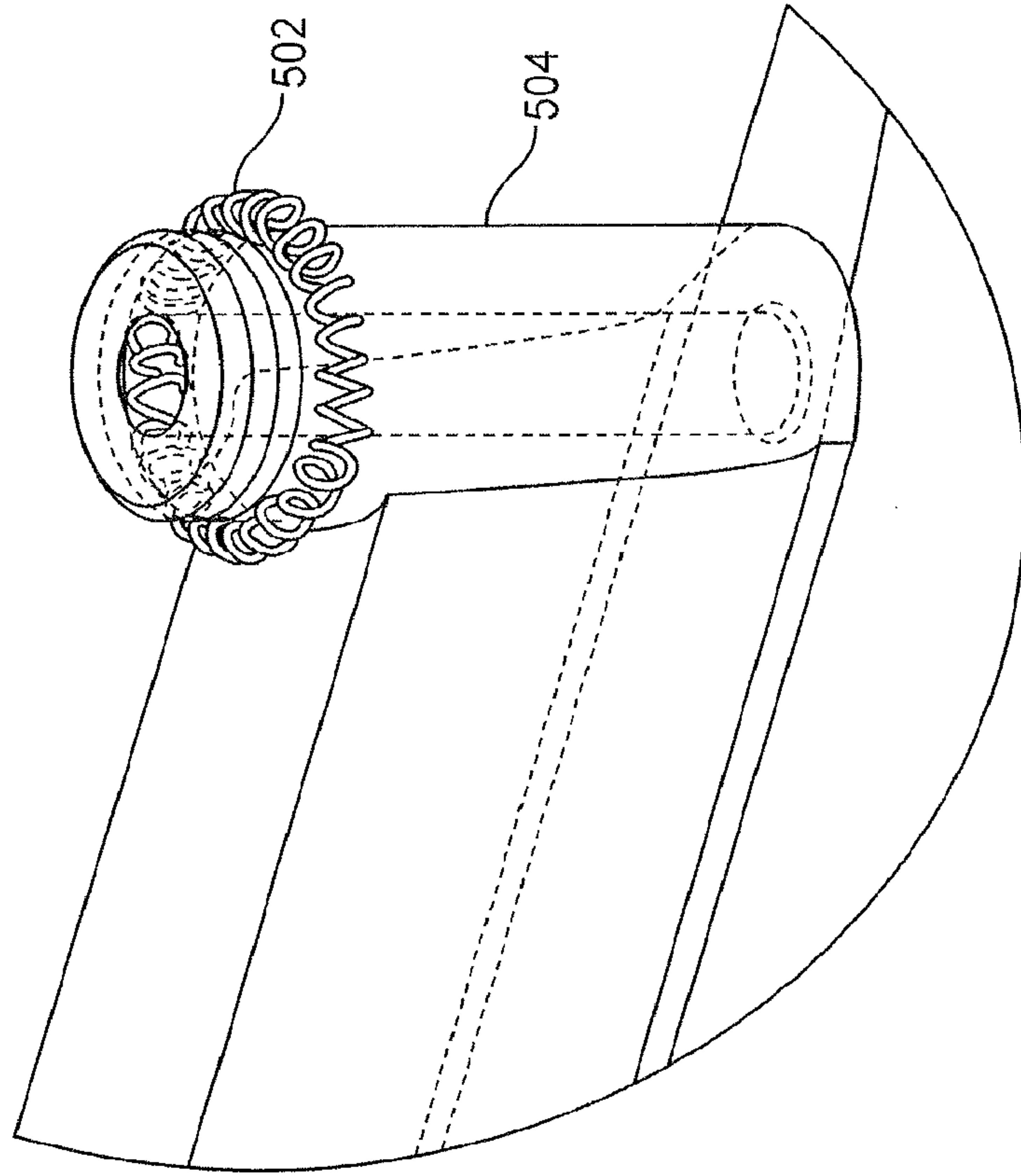
FIG. 16B
