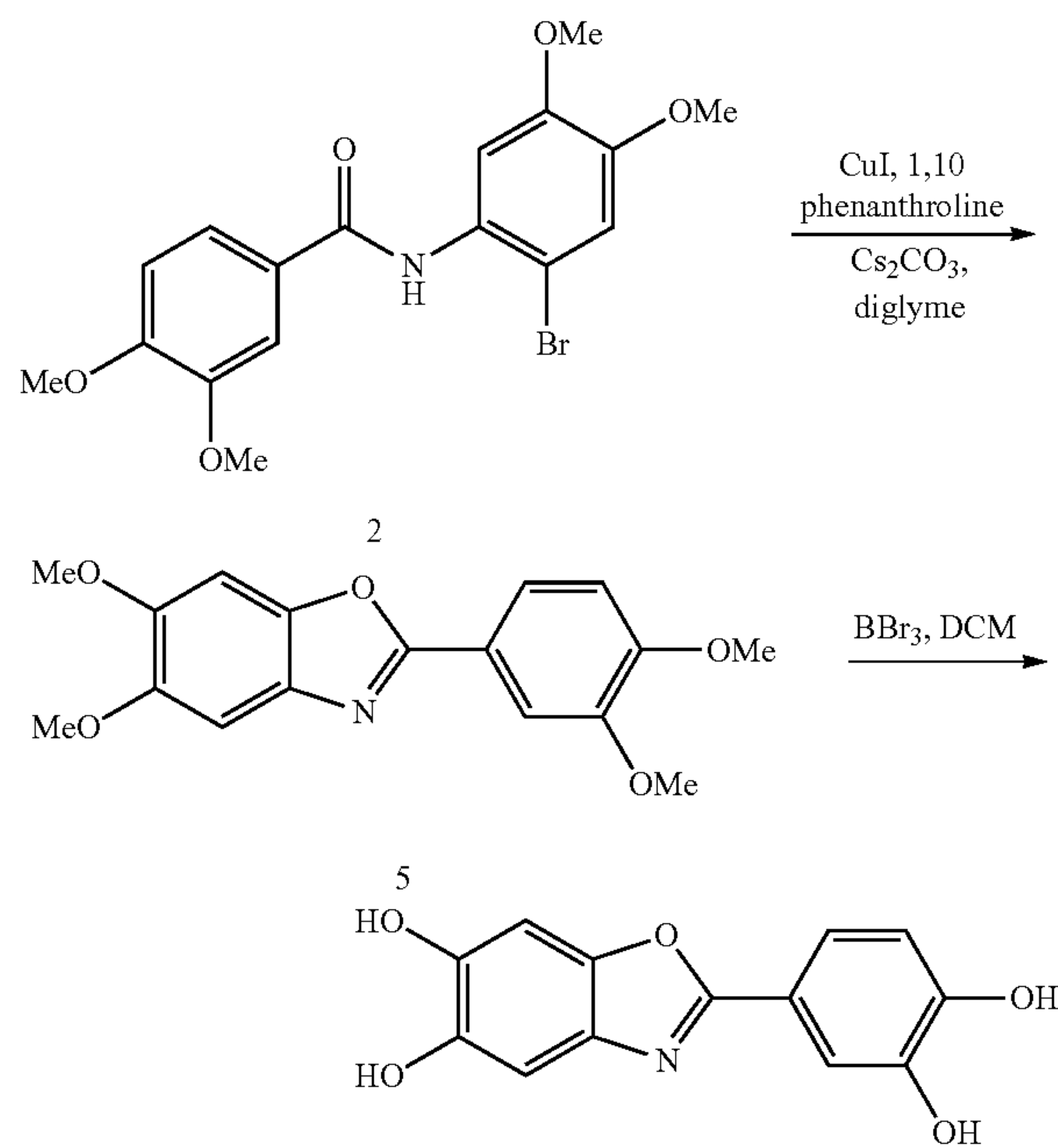
SA-54
