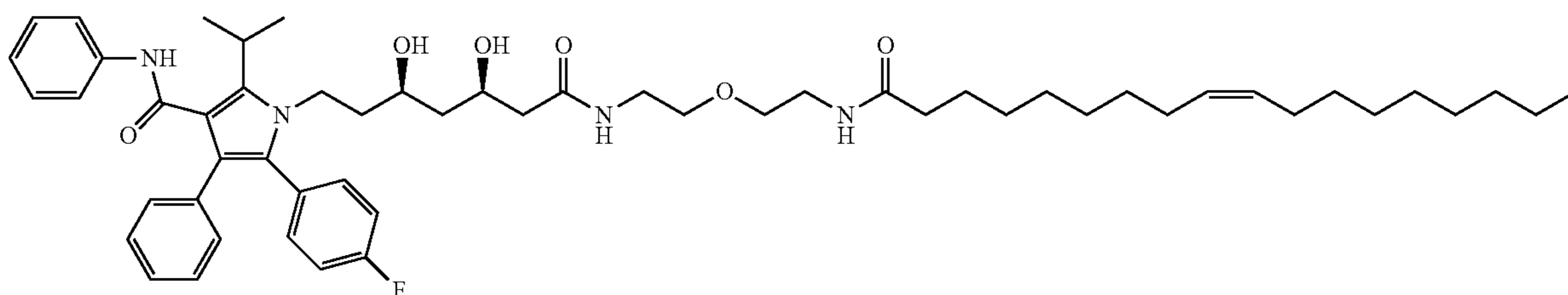
1-((3R,5R)-3,5-dihydroxy-7-((2-(methyl(2-oleamidoethyl)amino)ethyl)amino)-7-oxoheptyl)-5-(4-fluorophenyl)-2-isopropyl-N,4-diphenyl-1H-pyrrole-3-carboxamide (I-30)
