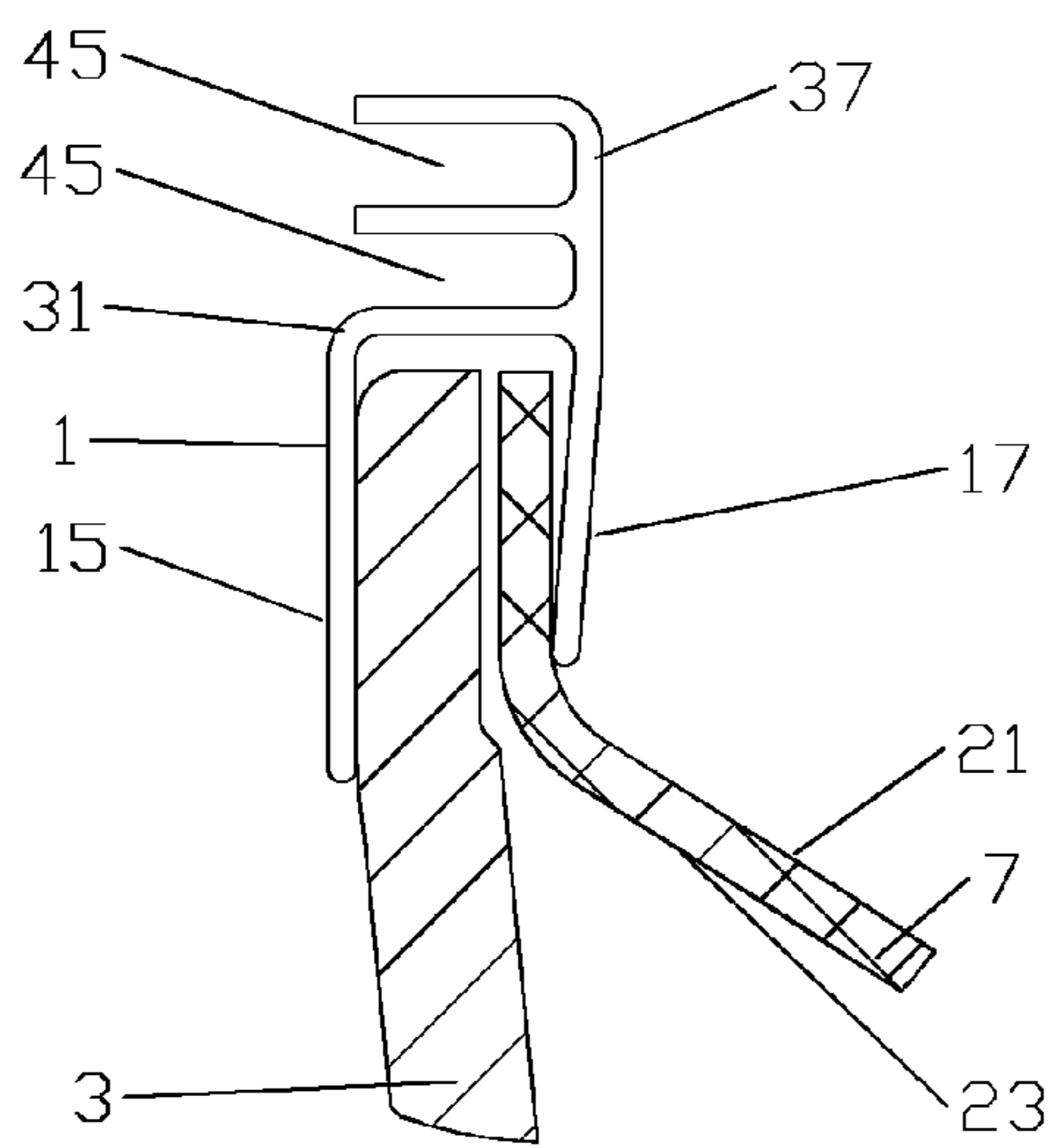
FIG. 38
