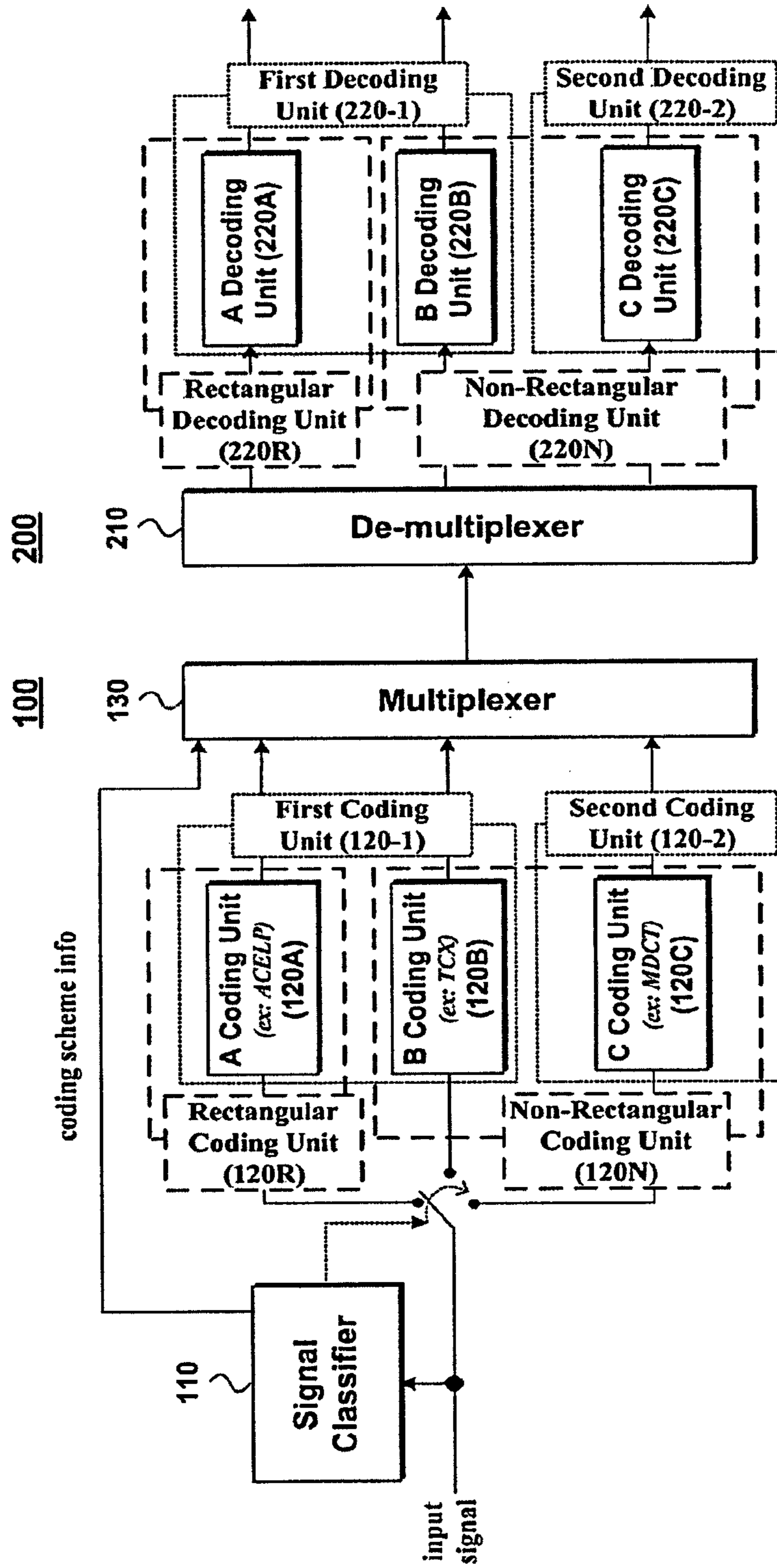
FIG. 1
