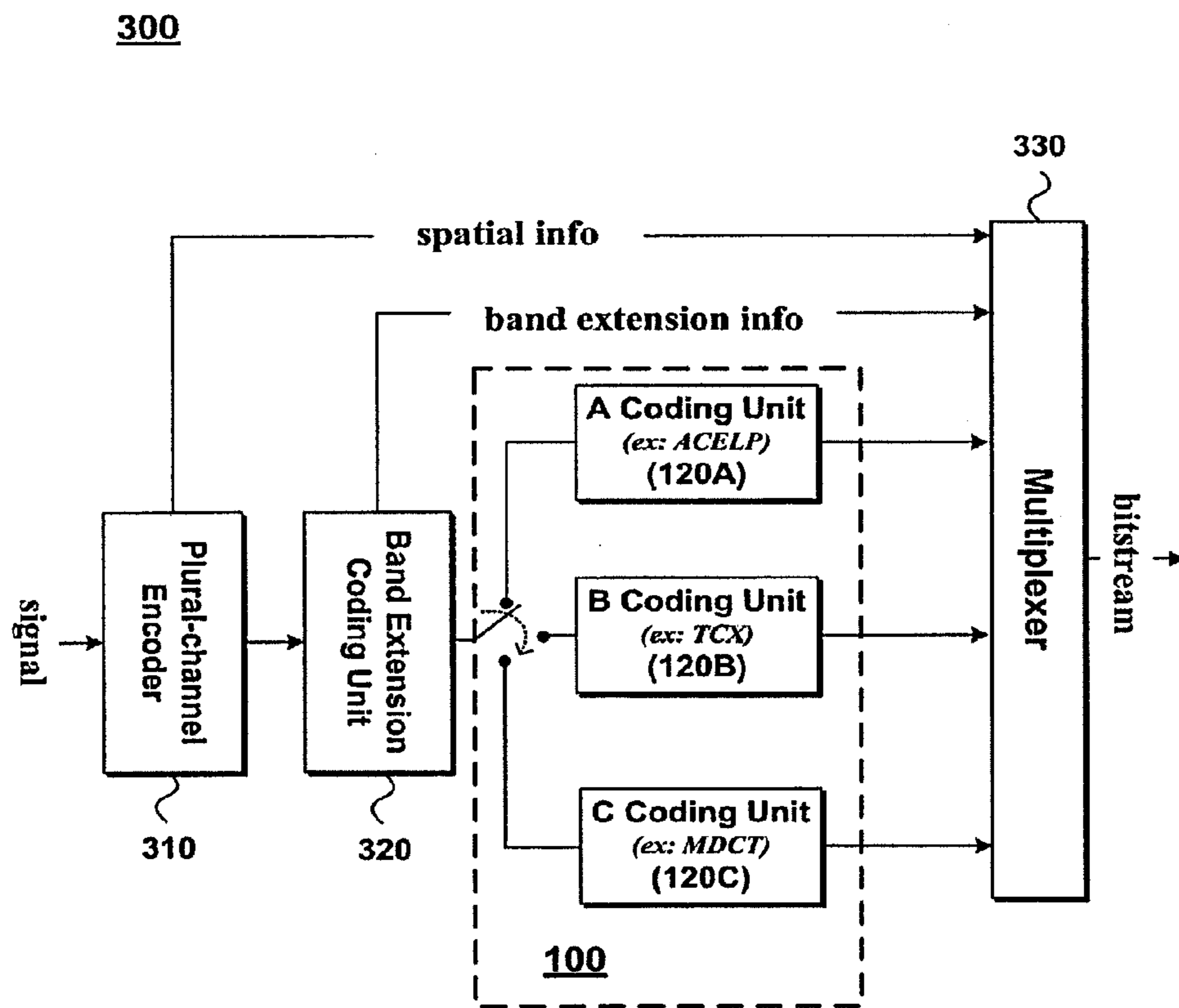
FIG. 33
