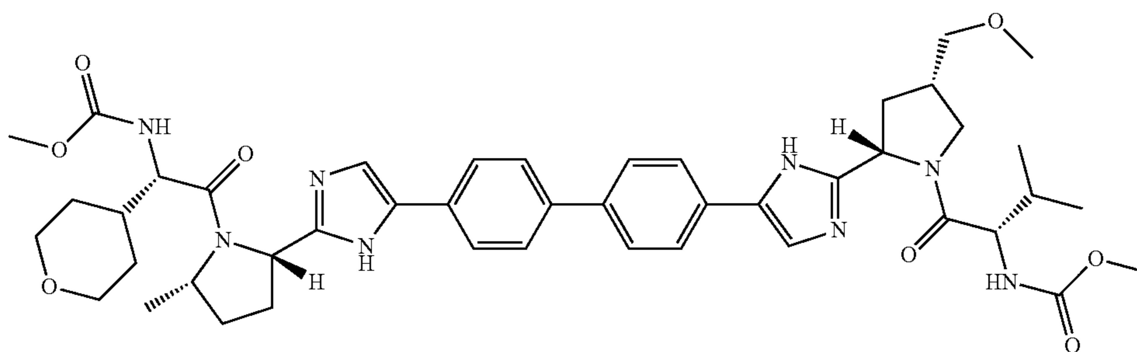
methyl ((2S)-1-[(2S,4S)-2-{5-[4'-(2-(2S,5S)-1-[(2S)-2-[(methoxycarbonyl)amino]-2-(tetrahydro-2H-pyran-4-yl)acetyl]-5-methylpyrrolidin-2-yl]-1H-imidazol-5-yl)biphenyl-4-yl]-1H-imidazol-2-yl}-4-(methoxymethyl)pyrrolidin-1-yl]-3-methyl-1-oxobutan-2-yl}carbamate
