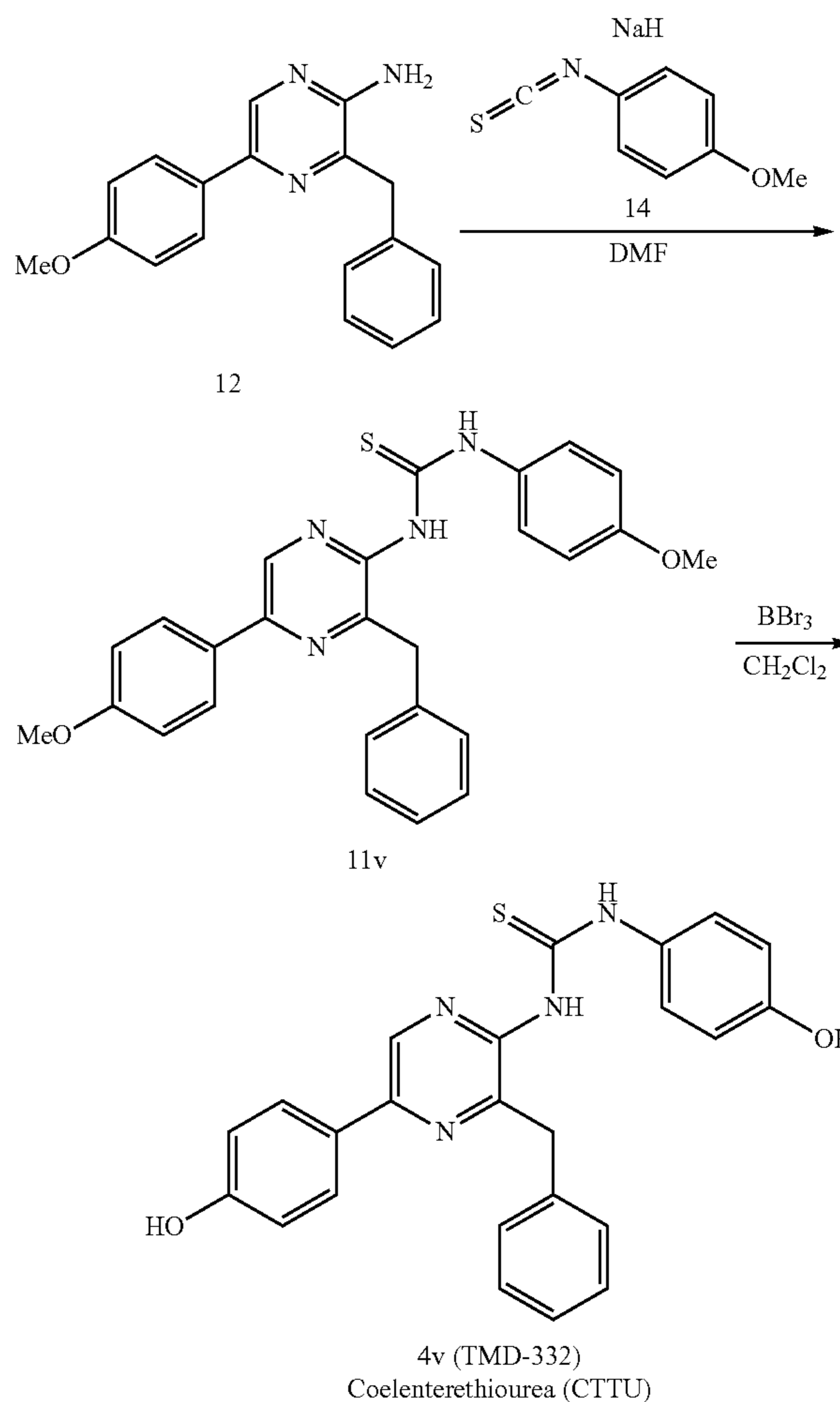
1-[3-Benzyl-5-(4-methoxyphenyl)pyrazin-2-yl]-3-(4-methoxyphenyl)thiourea (11v)
