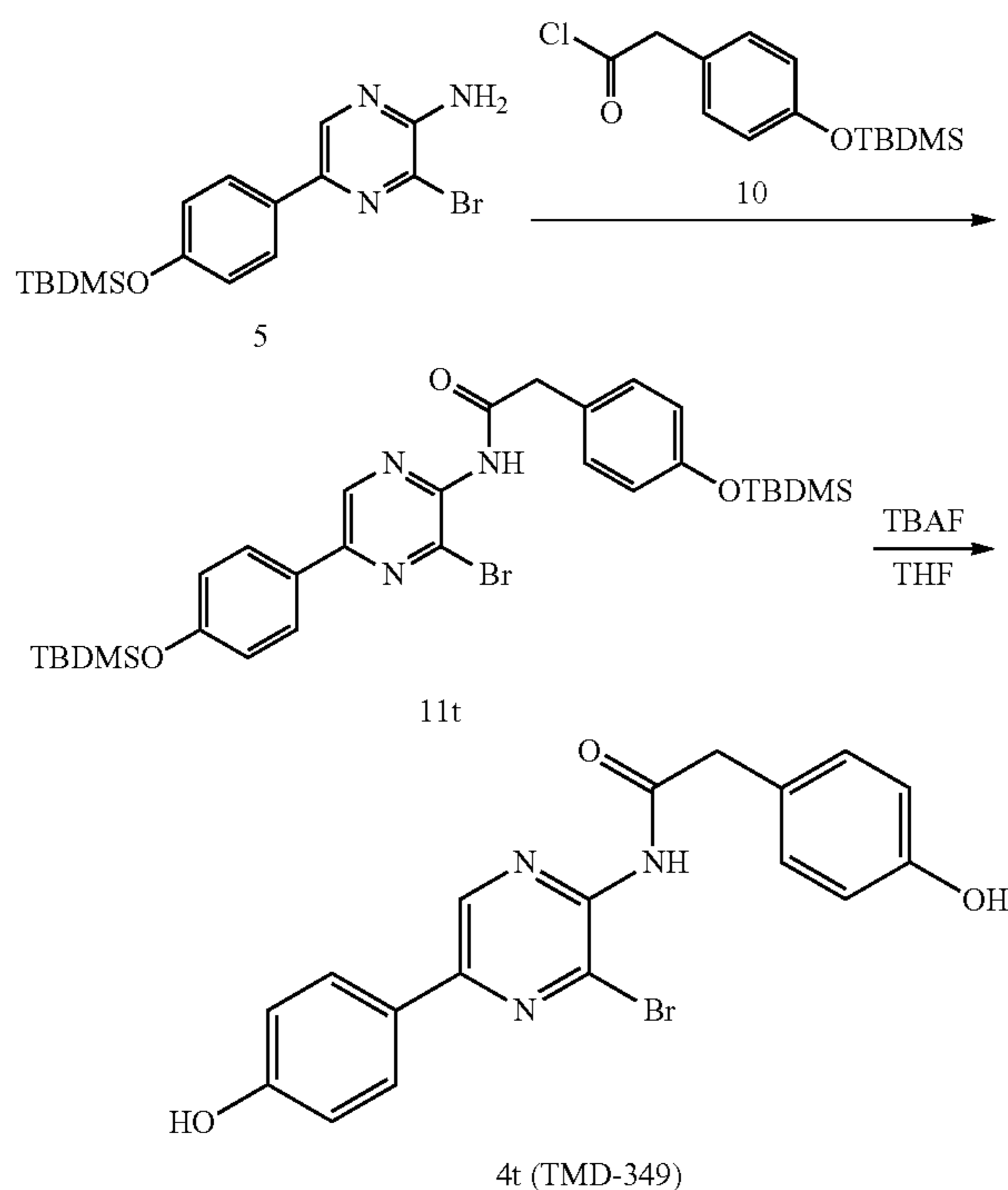
N-[3-Bromo-5-{4-(tert-butyldimethylsilyloxy)phenyl}pyrazin-2-yl]-2-[4-(tert-butyldimethylsilyloxy)phenyl]acetamide (11t)
