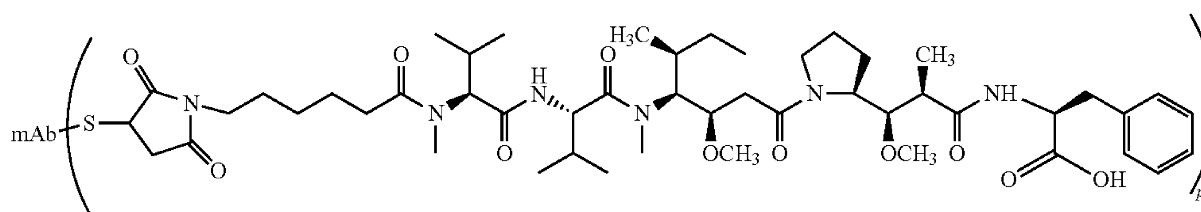
L-MC-MMAF
