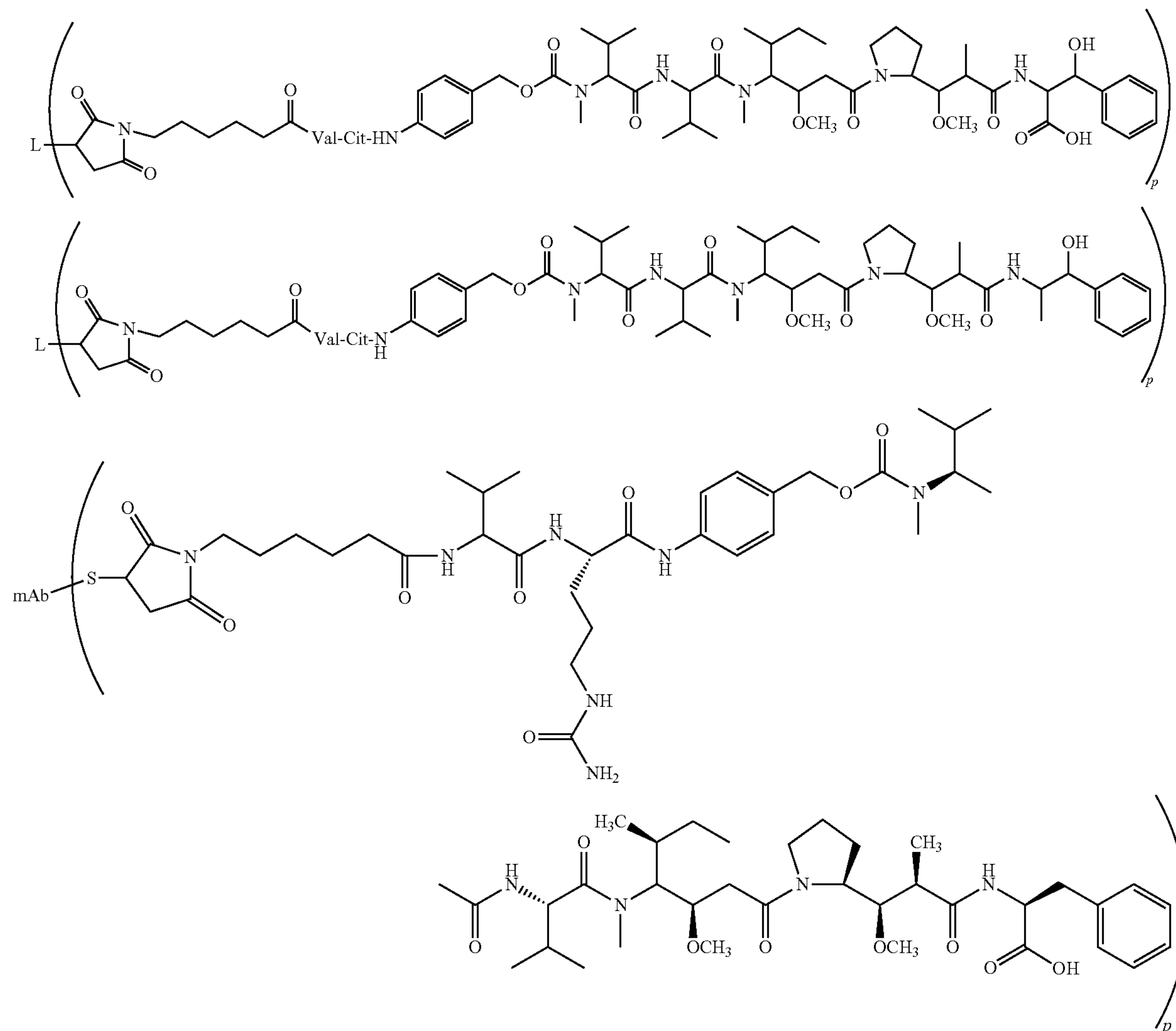
L-MC-vc-PAB-MMAF
