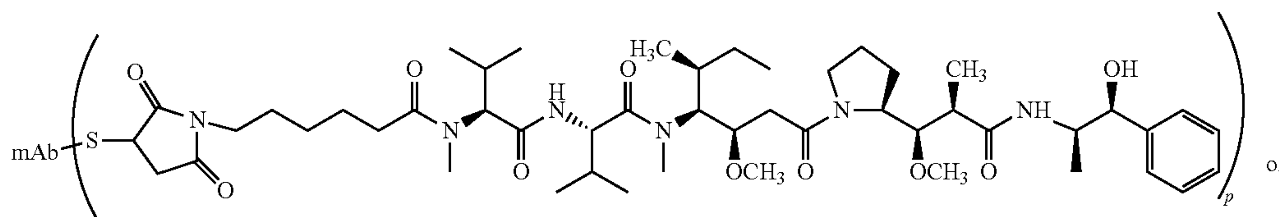
L-MC-MMAE
