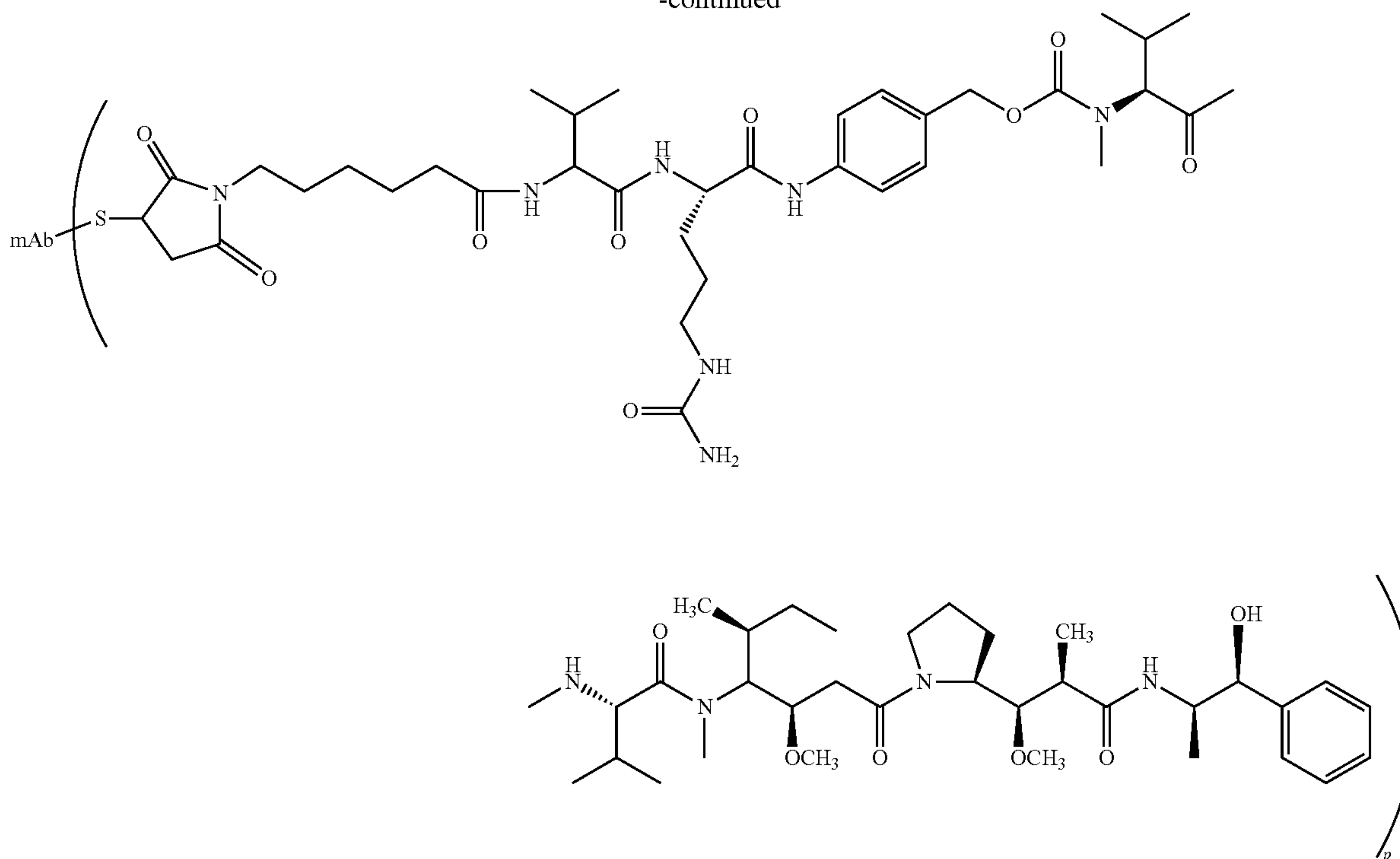
L-MC-vc-PAB-MMAE
