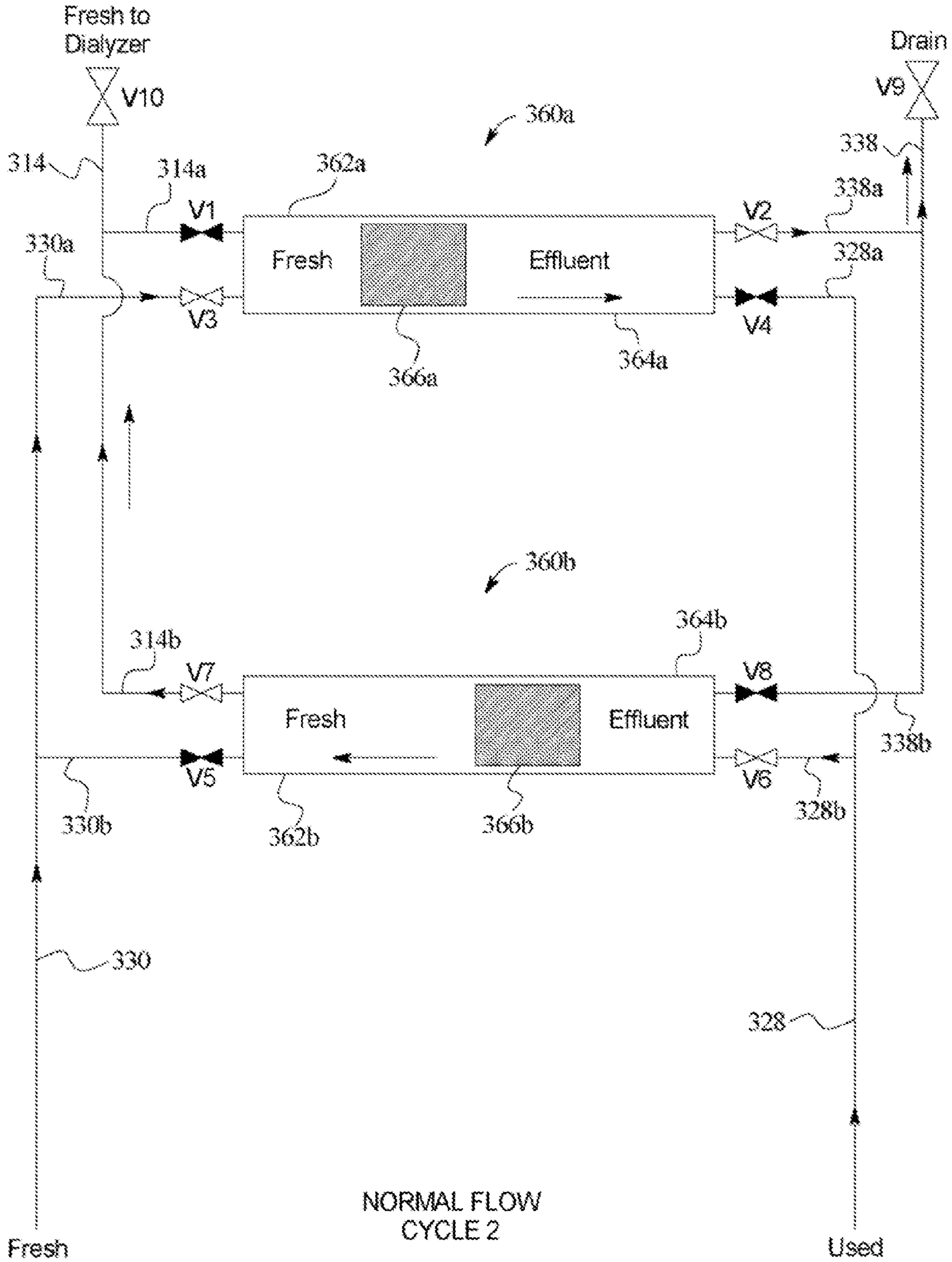
FIG. 27C
