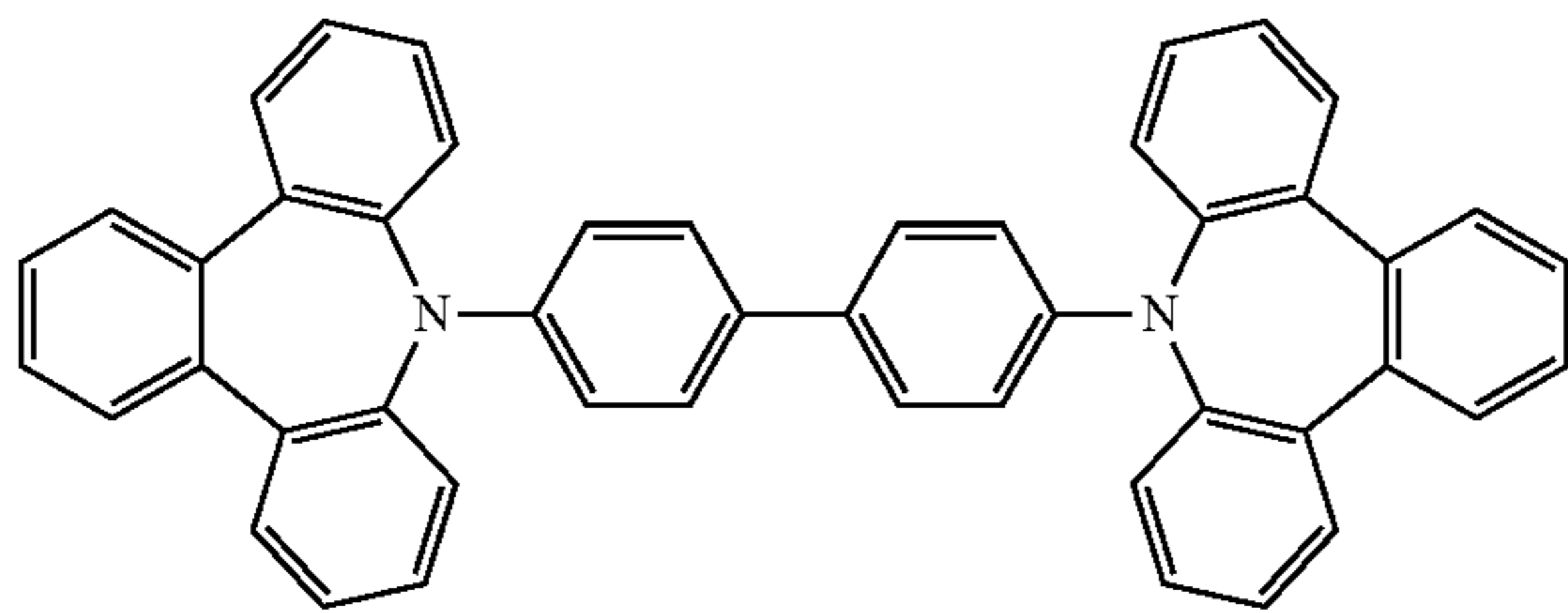
EB-3; E a = 1.9 eV, I p = 5.2 eV
