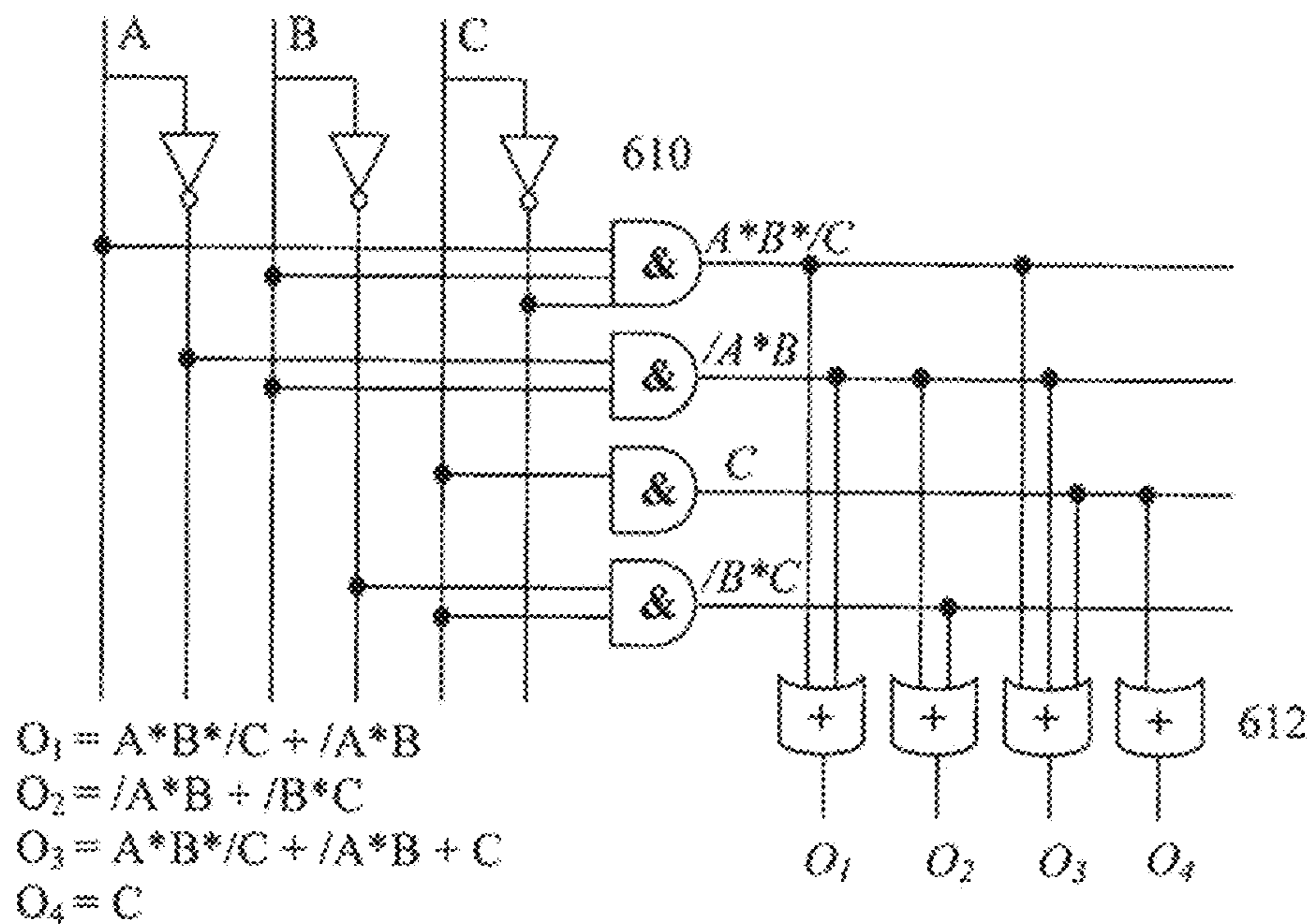
Fig. 6B
