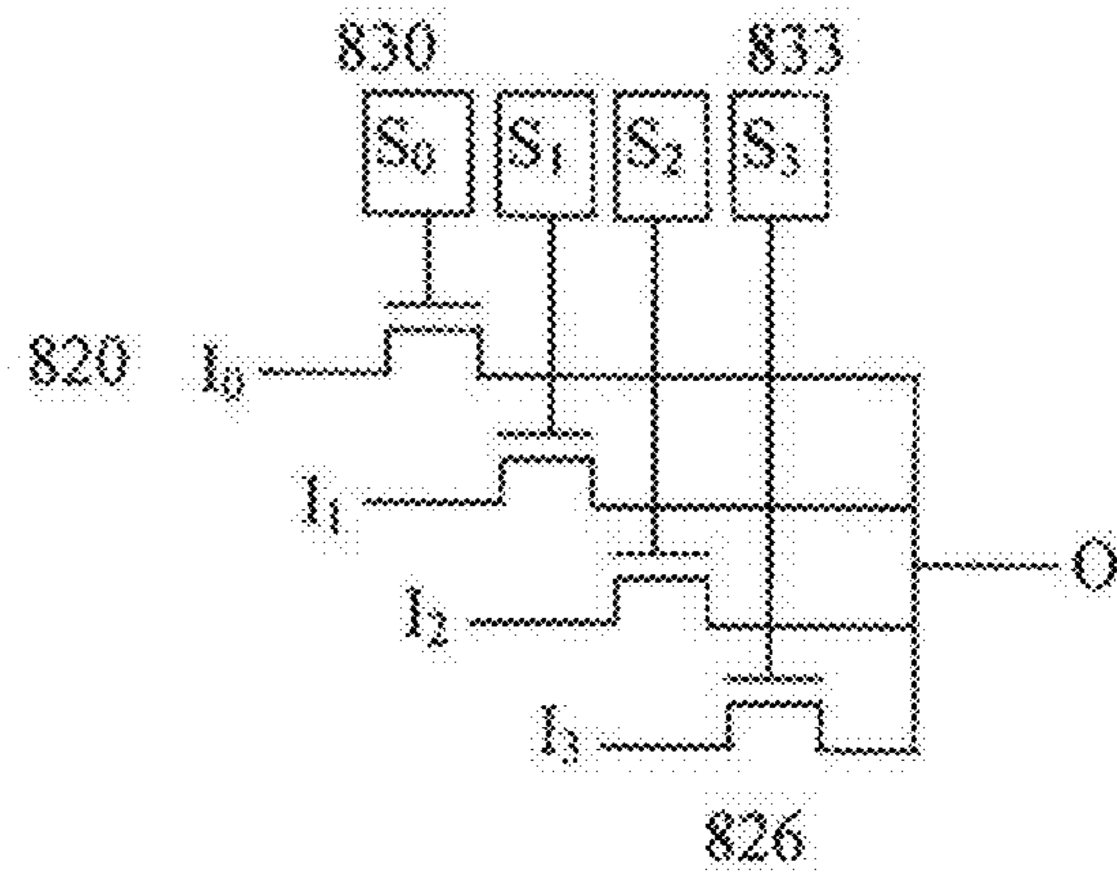
Fig. 8B
