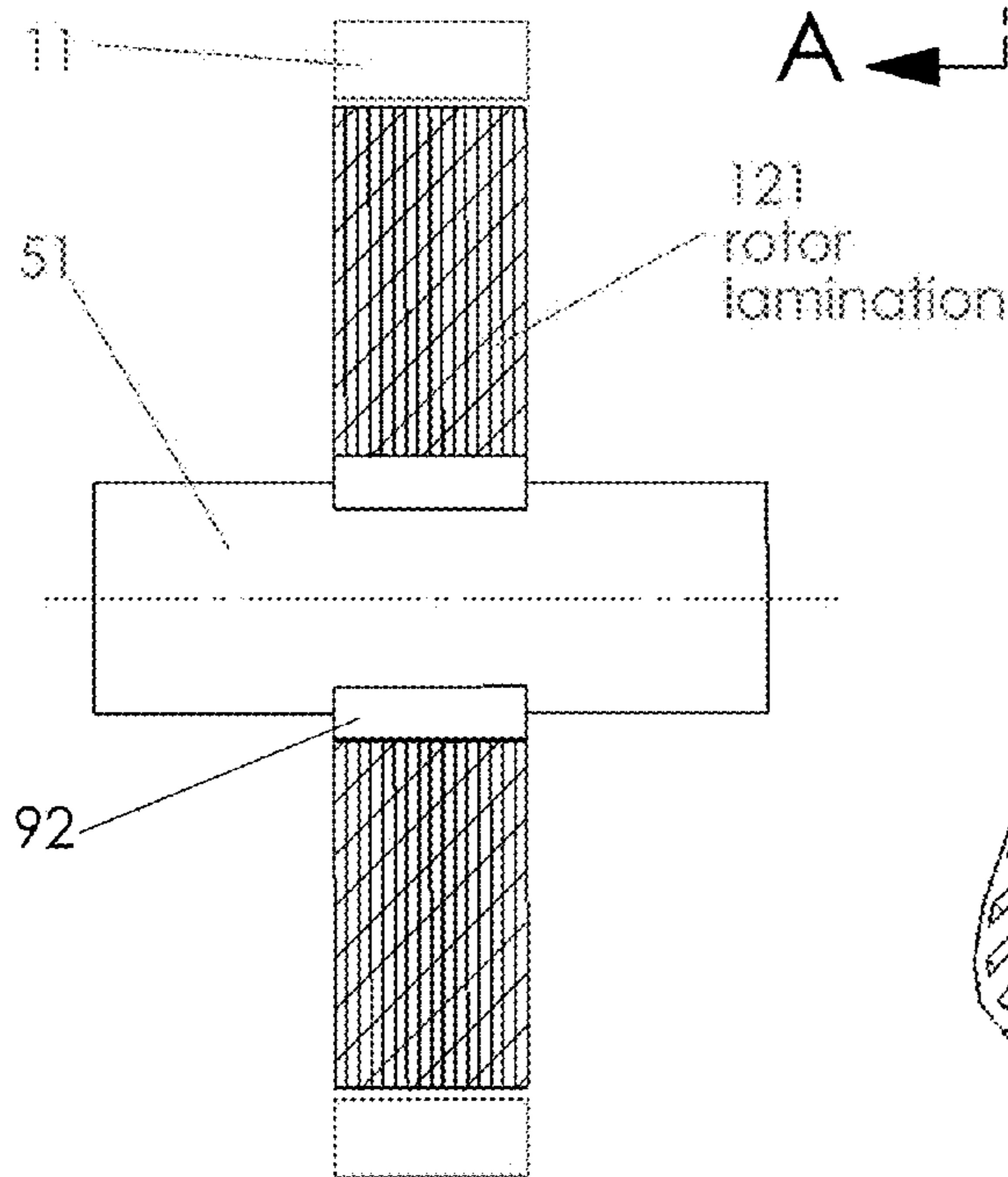
SECTION A-A
