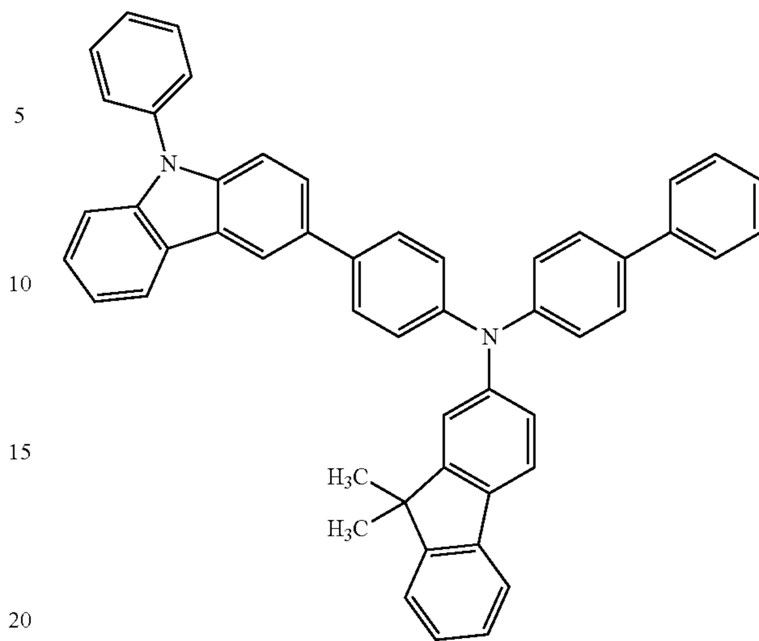
PCBBiF
