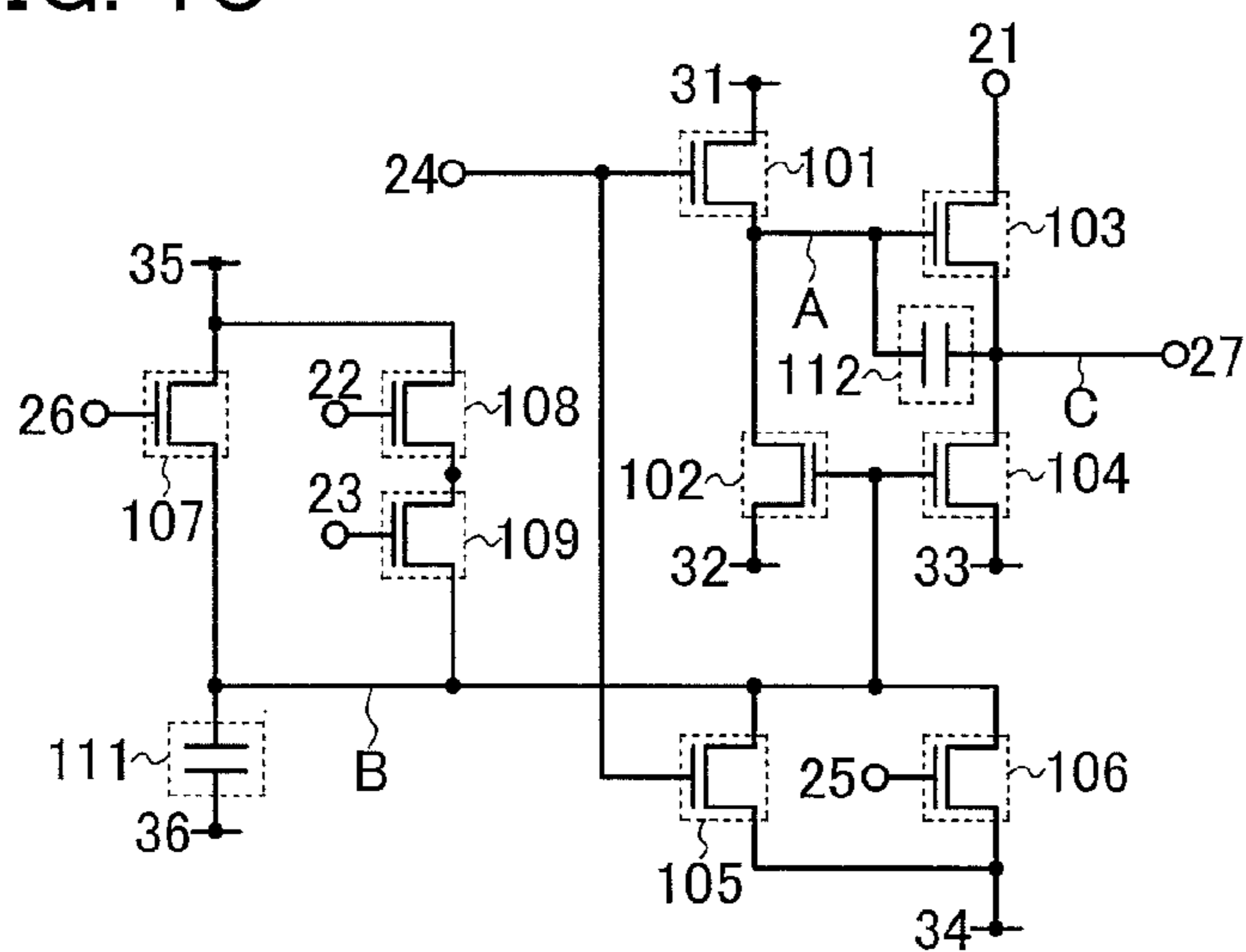
FIG. 1C
