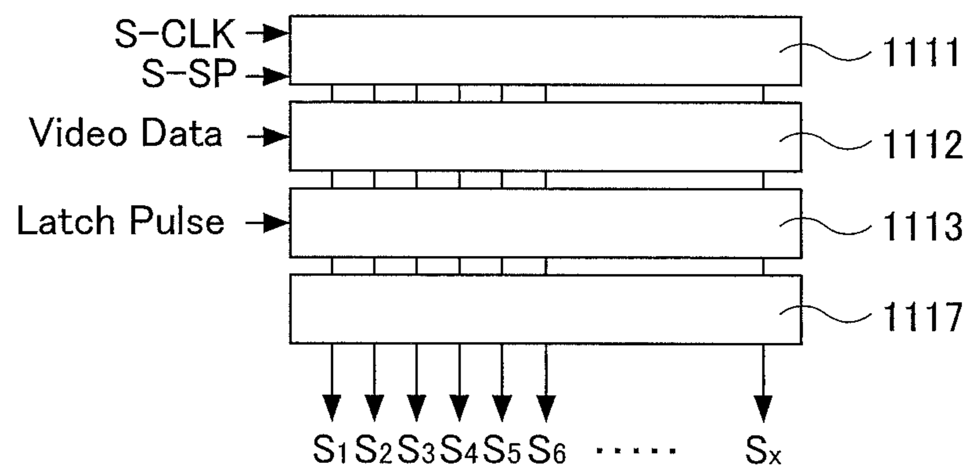
FIG. 9C
