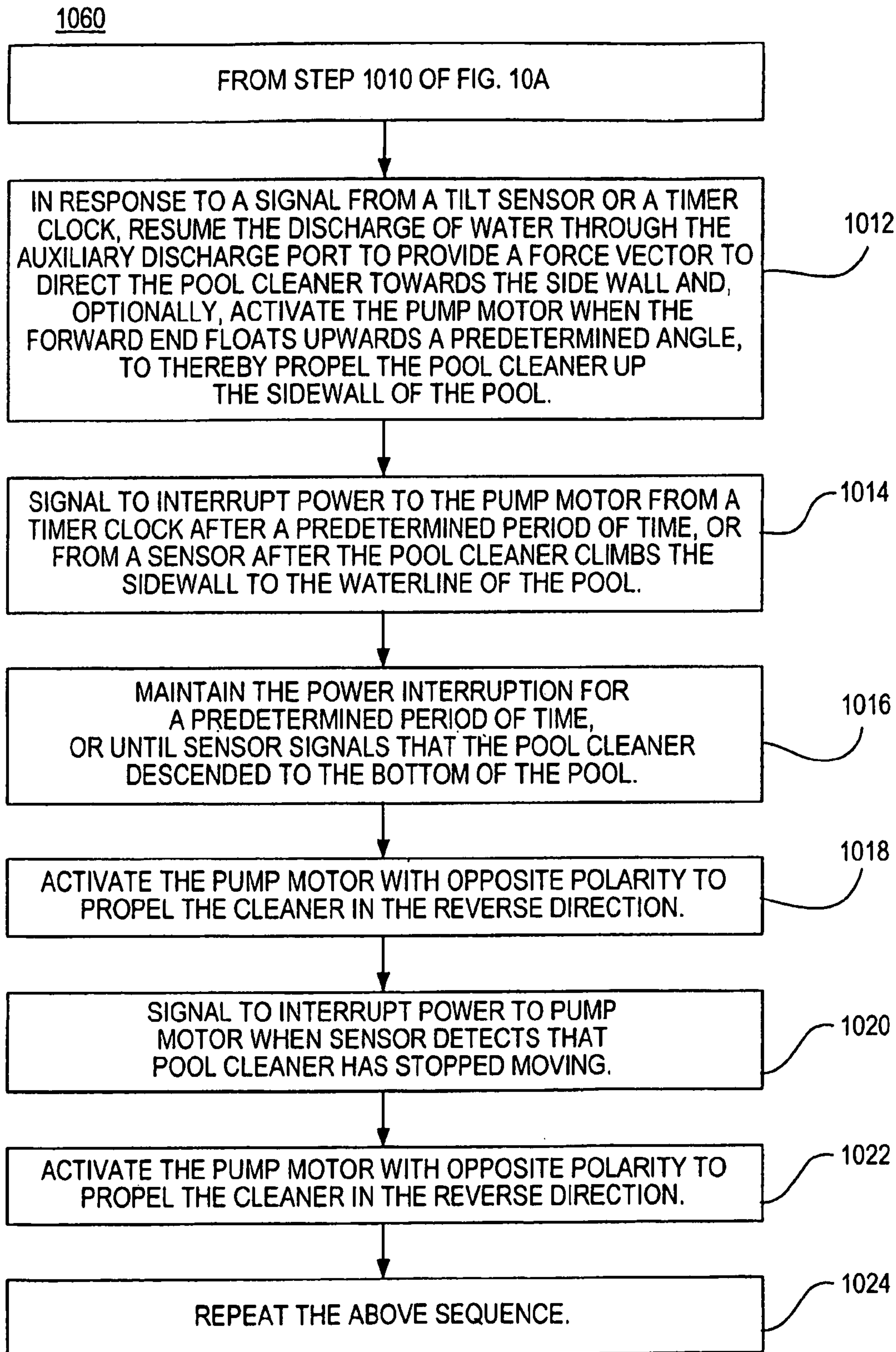
FIG. 10B
