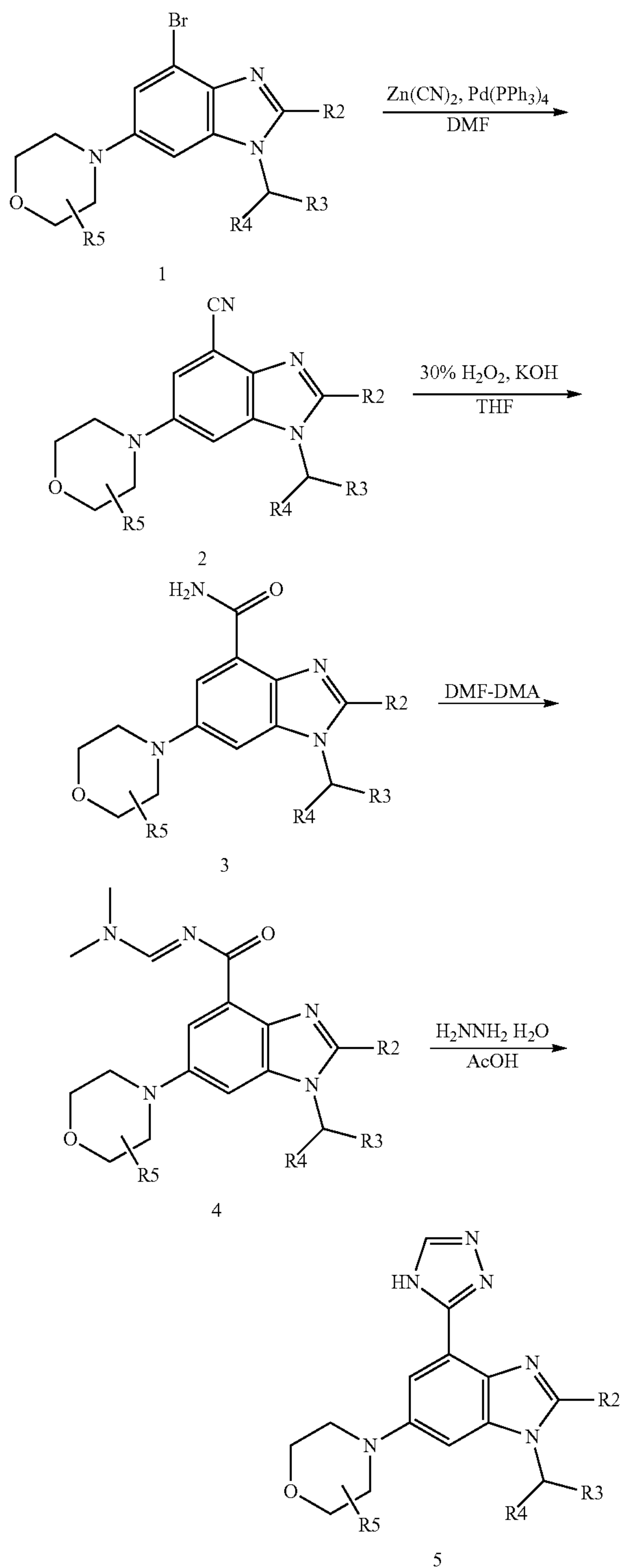
Scheme VI
