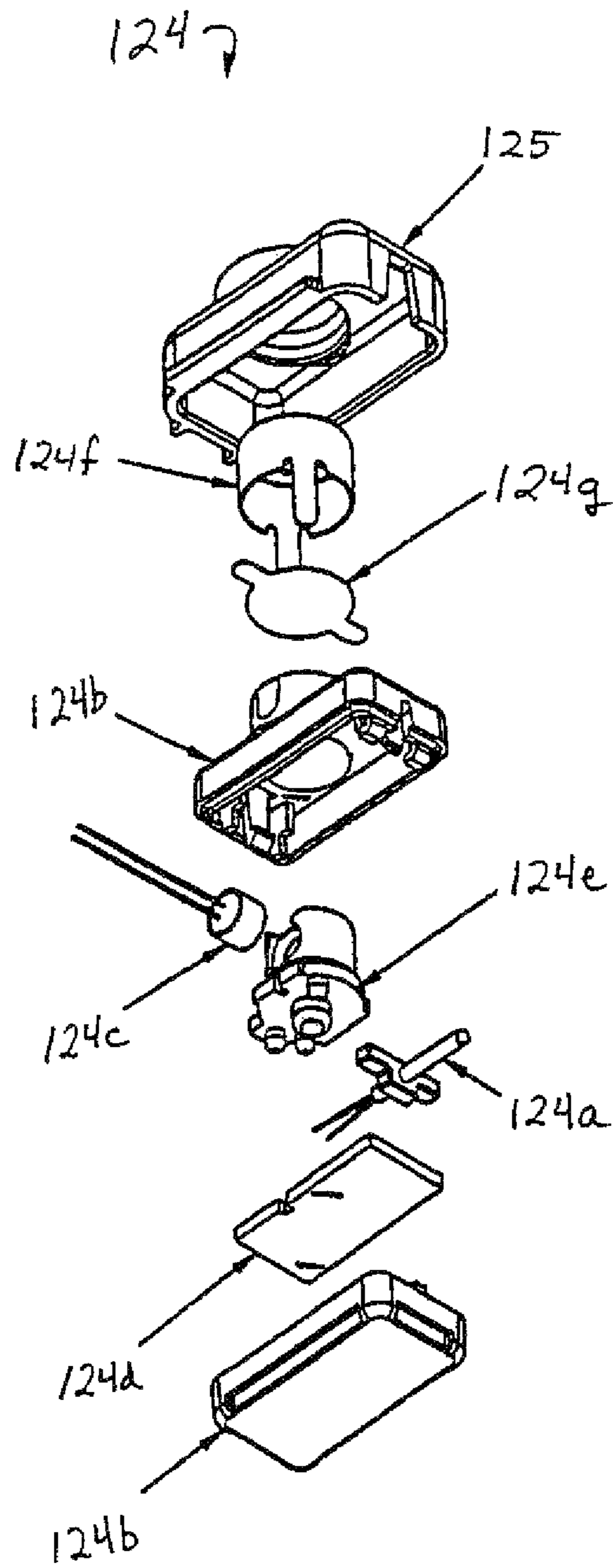
FIG. 16
