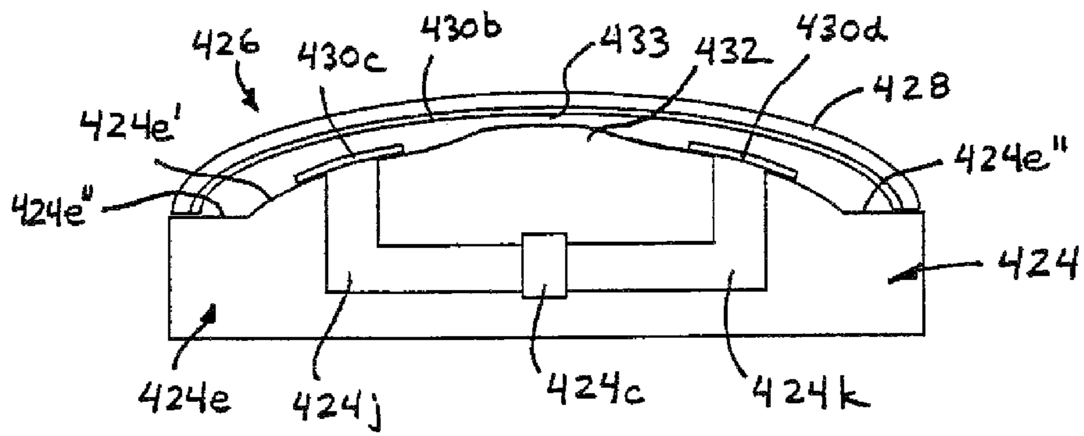
FIG. 25
