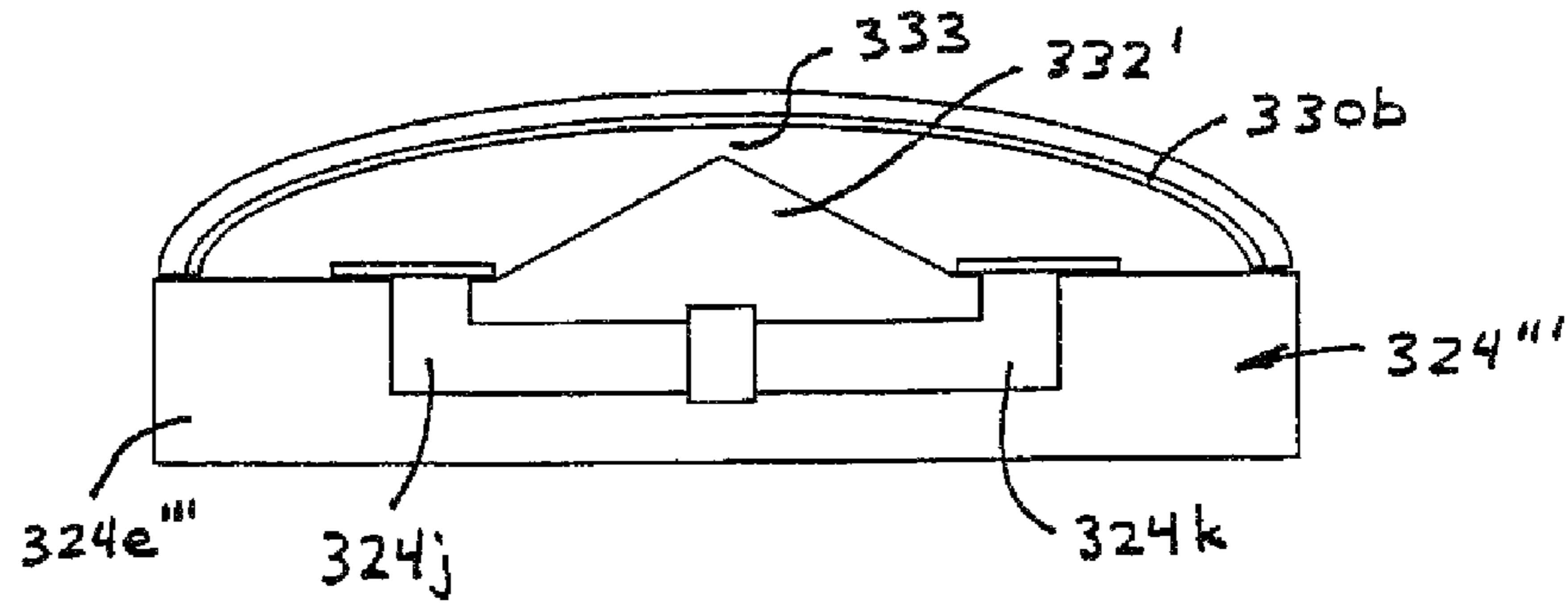
FIG. 24
