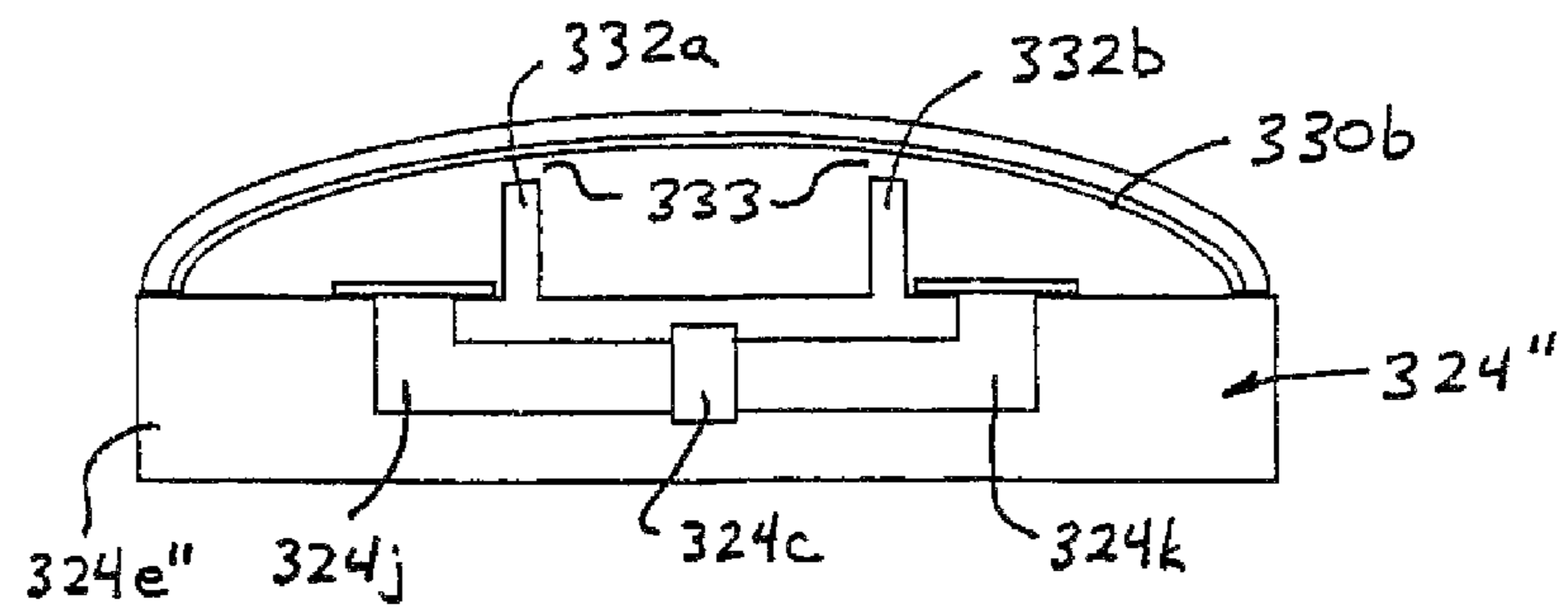
FIG. 23
