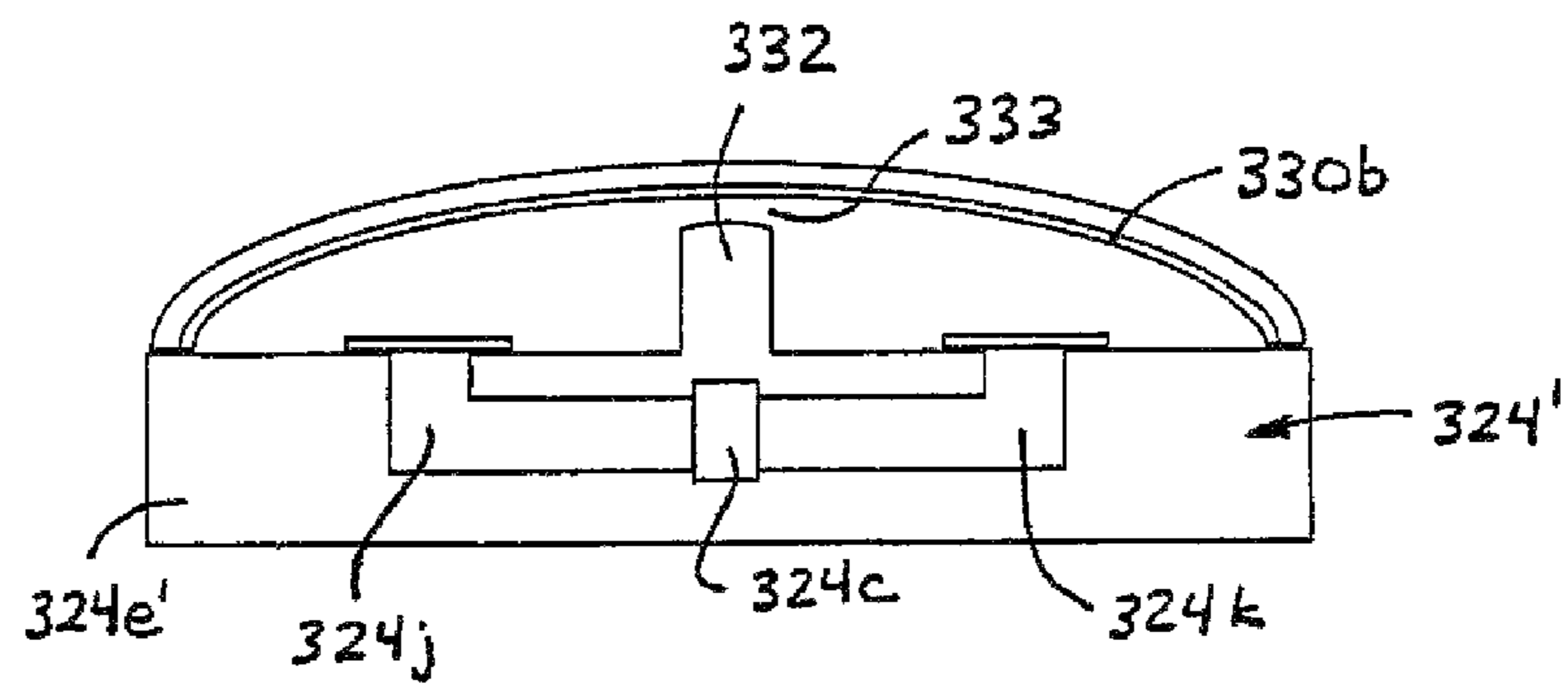
FIG. 22
