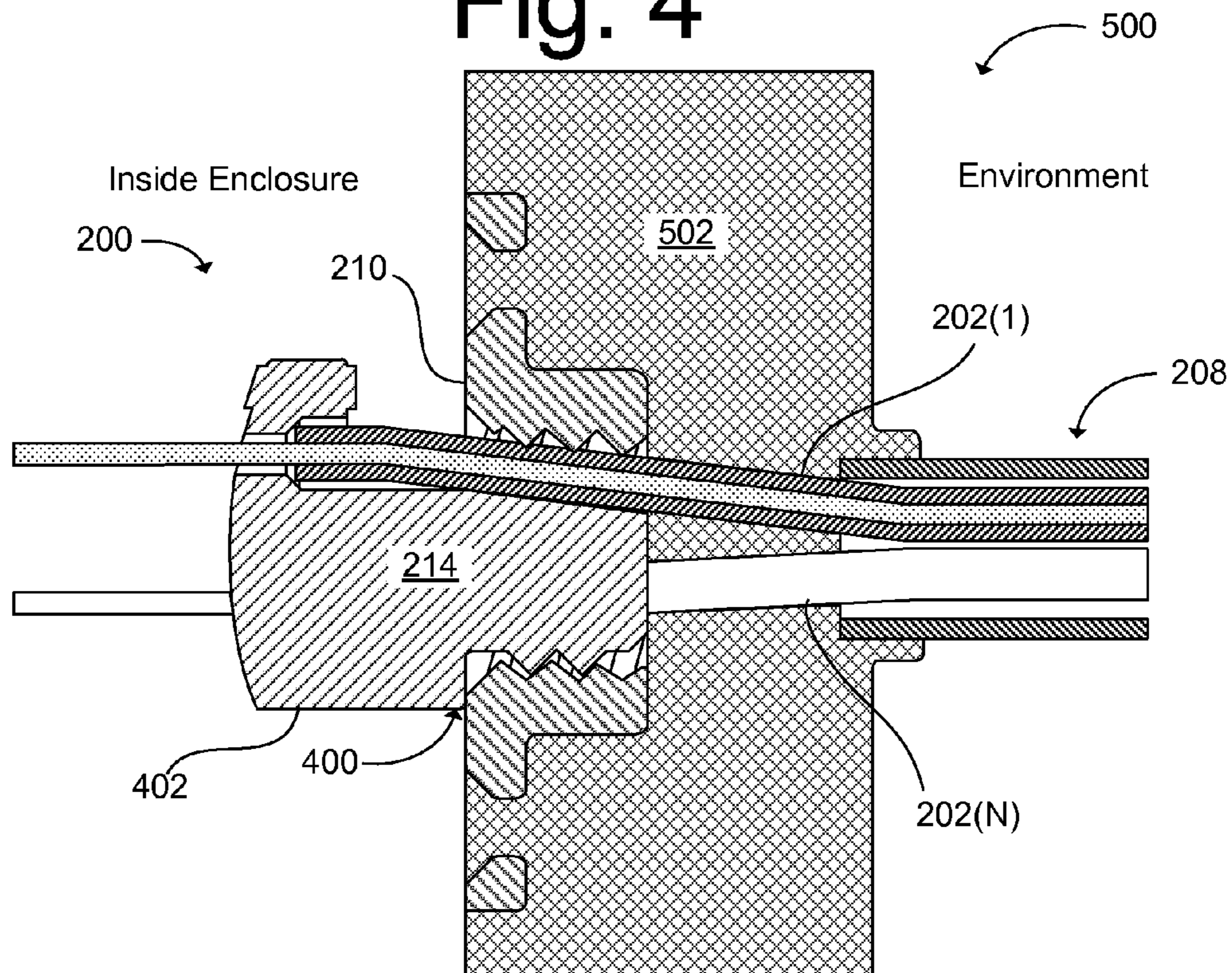
(Section A-A)
