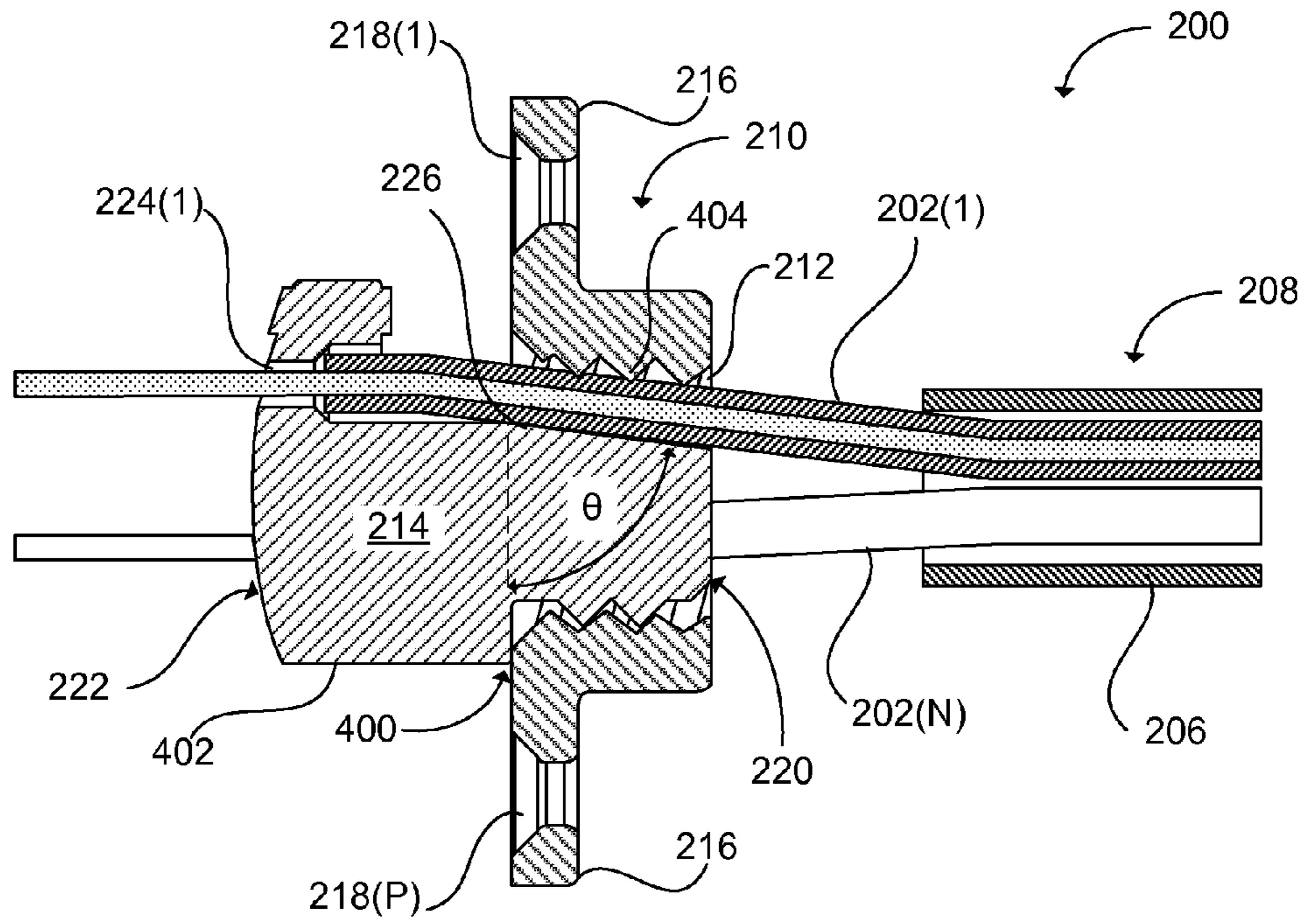
(Section A-A)
