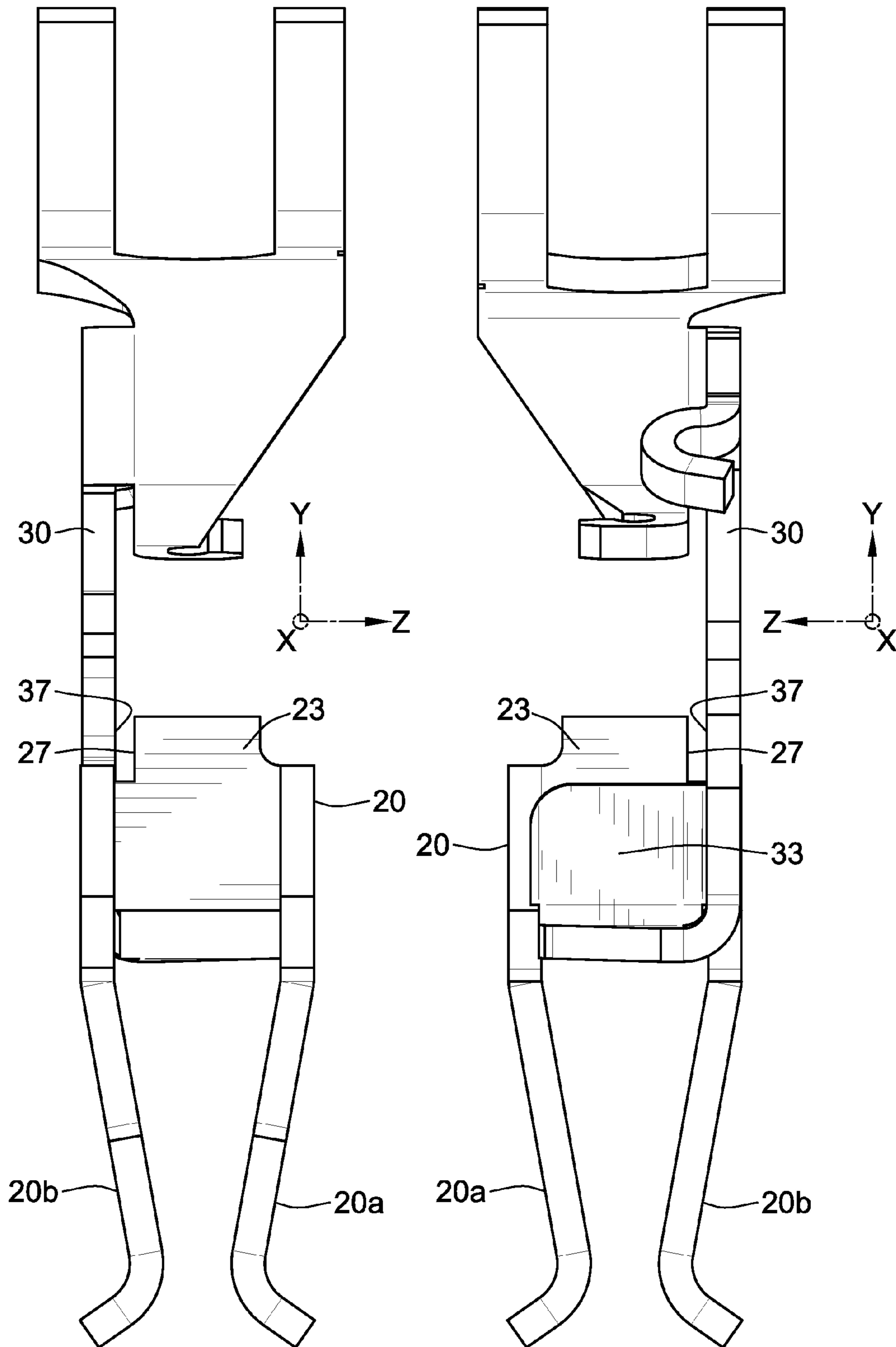
FIG. 3C
