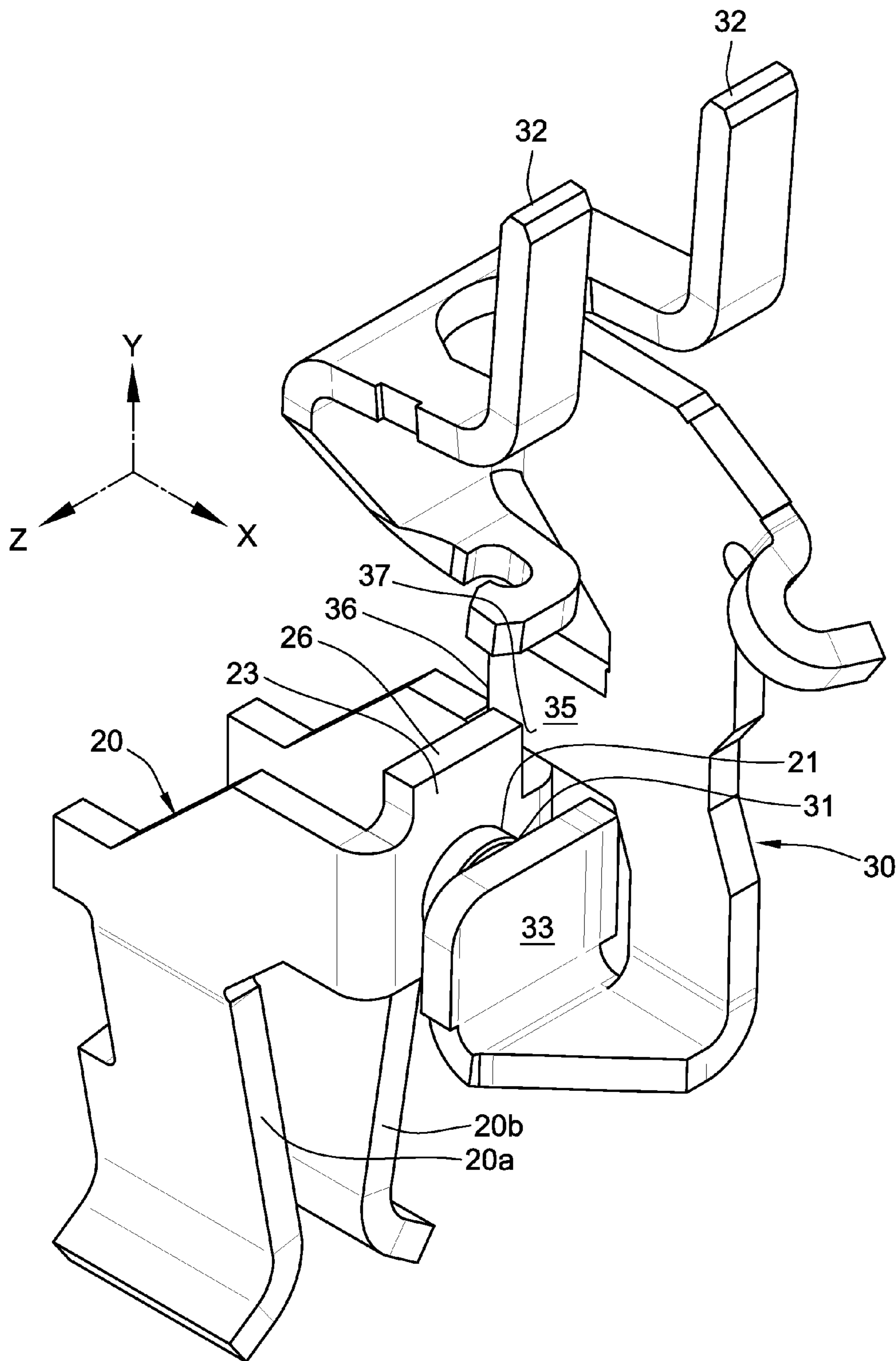
FIG. 3A
