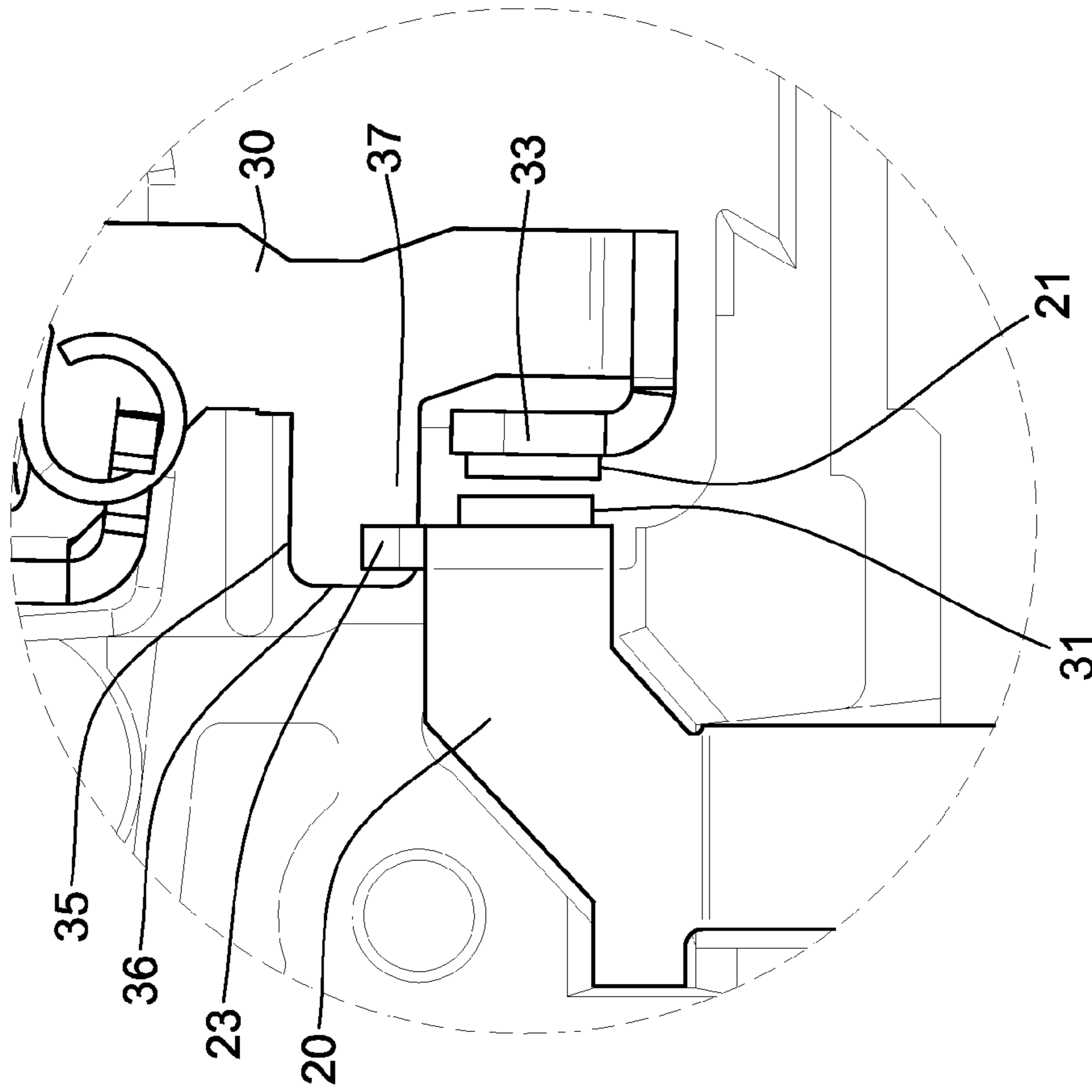
FIG. 5A
