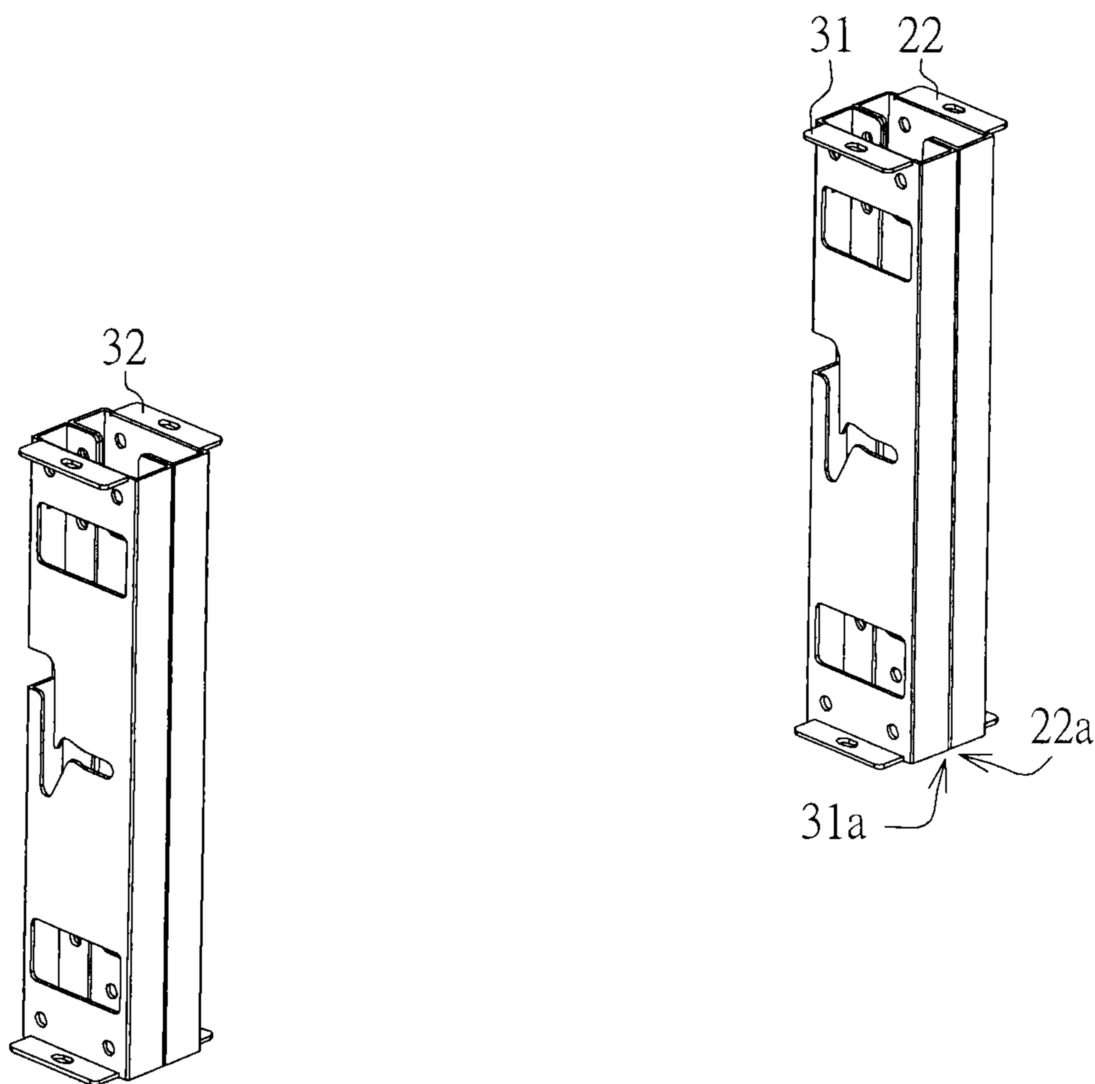
FIG. 5(a)
