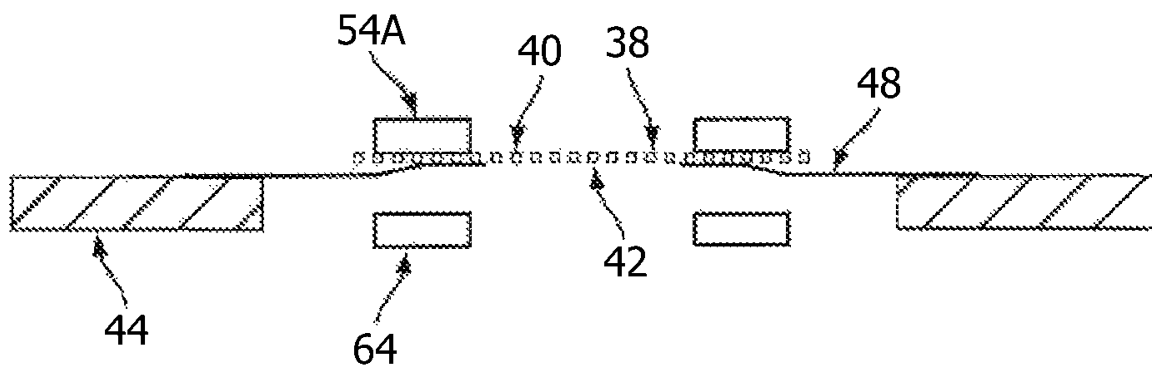
FIG. 5B
