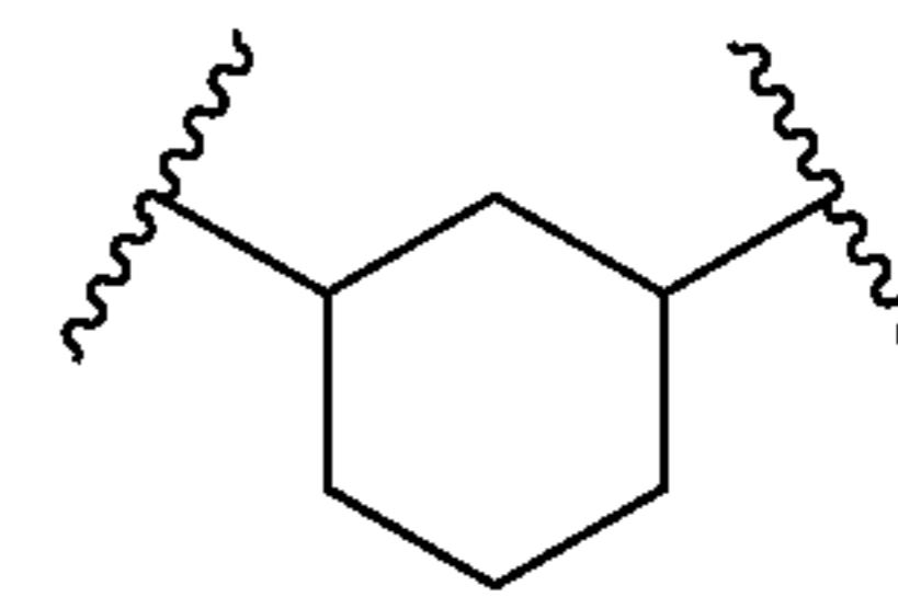
cyclohexane-1,3-di-yl
