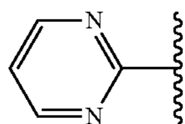
pyrimidin-2-yl
