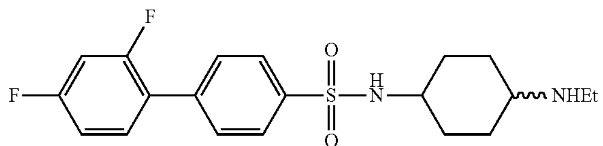
N-(4-(Ethylamino)cyclohexyl)-2',4'-difluorobiphenyl-4-sulfonamide (ABD817)
