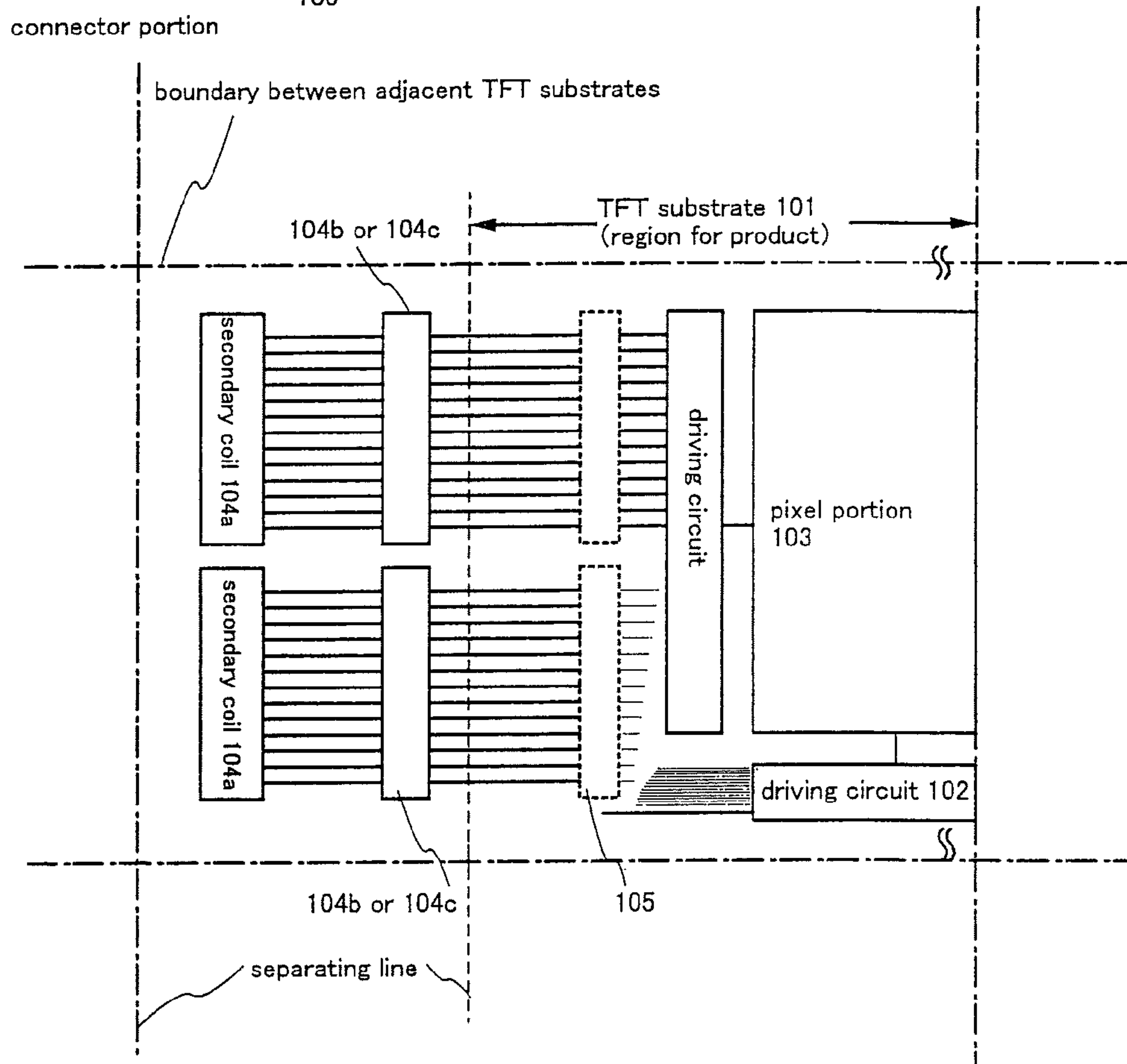
FIG. 4B array substrate
