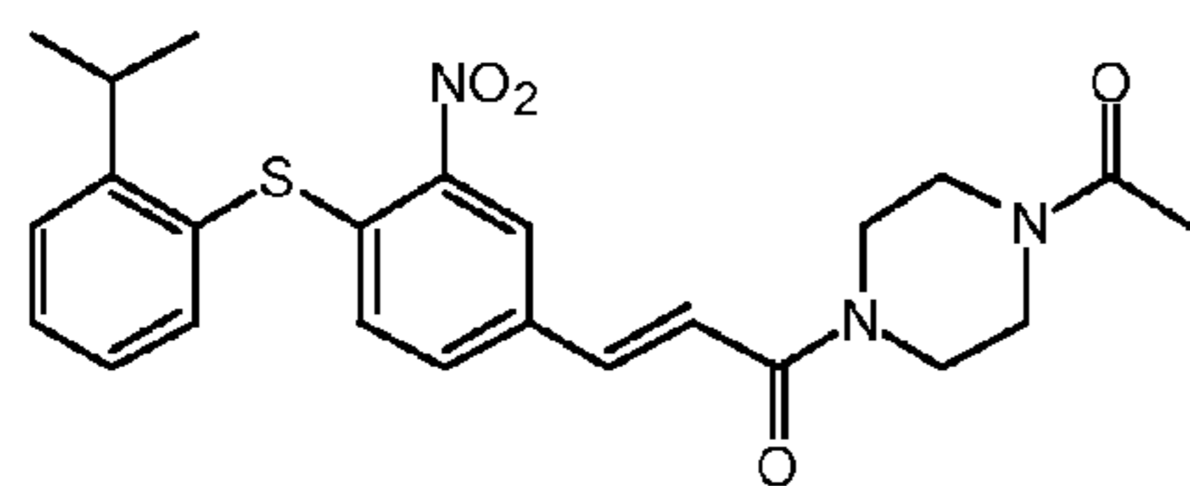
A-286982
